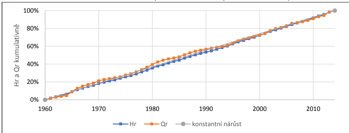
S. 78, Graf 5.13 - Jednoduché součtové řady – kumulativní řady ročních srážek a průtoků
