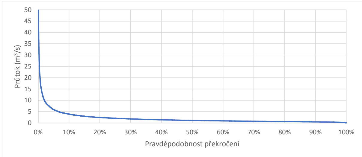
s. 76, Graf 5.11 – Čára překročení
