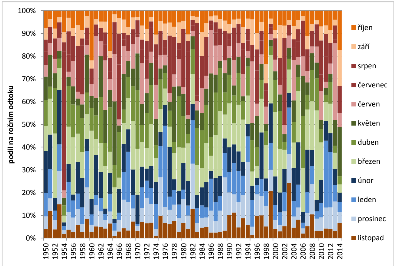
S. 72, Graf 5.5 – Vývoj podílu měsíců na ročním odtoku za období 1950-2014
