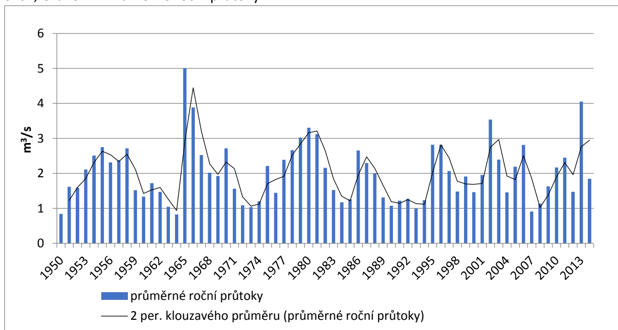
S. 67, Graf 5.1 – Průměrné roční průtoky
