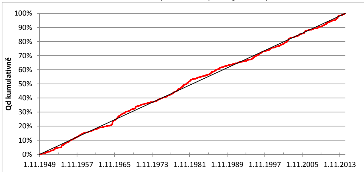
S 77, Graf 5.12 - Kumulativní řada denních průtoků za hydrologické roky 1950–2014
