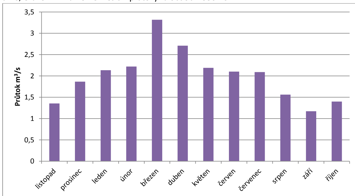
s. 70, Graf 5.2 – Průměrné měsíční průtoky za období 1950-2014
