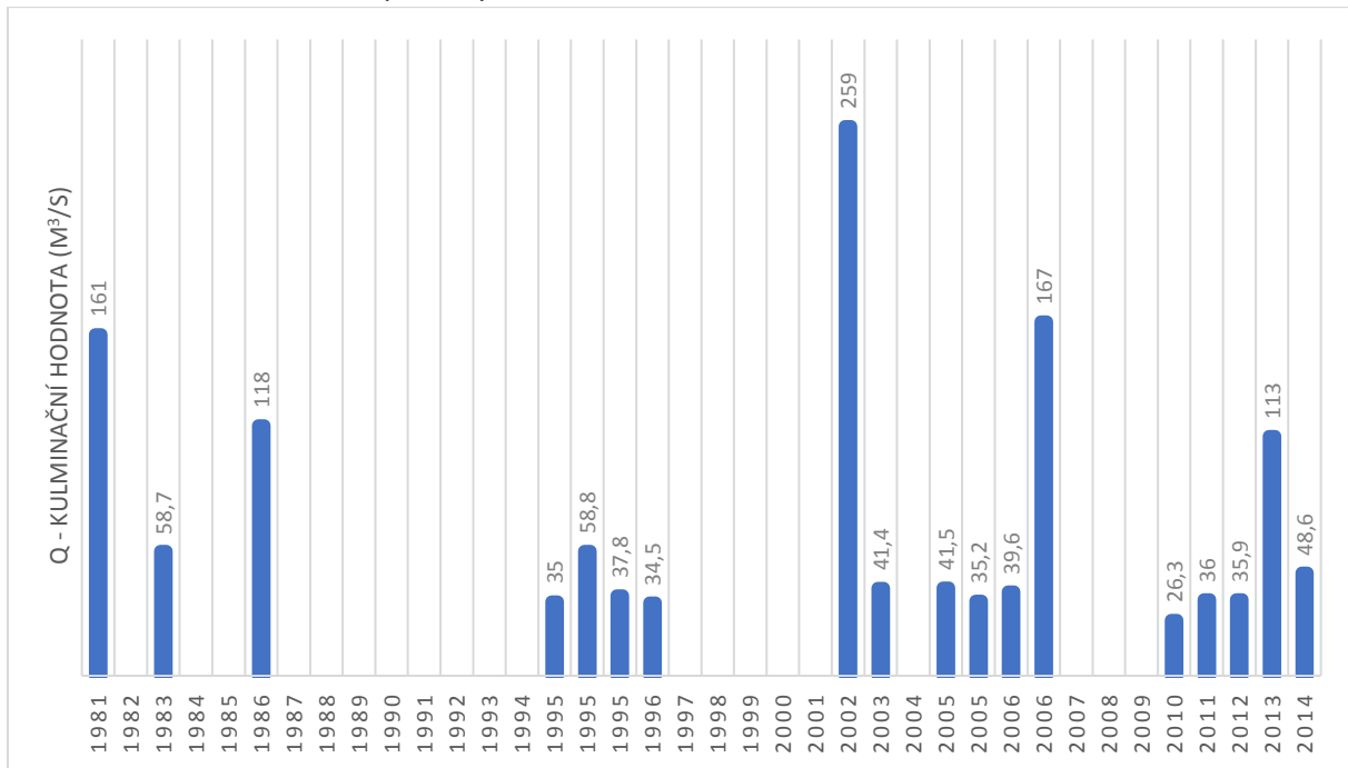
s. 87, Graf 5.20 Povodňové průtoky na Klabavě v období 1981-2014
