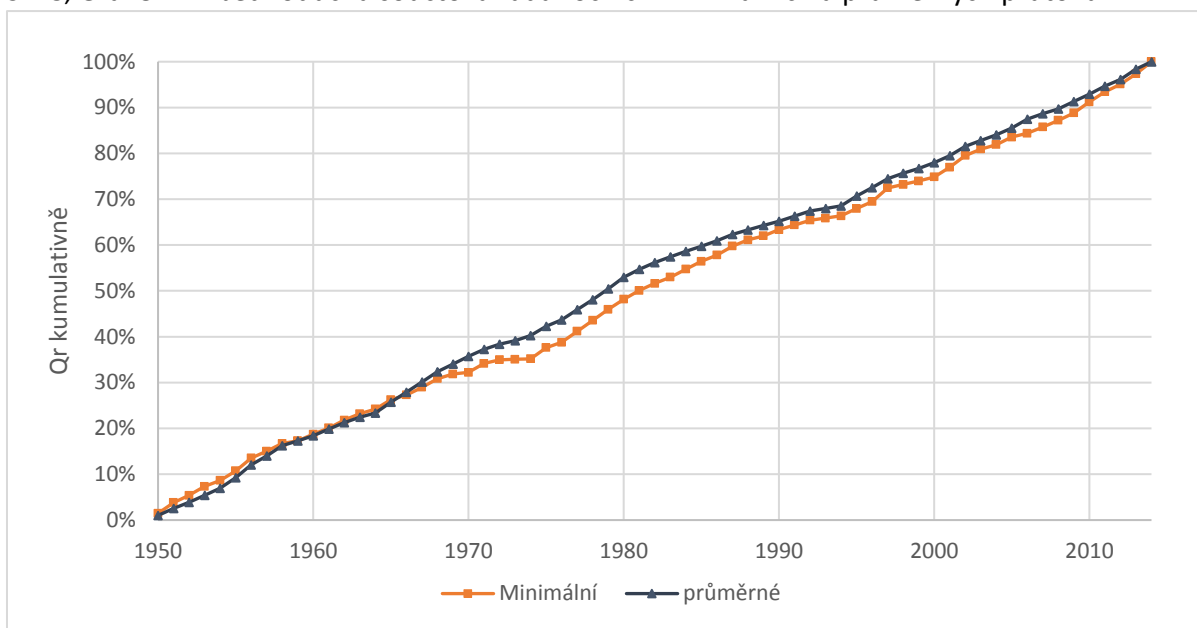
S. 78, Graf 5.14 – Jednoduchá součtová řada ročních minimálních a průměrných průtoků
