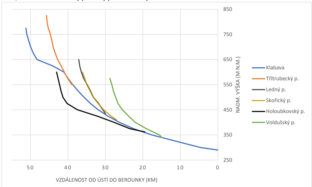
S. 63, Graf 4.8 – Rozvinutý podélný profil Klabavy
