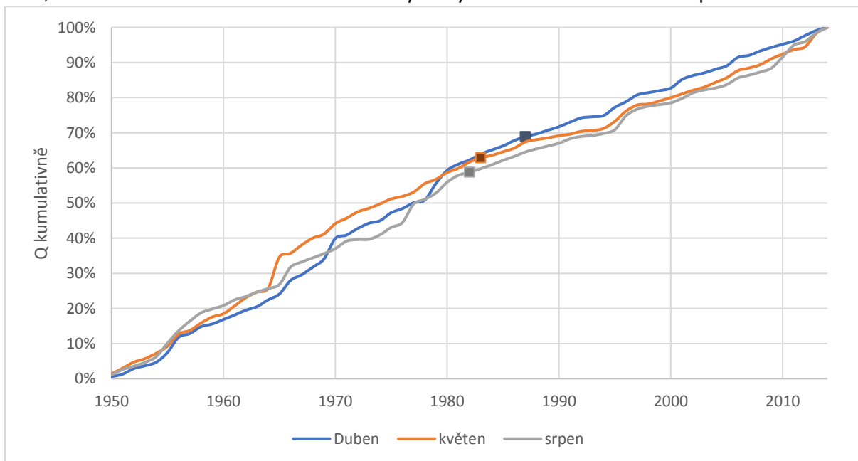
s. 81, Graf 5.15 – Jednoduchá součtová čára vybraných minimálních měsíčních průtoků
