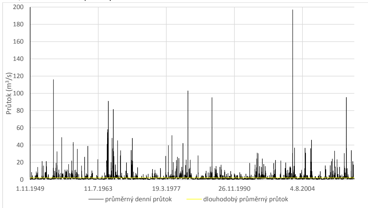
s. 74, Graf 5.7 – Denní průtoky za období 1950-2014
