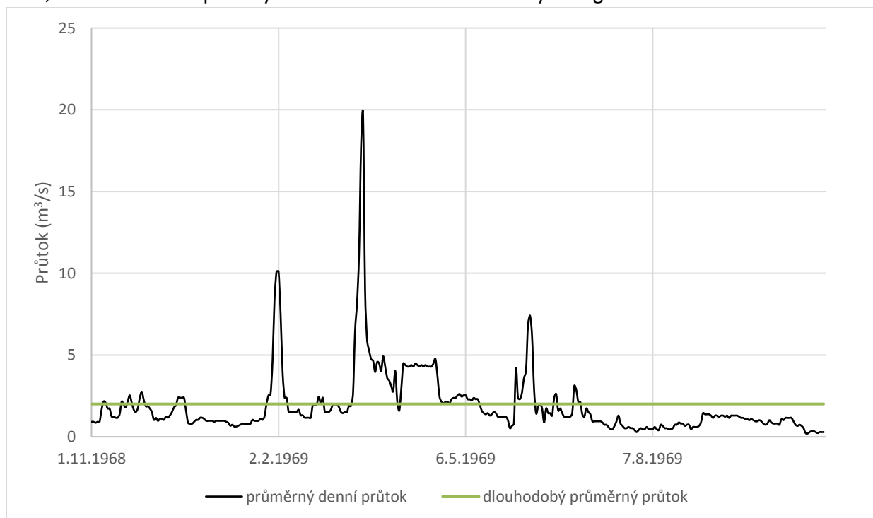
s. 74, Graf 5.8 – Denní průtoky v mimořádně málo vodném hydrologickém roce 1964
