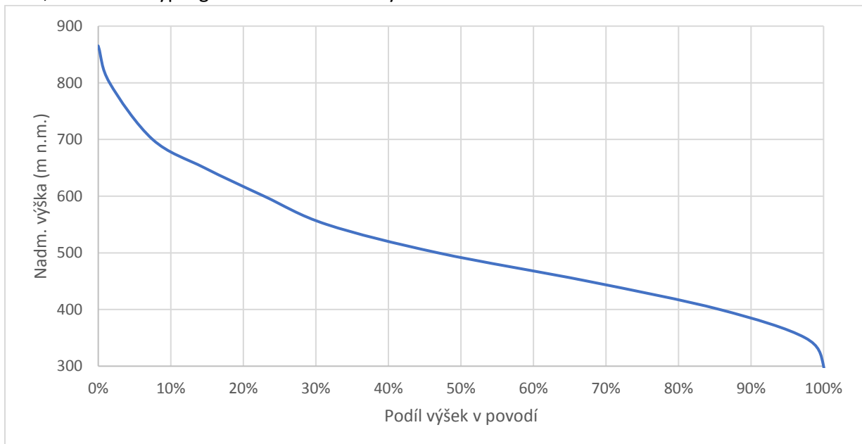
s. 63, Graf 4.9 – Hypsografická křivka Klabavy
