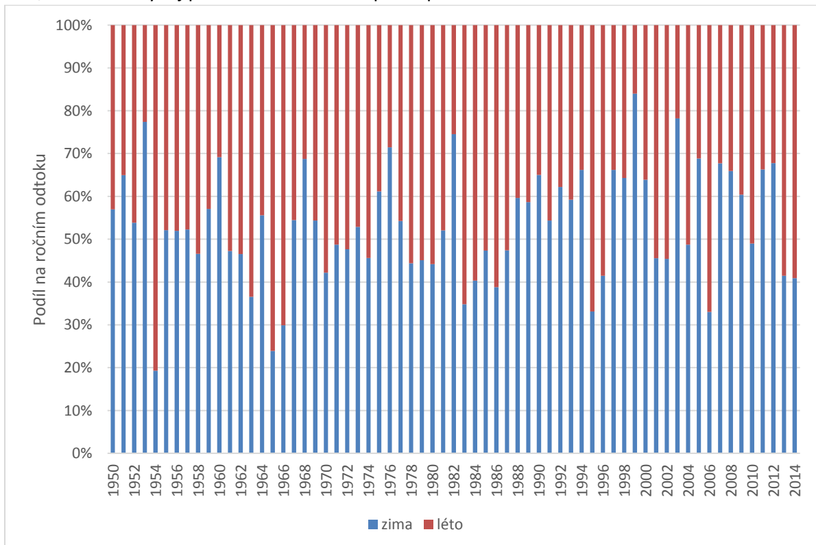
s.73, Graf 5.6 – Vývoj podílu chladného a teplého půlroku na ročním odtoku
