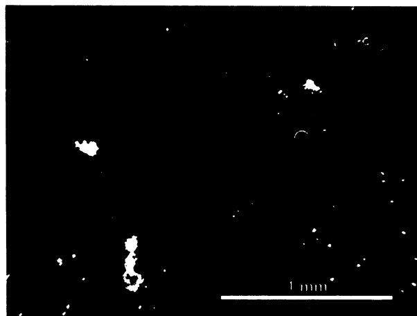
Obr. S.2.7. Výbrus č. 2b – CL: transversální průřez vzdušným kořínkem podlouhlého tvaru: buňky sklerenchymatické pochvy (červeně), chalcedonové struktury (modrofialově), dvě praskliny při okrajích vyplněny křemennou hmotou s jasně modrou CL (světle modrá uvnitř je CL podložního skla). Žlutá svítivá zrnka jsou zbytky diamantového leštidla.
