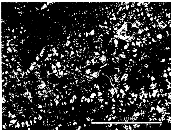
Obr. S.13.10. Výbrus č. 13 – PM: mikrokrytalický křemen (šedý), chalcedon (oranžovohnědý) a makrokrytalický křemen (vysoké interferenční barvy uprostřed snímku) v základní \text{SiO}_2 hmotě výbrusu.
