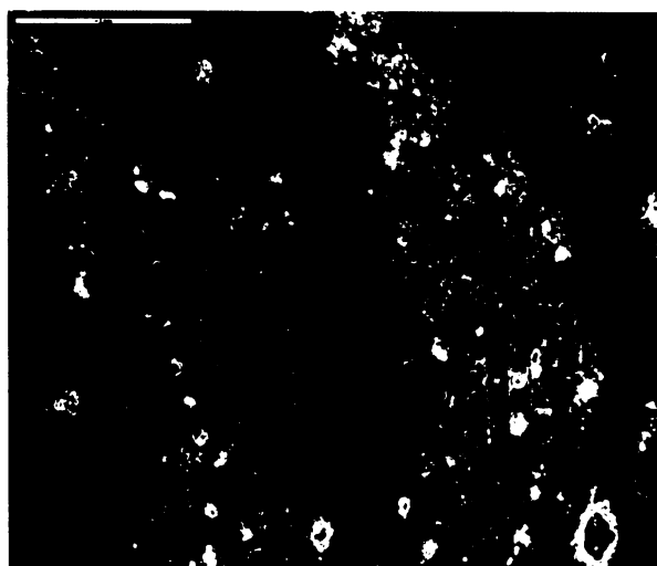
Obr. S.11.12. Výbrus č. 11 – SEM/EDX: zobrazení povrchu detektorem SE, na snímku vyniká zejména morfologie trhlín ve výbrusu, která je podobná v celém vzorku. Měřítko 1 mm; transverzální řez.
