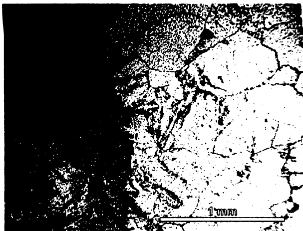
Obr. S.18.14. Výbrus č. 18 – OM: rozhraní zachovaného pletiva vnějšího sekundárního xylému přesličky (na snímku vlevo) a hypidiomorfních krystalů kalcitu (vpravo), obě vrstvy mají poměrně jasnou hranici; transverzální řez.
