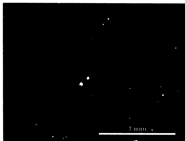
Obr. S.6.12. Výbrus č. 6b – CL: popis snímku jako na obr. vlevo, popis CL barev je uveden v textu. Všimněme si dlouhé tenké trhliny podél dřevního paprsku, která vyzářuje jasně modrou CL, hákovitě se uhybá doprava, a to v zóně dřevních buněk, které byly postiženy kompakcí a makroskopicky se na průřezu jeví jako „falešný letokruh“. Žlutá svítivá zrnka jsou zbytky diamantového leštidla.
