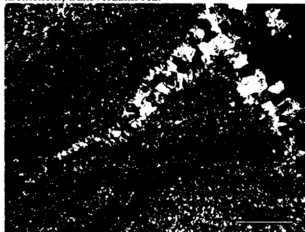
Obr. S.16.8. Výbrus č. 16 - PM: popis snímku jako na obr. vlevo, dobře rozeznatelné krystaly makrokrytalického mozaikovitého křemene, železitý pigment zůstává v polarizovaném světle hnědý; transversální řez.
