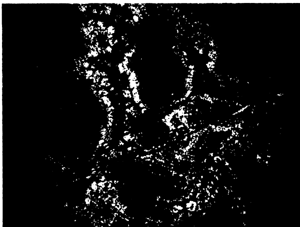
Obr. S.17.5. Výbrus č. 17 – OM: sekundární xylém dadoxylonového typu, silně porušený rekrytalizací. Pigmentované dřevo je roztrháno na samostatné segmenty, které jsou často ukloněny v blízkosti zlomových ploch až o desítky stupňů; transverzální řez.
