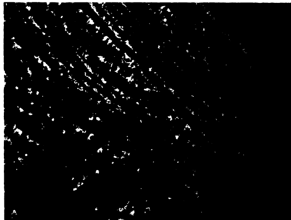
Obr. S.13.5. Výbrus č. 13 – PM: popis snímku jako na obr. vlevo. Základní hmota výlitku je tvořena krystaly mikrokrytalického křemene, uspořádanými do tenkých pásků, místy pigmentovaných oxidy železa a chalcedonem. Ve větších prostorách a dutinách jsou krystaly makrokrytalického křemene s vysokými interferenčními barvami.
