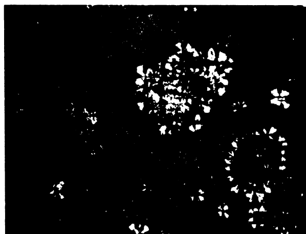
Obr. S.4.5. Výbrus č. 4a - PM: popis snímku jako na obr. vlevo. Intersticiální tkáň i sklerenchymatické pochvy kořínků jsou mineralizovány mikrokrystalickým křemenem (šedý a nahnědlý), chalcedon (oranžovohnědý) často nahrazuje jak cévní svazek, tak i původní parenchym či aerenchym uvnitř kořínku.
