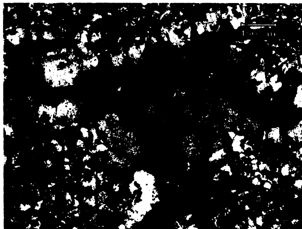
Obr. S.17.8. Výbrus č. 17 – PM: popis snímku jako na obr. vlevo. Rekrystalizovanou strukturu lemují krystaly makrokystalického křemene, ve zkřížených nikolech s vysokými interferenčními barvami.
