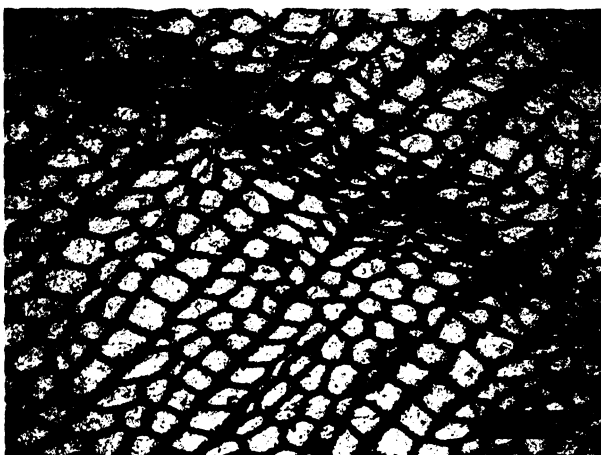
Obr. S.6.7. Výbrus č. 6b – OM: transverzální průřez sekundárním xylémem rodu Arthropitys . Řady tracheid i dlouhých paprsků vedou na snímku diagonálně. Po levé straně je doprovází tenká světlá trhlina. Buňky ve zdánlivé přírůstkové zóně zde vypadají velmi smáčknuté a spíše podporují hypotézu kompakce vzorku.
