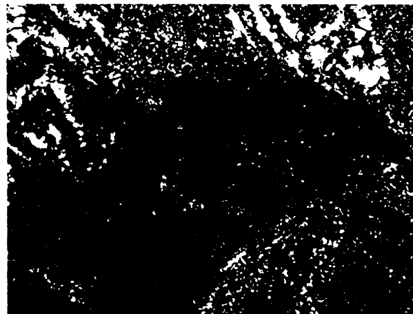
Obr. S.13.7. Výbrus č. 13 – PM: oxidy Fe (hnědé) jsou obklopeny základní hmotou z šedého mikrokrytalického křemene. Místy vykrytalizoval i makrokrytalický křemen (širší světlé pásky v horní polovině snímku).
