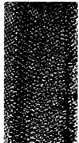
Obr D.3. Vpravo: radiální řez tracheidou sekundárního xylému se střídajícími se kruhovitými tečkami na radiální stěně. Svrchní pennsylvan; upraveno ze Stewarta & Rothwella (1993).
