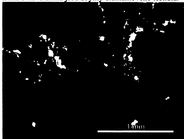
Obr. S.9.13. Výbrus č. 9 – CL: popis snímku jako u obr. S.9.11; odlišné místo ve výbrusu.
