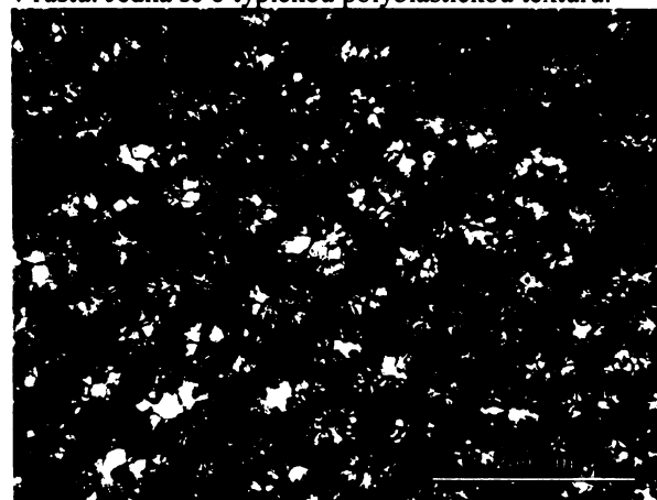
Obr. S.6.10. Výbrus č. 6b – PM: sekundární xylém rodu Arthropitys jako na obr. S.6.8 při větším zvětšení.
