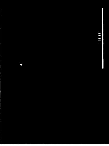
Obr. S.4.14. Výbrus č. 4b - CL - bod 1: mikrokrystalický křemen má červenou CL, chalcidon modrofialovou a makrokrystalický křemen uvnitř zachovaných parenchymatických buněk hnědofialovou CL. Tmavé karminové skvrny, rozptýlené v základní hmotě, jsou oxidy Fe.
