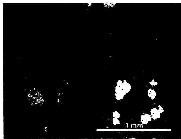
Obr. S.18.9. Výbrus č. 18 – CL: popis snímku jako na obr. vlevo. V detritickém materiálu jsou patrné K-živce (modrá CL) a plagioklasy (zelená CL), v karbonátových lalokovitých útvarech se objevuje zonalita (světlé oranžové skvrny); transverzální řez.
