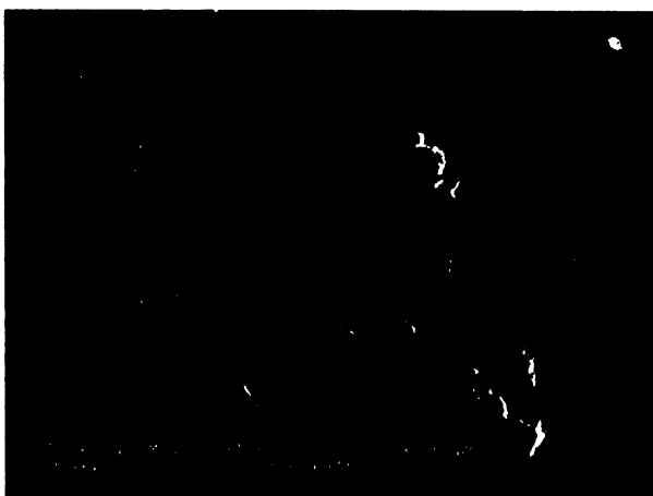
Obr. S.5.26. Výbrus č. 5b – SEM/EDX - bod 2.1: zobrazení chemického kontrastu slidového zrna (biotit, mírně vlevo od středu) s dobře patrnou štěpností detektorem RBS.
