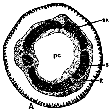
Obr. E.2. Stavba kordaitového dřeva. A - Příčný průřez mladou větví Cordaitoxylon GR.'EURY: dřeňová dutina (pc), sekundární xylém (sx), primární cévní svazek (s), listová stopa (lt); pennsylvan. B - Radiální řez kmenem kordaitů od centrální dřeně směrem ke kůře (zleva doprava): šroubovitě a kruhovitě ztlustlý protoxylém, schodovitě ztlustlý a přechodně dvůrkatý metaxylém a tečkované tracheidy sekundárního xylému s hustě sestavenými dvůrky ve více řadách (tzv. araukaroidní tečkování); karbon; upraveno podle Stewarta & Rothwella (1993).
