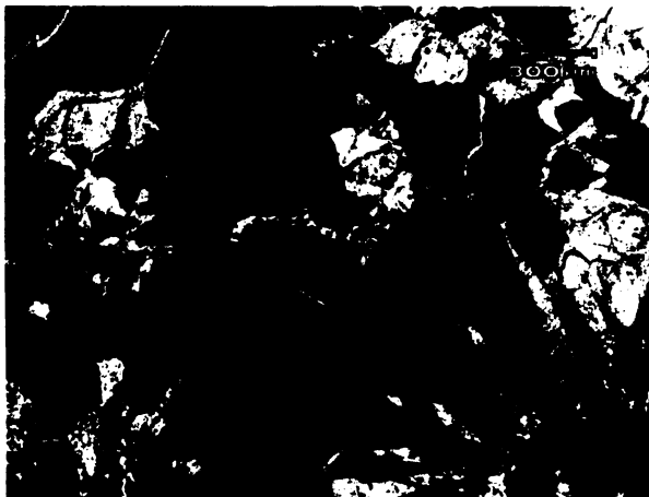
Obr. S.9.2. Výbrus č. 9 (vlevo): transverzální řez dřevem rodu Dadoxylon ENDL.: sekundární xylém se téměř nedochoval, celý výbrus je silně rekrystalizovaný krystaly křemene o různé velikosti a tvaru. Celý vzorek je roztrhán velkým množstvím prasklin, některé z nich jsou tmavě hnědé až rezavě lemované. Velikost podložního skla 5 x 2,7 cm.
