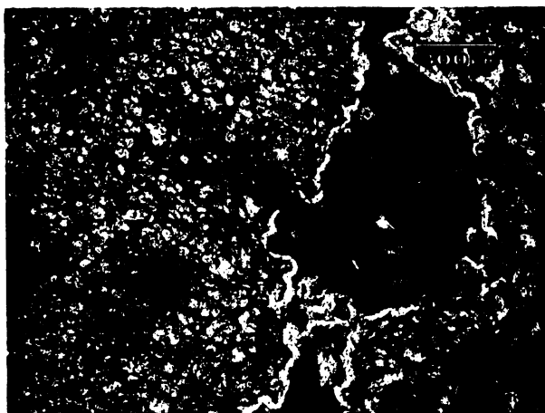
Obr. S.8.4. Výbrus č. 8 – OM: centrální dřeví složená z oblých parenchymatických buněk, v dřevěné dutině se nacházejí výrazné sférolity chalcedonu, rostoucí symetricky z obou okrajů dutiny proti sobě; transverzální řez.
