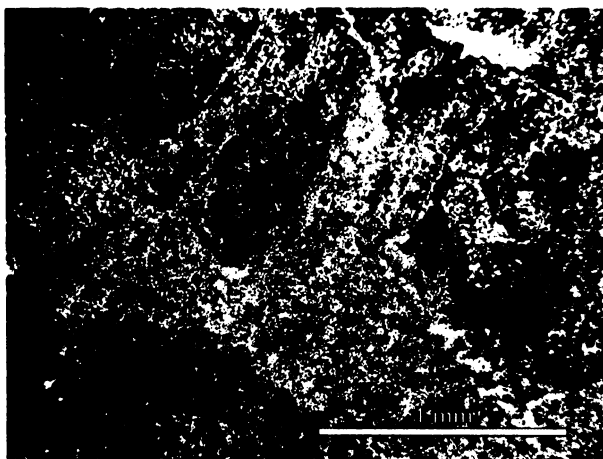
Obr. S.7.13. Výbrus č. 7 – OM – oblast 4 (CL); výrazně narušená oblast začínajícího sekundárního xylému v dolní části výbrusu (obr. S.7.3), opticky vypadá jako silně postižená rekrystalizaci; transversální řez.
