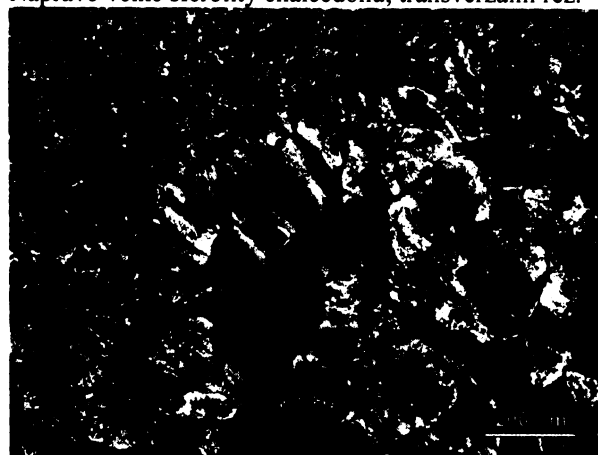
Obr. S.7.12. Výbrus č. 7 – PM: sekundární xylém z tmavé hladké zóny vnějšího okraje, tracheidy a paprsky tvoří mikrokrytalický křemen, vnitřky některých buněk vyplňuje oranžovohnědý chalcedon. Část pletiva byla silně rekrystalizována makrokrytalickým křemenem (vysoké interferenční barvy).
