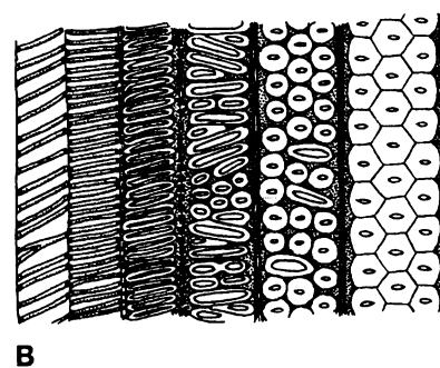
Obr. E.2. Stavba kordaitového dřeva. A - Příčný průřez mladou větví Cordaitoxylon GR.'EURY: dřeňová dutina (pc), sekundární xylém (sx), primární cévní svazek (s), listová stopa (lt); pennsylvan. B - Radiální řez kmenem kordaitů od centrální dřeně směrem ke kůře (zleva doprava): šroubovitě a kruhovitě ztlustlý protoxylém, schodovitě ztlustlý a přechodně dvůrkatý metaxylém a tečkované tracheidy sekundárního xylému s hustě sestavenými dvůrky ve více řadách (tzv. araukaroidní tečkování); karbon; upraveno podle Stewarta & Rothwella (1993).
