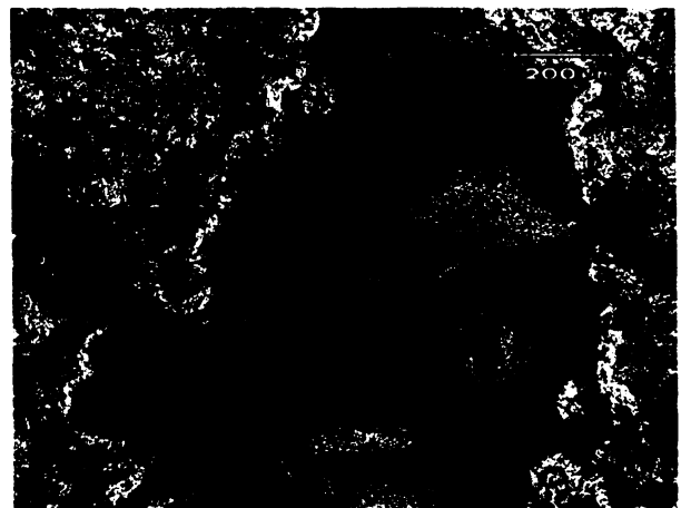
Obr. S.8.5. Výbrus č. 8 – PM: sférolity chalcedonu s typickým zhášením po paprscích, uspořádané proti sobě v centrální dřeví, lemované bílou žilkou mikrokrytalického křemenem; transverzální řez.
