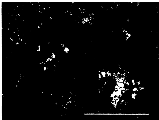
Obr. S.7.19. Výbrus č. 7 – PM – oblast 2 (CL): Sférolity chalcedonu (oranžovohnědé) ze světlé „očkovité“ části sekundárního xylému. Jejich středy jsou vyplněny makrokrytalickým křemenem čiré barvy, okolní tkáň je značně rozrušena; transverzální řez.
