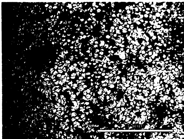
Obr. S.8.12. Výbrus č. 8 – OM: centrální dřeňová dutina se zachovanou strukturou některých eliptických parenchymatických buněk, tvořenou mikrokrytalickým křemenem a sférolity chalcedonu.
