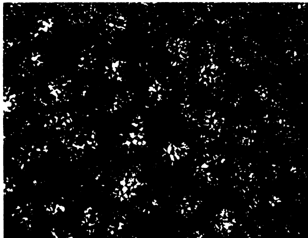
Obr. 29. Výbrus č. 6 – PM: buněčné stěny tracheid a paprsků jsou permineralizovány mikrokrytalickým křemenem, jejich vnitřky drobným a hrubším makrokrytalickým křemenem. Struktura pletiva je mnohem hůře rozlišitelná než v OM i CL. Transverzální řez dřevem rodu Arthropytis .
