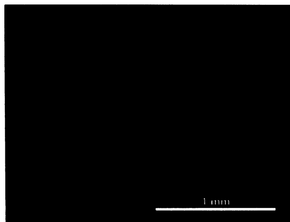
Obr. S.17.10. Výbrus č. 17 – CL: popis snímku jako na obr. vlevo. Červená CL mikrokrystalického křemene, se prolíná s modrofialovou CL a dává celému snímku červenofialový nádech, tmavě karmínové skvrny jsou oxidy železa; transverzální řez.
