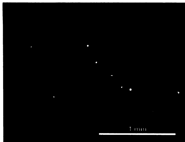
Obr. S.2.5. Výbrus č. 2b – CL: transversální průřez vzdušným kořínkem, buňky sklerenchymatické pochvy (červeně), chalcedonové struktury (modrofialově), prasklinu uprostřed lemují tenká modrá žilka, která vbíhá do sklerenchymu. Žlutá svítivá zrnka jsou zbytky diamantového leštidla.
