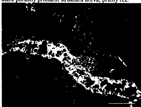
Obr. S.7.8. Výbrus č. 7 – PM: popis snímku jako na obr. vlevo. Prasklinu vyplňuje makrokrytalický čirý křemen, chalcedon je oranžově hnědý a typický po jednotlivých paprscích zháší ve zkřížených nikolech. Zbylou tkáň dřevních paprsků a tracheid převážně vyplňuje mikrokrytalický křemen (šedý). Některé vnitřky tracheid jsou vyplněny xenomorfními krystalky chalcedonu; transverzální řez.
