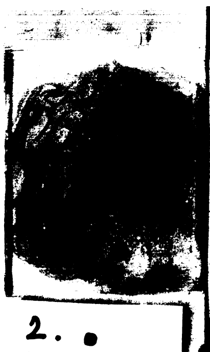
Obr. S.2.3. Výbrus č. 2a (vlevo) a 2b (vpravo): většinu výbrusu tvoří tmavě zbarvené sklerenchymatické pochvy vzdušných kořínků z vnitřního pláště, mezi nimi je ukryta sekundární (intersticiální) parenchymatická tkáň se zrní sedimentu. Vzorkem prochází velké množství prasklin. Velikost podložního skla 5 x 2,7 cm, transverzální průřez.
