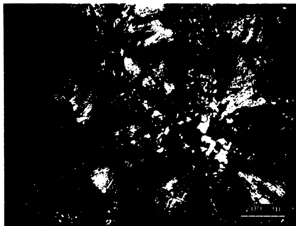
Obr. S.4.9. Výbrus č. 4b - PM: transverzální řez sférolity chalcedonu (oranžovohnědé) v oblasti parenchymatické výplně diktyostélé. V jejich středu vykristalizoval čirý makrokrytalický křemen, zatímco okolní hmota je tvořena jemným mikrokrytalickým křemenem šedé barvy.
