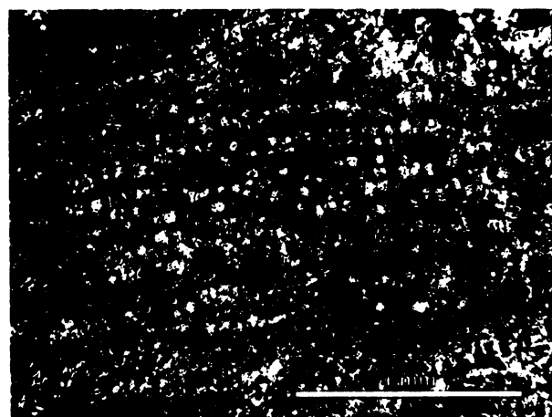
Obr. S.17.9. Výbrus č. 17 – PM: transverzální řez rekrystalizovaným sekundárním xylémem. Tracheidy a paprsky zachovaných dřevních buněk jsou mineralizovány mikrokrystalickým křemenem, v tracheidách jsou často nahloučeny oxidy Fe.
