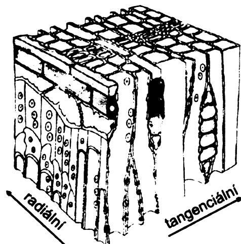
Obr. 24. Prostorový diagram pyknoxylického koniferového dřeva, šipkami je znázorněn radiální a tangenciální řez sekundárním xylémem, přičemž transverzální řez je horní plocha obrázku. Červeně jsou zvýrazněny průřezy dřevními parenchymatickými paprsky vedoucími v horizontálním směru, žlutě vybarvena jedna z mnoha vertikálně jdoucích tracheid, na jejich radiálních stěnách jsou vidět dvojtečky; upraveno z internetového zdroje č. 2.
