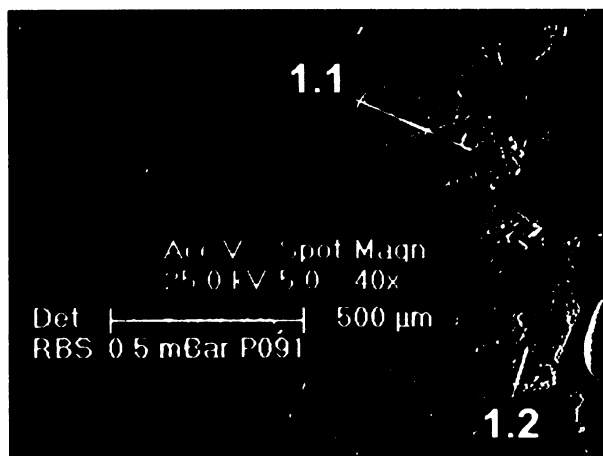
Obr. S.9.15. Výbrus č. 9 – SEM/EDX – oblast 1: zobrazení chemického kontrastu vybrané oblasti 1 ve střední části výbrusu detektorem RBS a lokalizace měřených bodů (1.1 a 1.2).
