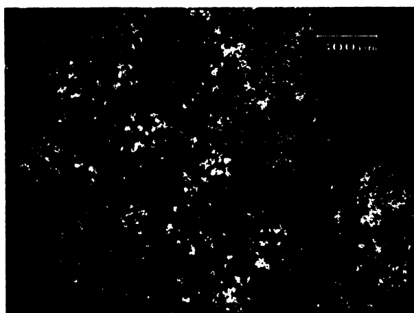
Obr. S.8.8. Výbrus č. 8 – OM: oblast sekundárního dřeva, silně rekrystalizovaná chalcedonem a makrokrystalickým křemenem, diagonálně se táhne tmavě lemovaná řada tracheid, výrazně prolomená rekrystalizací; transverzální řez.
