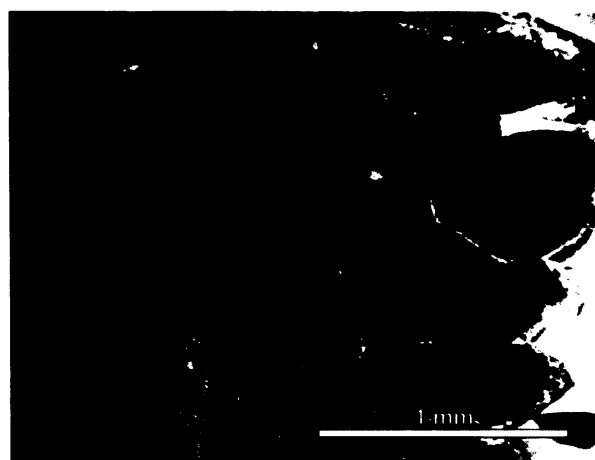
Obr. S.18.13. Výbrus č. 18 – CL: popis snímku jako na obr. vlevo. Vymezený pásek karbonátu má úplně jiný odstín oranžové barvy, což ukazuje na jeho odlišnou genezi; transverzální řez.
