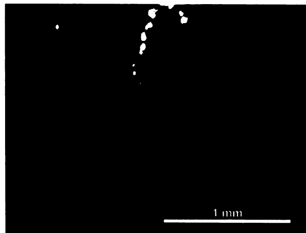
Obr. S.11.7. Výbrus č. 11 – CL: tmavě fialovou CL má hmota permineralizující zbytky sekundárního xylému, modrou CL doslova září všechny objekty obklopující dutiny a praskliny. Jasně svítivá drobná zrnka jsou nahromaděny v prasklině, jedná se o zbytky diamantového leštidla; transversální řez.
