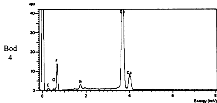
Obr. S.19.9. Vzorek č. 19 - SEM/EDX - oblast 4: spektra analyzovaných bodů 2 a 4 (vlevo) k obr. S.19.8.
