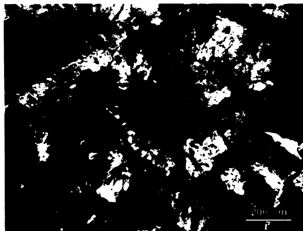
Obr. S.9.5. Výbrus č. 9 – PM: buňky sekundárního xylému jsou ve středu radiálně rostlých krystalů křemene, díky okolním výrazným interferenčním barvám křemene téměř nerozeznatelné; transverzální řez.
