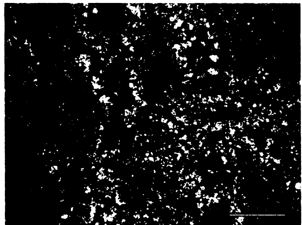
Obr. S.17.6. Výbrus č. 17 – PM: popis snímku jako na obr. vlevo. Dřevo je tvořeno mikrokrystalickým křemenem, v rekrytalizovaných úsecích převažují různé veliké krystaly makrokrystalického křemene (vysoké interferenční barvy); transverzální řez.
