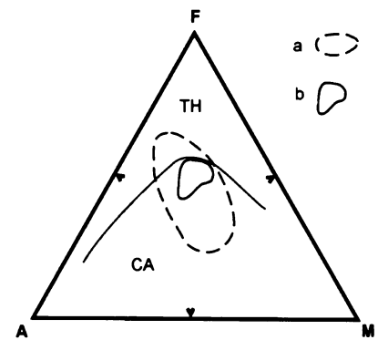
Obr. 21. Ternární AFM diagram s vyznačeným rozhraním mezi alkalicko-vápenatými a tholeitickými horninami. Porovnání chemického složení podkrkonošských „melafyrů“ (b) s „melafyrů“ střední Evropy (a); převzato ze Šreinové & Šreina (1997).
