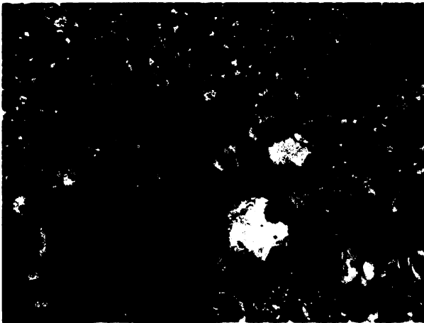
Obr. S.13.8. Výbrus č. 13 – PM: v šedé základní hmotě mikrokrytalického křemene se místy nacházejí obrovské krystaly hypidiomorfní makrokrytalického křemene, s vysokými interferenčními barvami.
