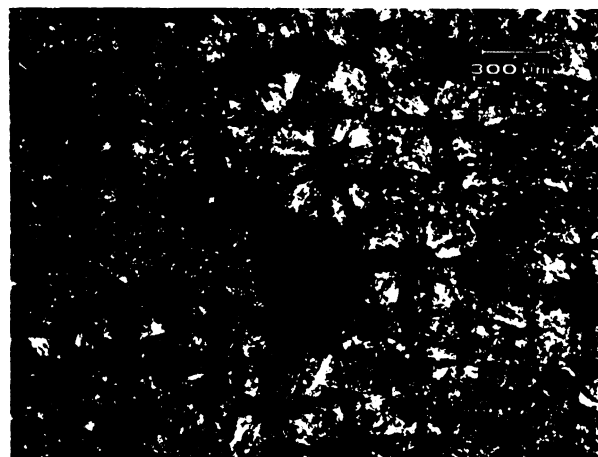
Obr. S.8.11. Výbrus č. 8 – PM: popis snímku jako u obr. vlevo, chalcedon vytváří oranžovohnědé sférolity ve tvaru „hvězdiček“ obklopené šedivým mikrokrytalickým křemenem; transverzální řez.
