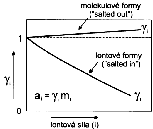
Obr. 2. Závislost aktivních koeficientů látek na iontové síle roztoku. Kyselina křemičitá patří mezi molekulové formy, které mají \gamma_i > 1 .
