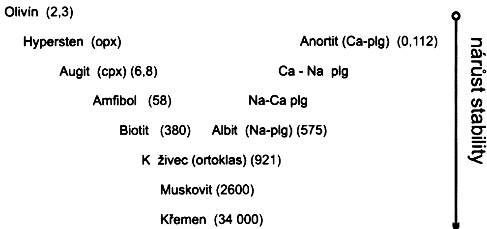
Obr. 3. Vzárust stability minerálů za stejných podmínek zvětrávání v exogenním prostředí, doba setrvání běžných horninotvorných minerálů v podmínkách zemského povrchu je uvedena červeně (v tisících let); podle Goldicha (1938).
