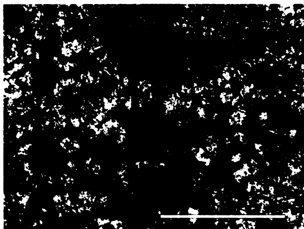
Obr. S.17.11. Výbrus č. 17 – PM: kolmo na prasklinu (tmavá svislá rozdvojená linie táhnoucí se podél levé hrany snímku) se rozkládá silně rekrystalizovaný úsek, který nenávratně porušil strukturu dřeva. Tvoří ho zejména makrokrytalický křemen; transversální řez.
