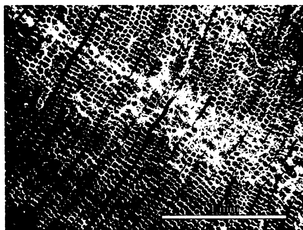
Obr. S.7.17. Výbrus č. 7 – OM – oblast 1 (CL); 4 až 8 řad tracheid tvoří pásy sekundárního xylému obklopené tmavými paprsky dřevního parenchymu. Příčně přes tuto strukturu (na snímku diagonálně) prochází narušená rekrystalizovaná vybělená zóna; transversální řez.
