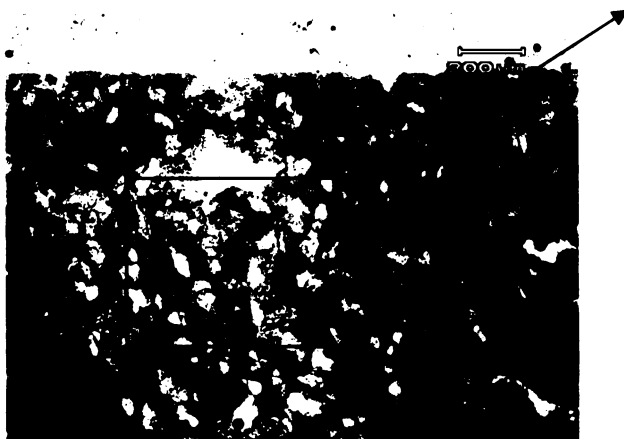
Obr. S.5.23. Výbrus č. 5b – OM/(EDX): optická fotografie sedimentárního okolí oblasti 2, z kterého byl udělána průměrná analýza. Vybraná oblast bodu 2 (v červeném obdélníku; blízko tůhliny) byla podrobněji analyzována.
