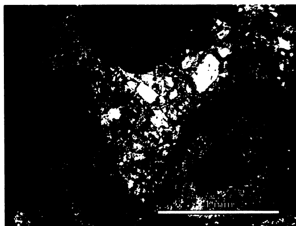
Obr. S.18.8. Výbrus č. 18 – OM: heterogenní detritický materiál uzavřený v prohlubni mezi lalokovitými a bochníkovitými strukturami; transverzální řez.
