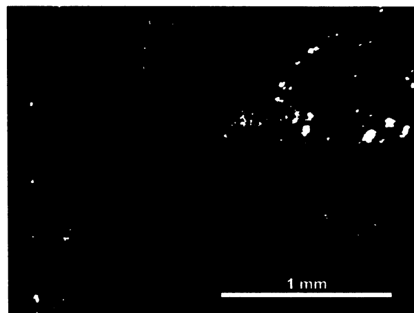
Obr. S.3.14. Výbrus č. 3b – CL: červeně, modře a fialově luminiskující objekty, v dolní polovině snímku vpravo je pravděpodobně triletní spora. Žlutá zrnka jsou zbytky diamantového leštidla; transversální řez.
