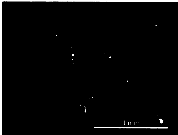
Obr. S.9.11. Výbrus č. 9 – CL: velké krystaly křemene mají červenofialovou CL a projevuje se na nich zonalita, a to ze strany kde byly v kontaktu s hydrotermálním roztokem. Mikrokrystalický křemen má krátce-žijící modrou CL a vznikl pravděpodobně v druhé fázi silicifikace po průniku hydrotermálního roztoku. Žlutá svítivá zrnka jsou zbytky diamantového leštidla.
