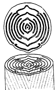
Obr. C.2. Schéma uspořádání cévních svazků v kmeni distichického typu psaronií, převzato z Němejce (1963).
