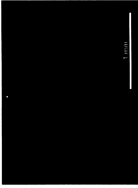
Obr. S.14.11. Výbrus č. 14 – CL – oblast 1: popis snímku jako na obr. vlevo, světlá část dřeva má jasně modrou CL, narozdíl od Fe pigmentované oblasti, která má CL červenou, hranice obou barev je poměrně ostrá.
