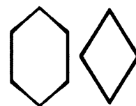
Obr. 6. Idiomorfní tvary křemene.
