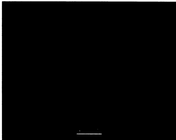
Obr. 30. Výbrus č. 6 – CL: popis snímku jako na obr. vlevo, každý typ krystalů \text{SiO}_2 poskytuje jinou CL. V buňkách je hnědočervená CL makrokrytalického křemene, v základní hmotě převažují různé odstíny červené CL mikrokrytalického křemene, kopírující původní strukturu pletiva, zde zejména tracheid.
