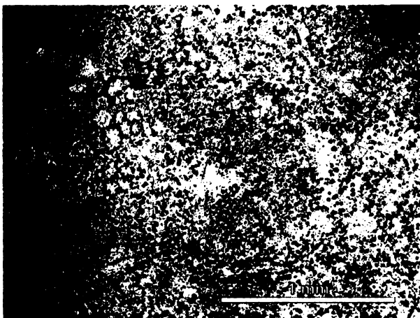
Obr. S.5.11. Výbrus č. 5b – OM: transverzální průřez psaroniovým kořínkem, tmavší sklerenchymatická pochva je špatně viditelná, vlevo uprostřed lze najít dochované buňky cévního svazku. Volně rozptýlené hnědé tečky jsou železitý pigment.
