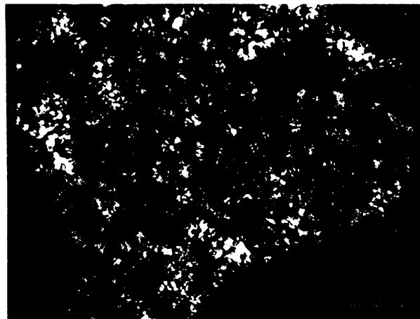
Obr. S.5.8. Výbrus č. 5a – PM: popis snímku jako na obr. vlevo. V oblasti parenchymu či aerenchymu jsou přítomny oranžovohnědé sférolity chalcedonu, obklopené makrokryalickým křemenem. Mikrokrystalický křemen permineralizoval buněčné stěny tracheid cévního svazku a sklerenchymatickou pochvu.
