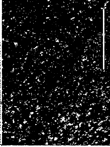
Obr. S.16.17. Výbrus č. 16 - PM: popis snímku jako na obr. vlevo a nahofé. Ve zkřížených nikolech se jednotlivé linie dřeva téměř ztrácí, převažuje pouze obraz jemných krystalů mikrokrytalického křemene. Vysoké interferenční barvy způsobila tloušťka výbrusu.
