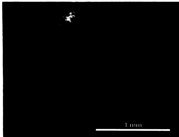
Obr. S.10.15. Výbrus č. 10 – CL – Bod 4: rozhraní dvou odlišných struktur, podobně jako na obr. S.10.13. (vlevo struktura anorganického původu tvořená chalcedonem, vpravo řady tracheid sekundárního xylému), výrazná pigmentace oxidy železa (tmavě karmínová CL).
