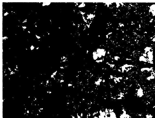
Obr. S.4.11. Výbrus č. 4b - PM: popis snímku jako na obr. vlevo. Chalcedonové výplně parenchymatických buněk z oblasti diktyostélé mají oranžovohnědou barvu. Oxidy železa v okolí praskliny jsou tmavě rezavé až černé a v některých místech kontaminovaly i buněčné stěny nejbližších buněk.
