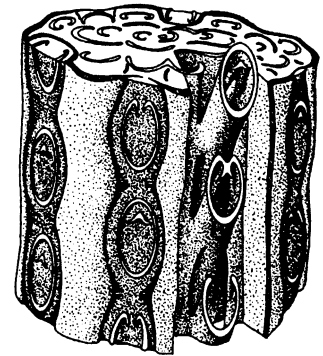
Obr. C.9. Rekonstrukce cévního systému psaroniového stonku (vlevo): listové stopy (lt); transverzální průřez. Převzato ze Stewarta & Rothwella (1993).
