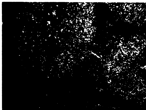
Obr. S.4.7. Výbrus č. 4a - PM: popis snímku jako na obr. S.4.5, ale chybí chalcedon uvnitř kořínků, místo toho se v centru zachoval cévní svazek. Hrubá prasklina v dolní levé polovině snímku zůstala nevyplněna. Výrazná je také tmavá pigmentace sklerenchymatických pochev a tkáně mezi kořínky.
