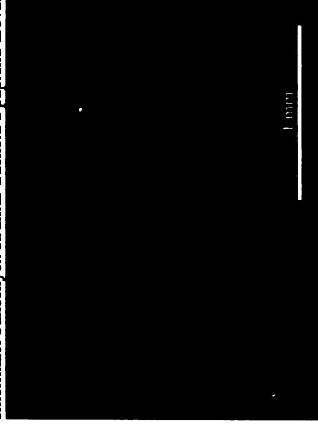
Obr. S.16.18. Výbrus č. 16 - CL: popis snímku jako na obrázcích vlevo. V levé polovině snímku je zachycena krátce-žijící modrá CL, která zobrazuje morfologii struktur mnohem lépe. Žlutá svítivá zrnka jsou zbytky diamantového leštidla.
