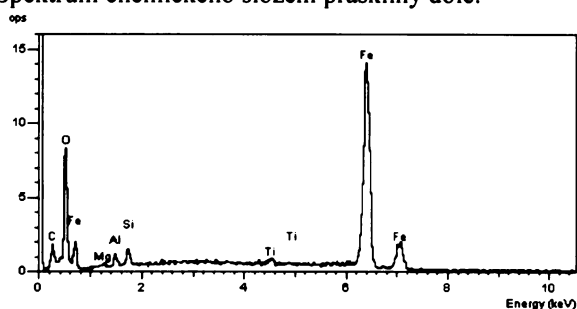
Obr. S.12.12. Výbrus č. 12 – SEM/EDX – oblast 1: prasklina v horní části výbrusu zobrazená detektorem BSE, vyplněná oxidy Fe s příměsí Ti; měřítko 200 \mu\text{m} ; transverzální řez. Spektrum chemického složení praskliny dole.
