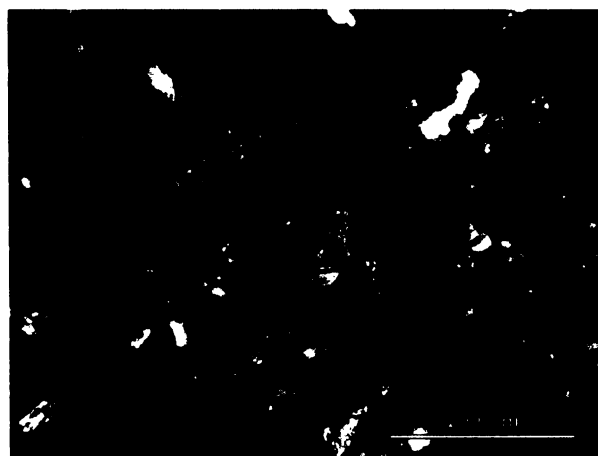
Obr. S.5.10. Výbrus č. 5a – PM: popis snímku jako na obr. vlevo. Krystal biotitu postižený hematitizací. Zirkon s pestrými interferenčními barvami uprostřed, granátové zrno vpravo nahoře od něj zhaslé; transverzální řez.
