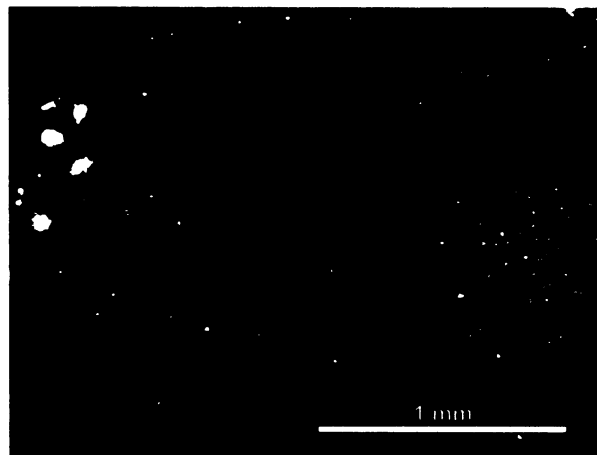
Obr. S.5.12. Výbrus č. 5b – CL: transverzální průřez psaroniovým kořínkem, sklerenchymatická pochva mnohem lépe patrná než v OM, stejně tak i intersticiální tkáň (protáhlé buňky v levém dolní rohu snímku). Převažuje červený odstín CL kořenového pláště. Žlutá svítivá zrnka jsou zbytky diamantového leštidla, zelenohnědá v dírách je barva podložního skla.
