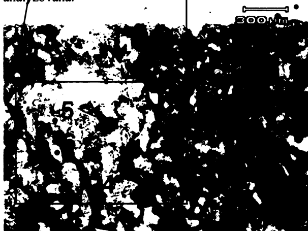
Obr. S.5.25. Výbrus č. 5b – OM/(EDX): optická fotografie klastického materiálu v oblasti 2) při větším zvětšení (červený obdélník). Číselná lokalizace analyzovaných minerálních zrn 1 - 6.
