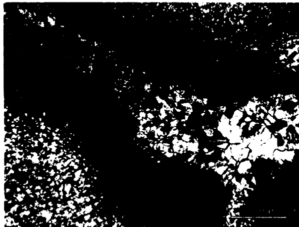
Obr. S.16.6. Výbrus č. 16 - PM: popis snímku jako na obr. vlevo, buňky sekundárního xylému perminalizuje mikrokrystalický křemen, prasklinu v jejím středu vyplňuje makrokrytalickým mozaikovitým křemenem; transversální řez.
