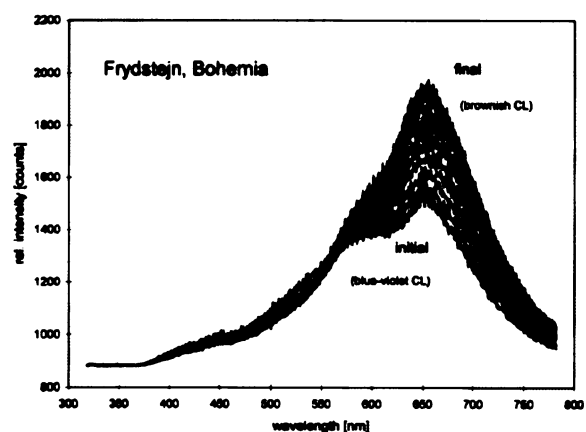
Obr. 15. Časově závislá CL spektra u achátu z Frydštejna podle Götzeho et al. (1999).
