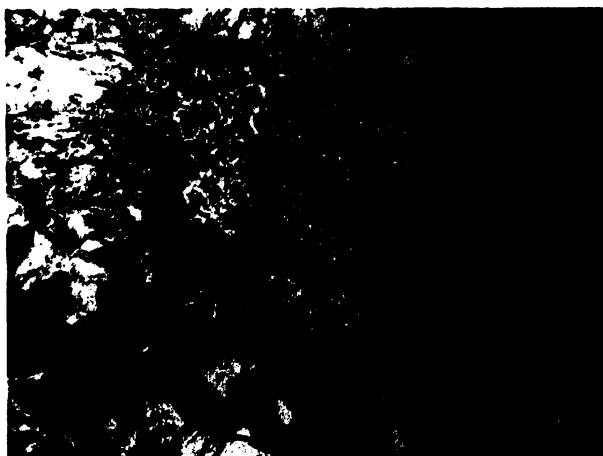
Obr. S.9.4. Výbrus č. 9 – OM: nahnědlé reliktů buněk sekundárního xylému v centru radiálně rostlého křemene; transverzální řez.
