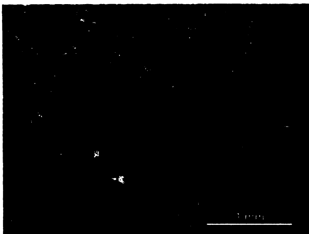
Obr. S.4.8. Výbrus č. 4b - OM: transverzální řez rozhraním parenchymatických buněk diktyostélé (levý horní roh snímku) a plátem stélé s tracheidovými buňkami (prochází snímek diagonálně). Tmavě hnědé struktury jsou krystaly chalcedonu (uvnitř buněk stélé) a také jeho sférolity (v parenchymu, levý horní roh).
