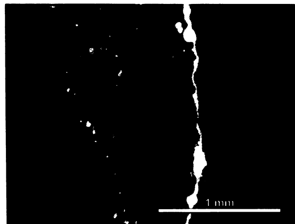
Obr. S.3.8. Výbrus č. 3b – CL: ukazuje dva odlišné odstíny CL silicifikované hmoty sedimentu (červený a fialový), přičemž další, a to modrý, lemují jednotlivé detritické struktury. Tyrkysová barva podložního skla prosvítá trhlinou ve výbrusu. Žlutá svítivá zrnka jsou zbytky diamantového leštidla; transversální řez.
