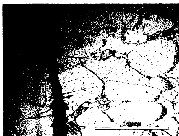
Obr. S.18.12. Výbrus č. 18 – OM: popis snímku jako na obr. S.18.10, oblast čirých karbonátových zrn, mezi kterými je vymezená tmavě pigmentovaná karbonátová vrstva; transverzální řez.
