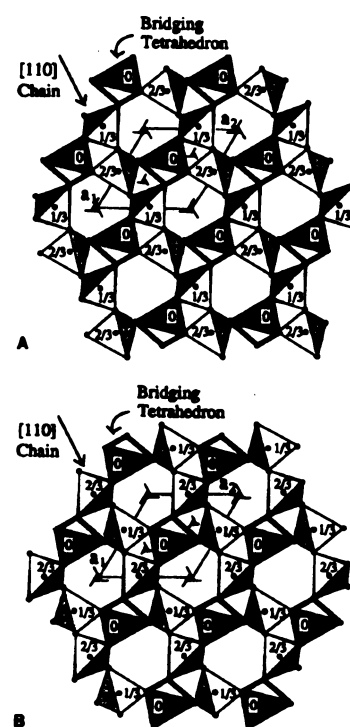
Obr. 12. Prostorová projekce křemene podél osy c . A – pravotočivá forma křemene (prostorová grupa P 3 21); B – levotočivá forma křemene (prostorová grupa P 3 121). Můstkové tetraedry jsou zvýrazněny tučně. Převzato z Heaneyho (1993).
