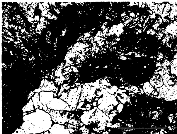
Obr. S.18.6. Výbrus č. 18 – OM: rozhraní centrální dutiny stonku přesličky a oblasti karinálních kanálů s metaxylémem a relikty vyběhajícího sekundárního xylému (v levé části snímku), uprostřed a vpravo centrální dutina vyplněná hypidiomorfními kalcitovými zrnky uzavírajícími detrit; transverzální řez.
