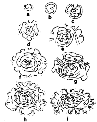
Obr. C.3. Sled příčných průřezů (a - i) stonku rodu Psaronius COTTA ukazuje spletitost cévního systému od báze k vrcholu, narůstá počet cyklů i listových stop; převzato ze Stewart & Rothwella (1993).
