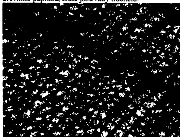
Obr. S.6.8. Výbrus č. 6b – PM: transverzální průřez sekundárním xylémem rodu Arthropitys (jako na obr. vlevo). Buněčné stěny tracheid jsou velmi tmavé, tvořené mikrokrytalickým křemenem, vnitřky buněk vyplňují krystaly makrokrytalického čírého křemene, které respektují buněčné stěny a jsou jimi omezeny v růstu. Jedná se o typickou polyblastickou texturu.
