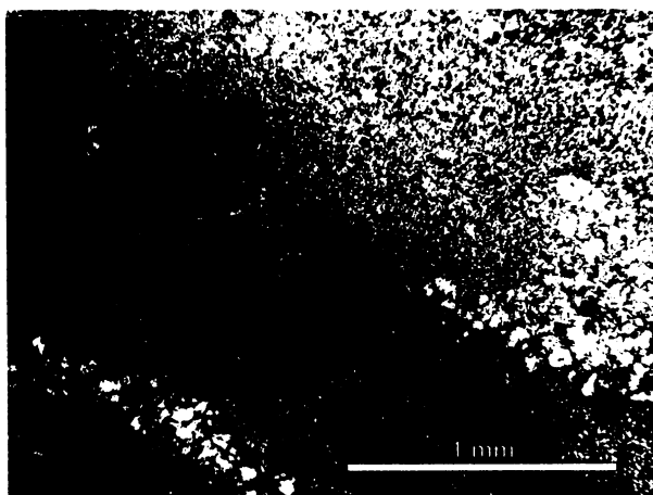
Obr. S.5.13. Výbrus č. 5b – PM: transverzální řez na rozhraní diktyostélé a kořenového pláště. Převažuje mikrokrystalický křemen, v dutině prohnutého stélé chalcedon. Volně rozptýlené hnědé tečky jsou železitý pigment.
