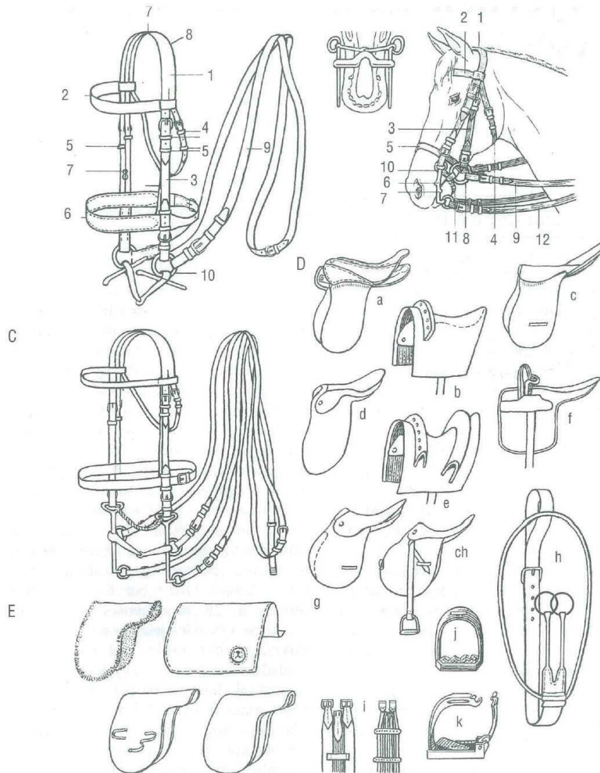
49. Jezdecká výstroj: A – uzdečka: 1 – nátylník s podhrdelníkem, 2 – čelenka, 3 – lícnice, 4 – průvlečky, 5 – posuvky, 6 – nánosník, 7 – zápřezek k nátylníčku, 8 – nátylníček, 9 – otěže, 10 – udidlo (roubíčkové), B – uzda: 1 – nátylník, 2 – čelenka, 3 – lícnice, 4 – podhrdelník, 5 – nánosník, 6 – pákové udidlo, 7 – dolní rameno páky s kroužkem pro zapnutí otěže, 8 – udidlo, 9 – otěže od udidla, 10 – horní rameno páky s háčky na podbradní řetízek, 11 – podbradní řetízek, 12 – pákové otěže, C – pelham, D – sedla: a – armádní kozlík, b – francouzské drezurní sedlo pro vysokou španělskou školu, c – anglické školní sedlo, d – drezurní sedlo, e – pikadorské sedlo, f – dámské sedlo, g – sedlo pro skokové soutěže, h – jednoduchý martingal, ch – dostihové sedlo, i – dvojitý podbřišník popruhový a praménkový kožený nebo provázkový, j – třmen normální, k – pojistný, E – podložky pod sedla.
