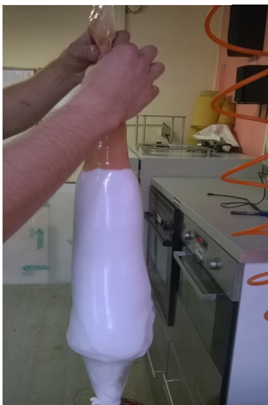
Lití pryskyřice – využití vakua Zdroj: autor práce
