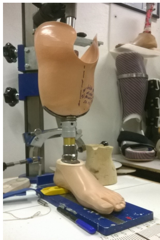
Bércová protéza Zdroj: autor práce
