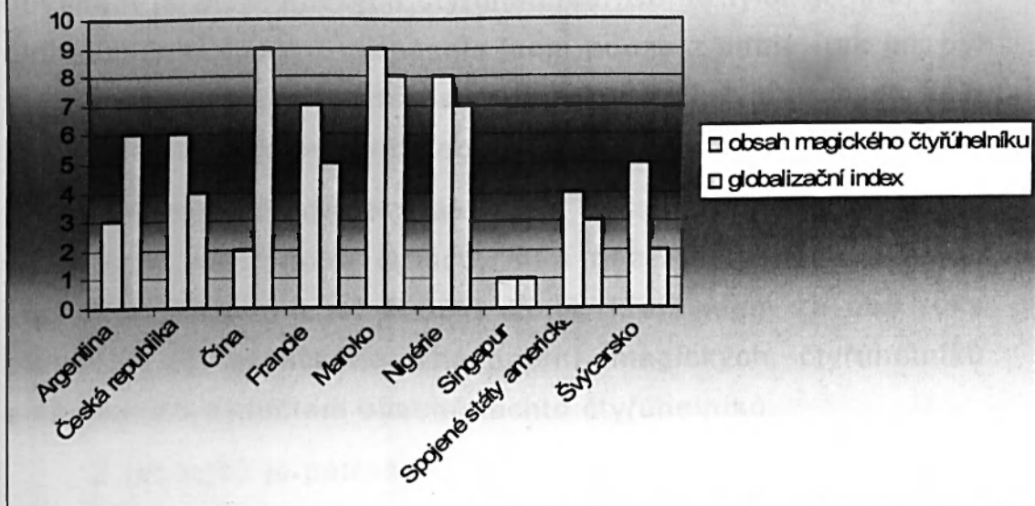
graf č. 4 – Srovnání obsahu magického čtyřúhelníku a globalizačního indexu v roce 2004
