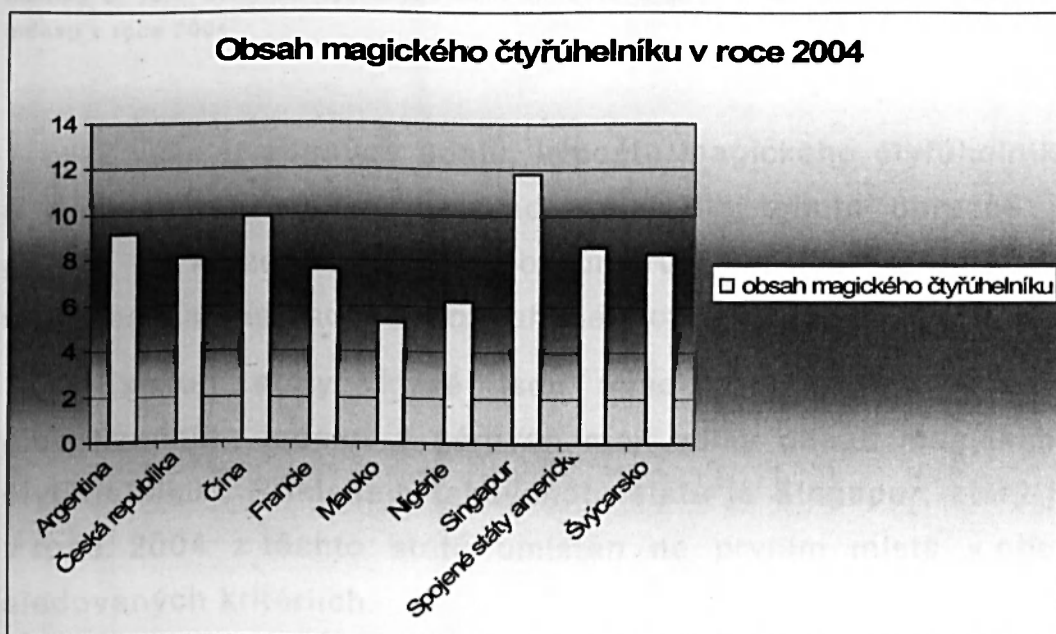
graf č. 2 – Obsah magického čtyřúhelníků v roce 2004
