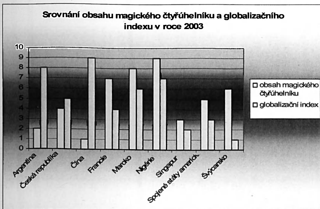
graf č. 3 – Srovnání obsahu magického čtyřúhelníku a globalizačního indexu v roce 2003
