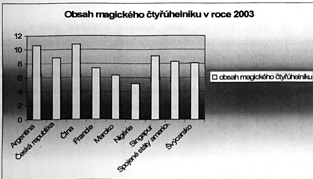
graf č. 1 – Obsah magického čtyřúhelníků v roce 2003
