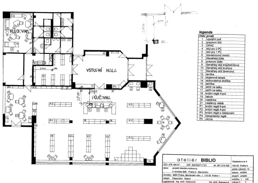
Obr. č. 58 Plánek knihovny Barrandov před proměnou knihovny v roce 2014, zdroj: archiv MKP
