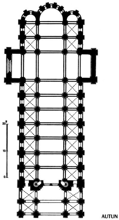
67. Autun, Saint-Lazare, půdorys chrámu
