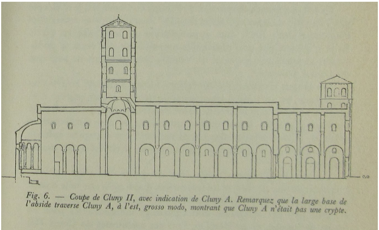
33. Cluny II., podélný řez předpokládanou rekonstrukcí kostela, K. J. Conant,
