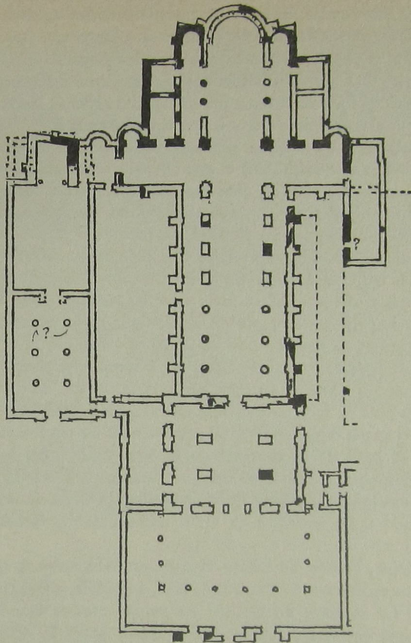
Fig. 2. — Plan de Cluny II (c. 950-981) avec le Galilée (c. 991-1000?) ; à gauche: hypothétique Cluny I (dédiacé 927) avec la Tour (1020-1030) ; à droite: chapelle au sarcophage (c. 915?).
