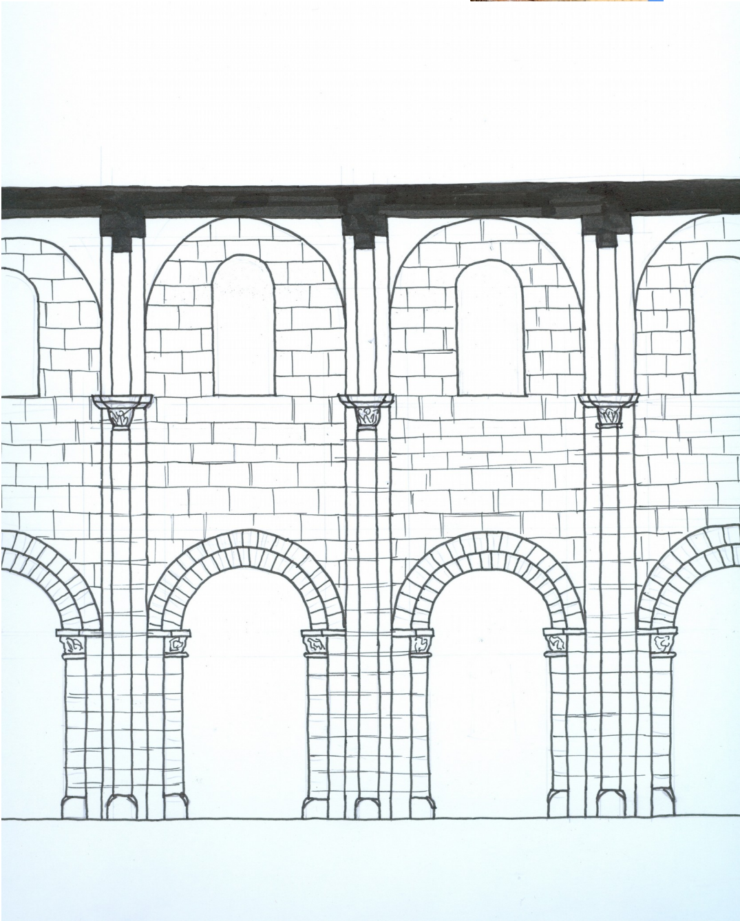
76. Anzy-le-Duc , Notre-Dame, studie rozdělení stěny v hlavní lodi chrámového interiéru, vlastní kresba
