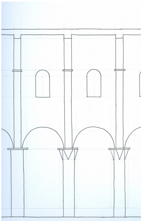
34. Cluny II. , studie elevace stěny v chrámovém interiéru kostela, vlastní kresba
