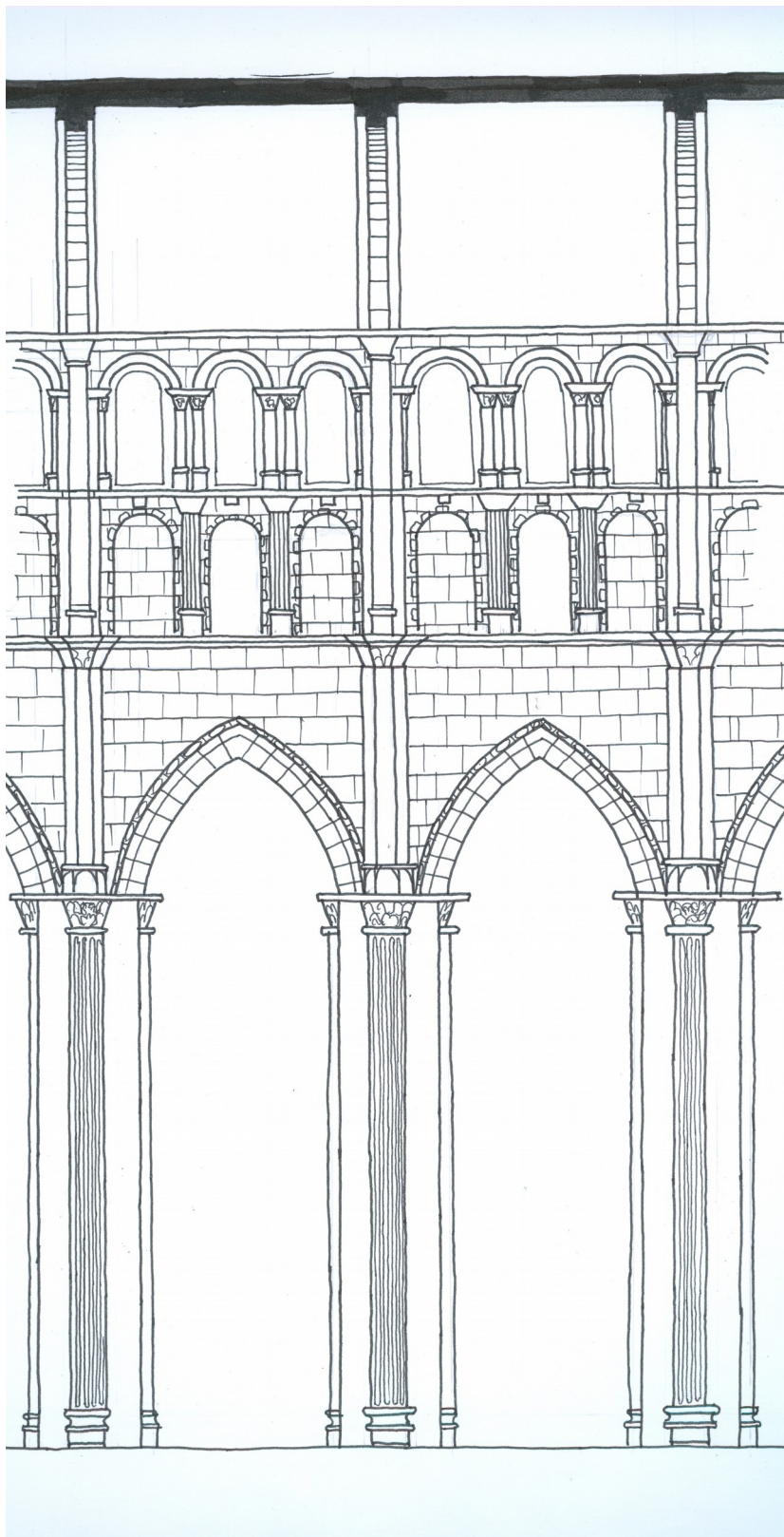
19. Cluny III, studie rozdělení stěny v hlavní lodi chrámového interiéru, vlastní kresba
