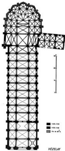
64. Vézelay, chrám Máří Magdaleny, půdorys 65. Vézelay, chrám Máří Magdaleny, vedlejší loď
