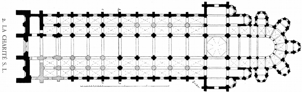
44. La Charite-sur-Loire, Notre-Dame, půdorys kostela
