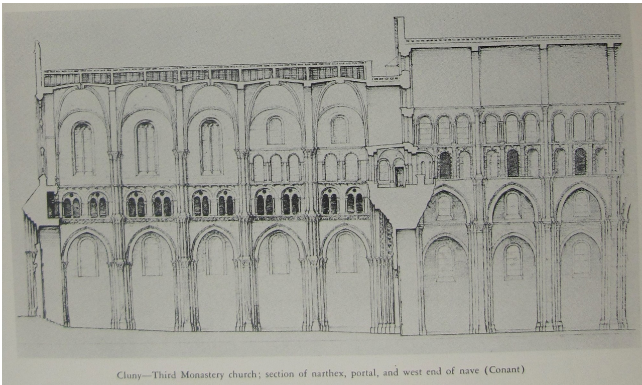
14. Cluny III., rekonstrukce podélného řezu nartexem a částí chrámové lodi, K. J. Connant
