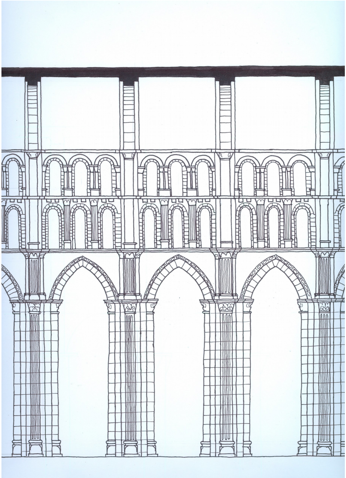
60. Paray le Monial, Notre-Dame, studie rozdělení stěny v hlavní lodi, vlastní kresba
