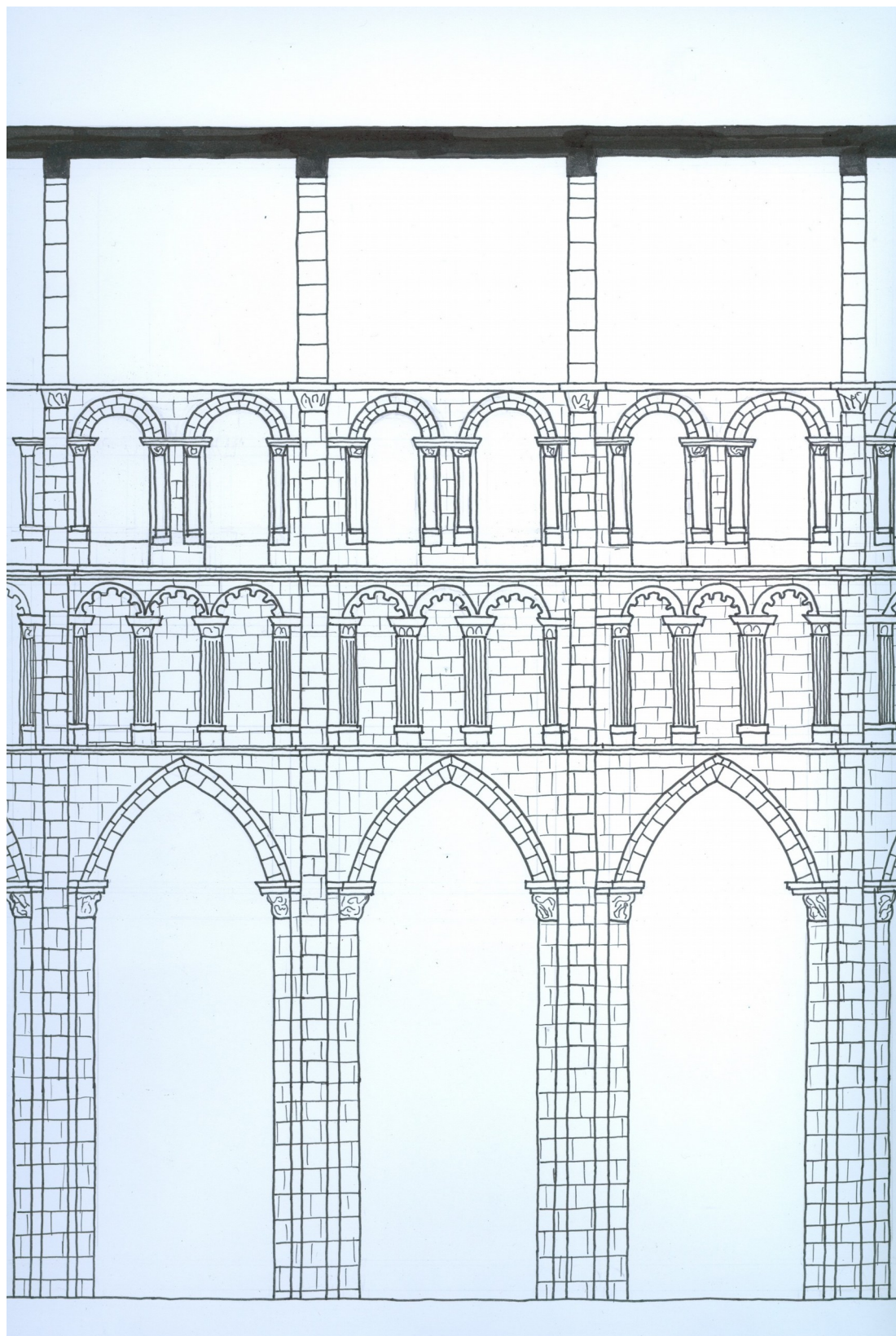
49. La Charite-sur-Loire, Notre-Dame, studie rozdělení stěny v hlavní lodi v chórové části, vlastní kresba
