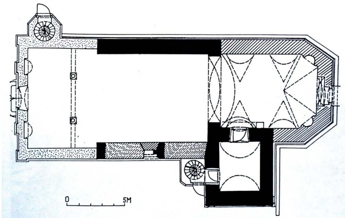
8. Velké Popovice, kostel Panny Marie Sněžné, řez přízemím stavby, analýza stavebního vývoje. Černě položené je zdivo gotické, čárkované barokní, přerušované čárkované hypoteticky barokní, tečkované konec 19. století, neznačené je neurčené.
