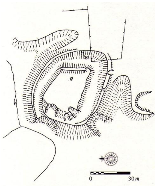
2. Velké Popovice, náčrt tvrziště. Stav v roce 1985
