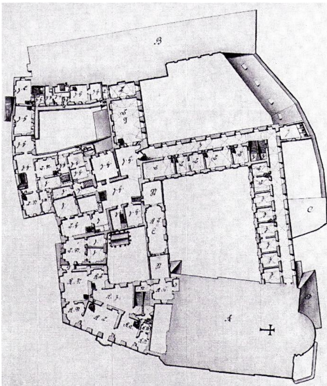
18. Konvent benediktinů na Starém Městě, půdorys 1. patra, konec 18. století
