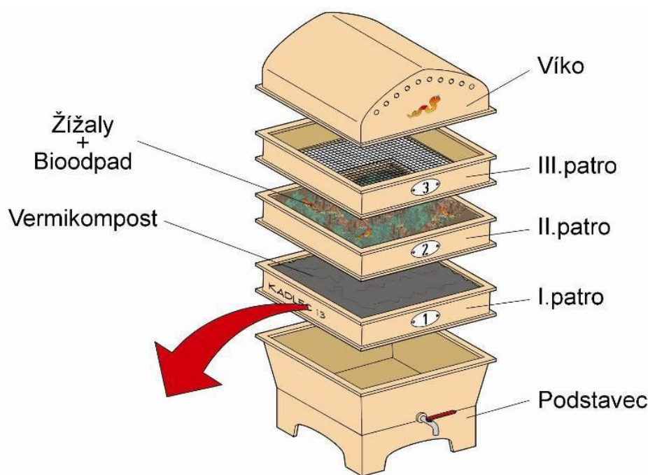
Obr. I: Schématické znázornění domácího vermikompostéru [Hanč, Plíva, 2013:
