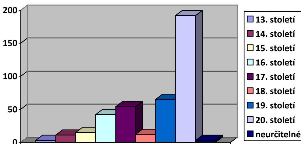
graf 2 – časové zařazení jednotlivých mincí – Jihlava (13)
