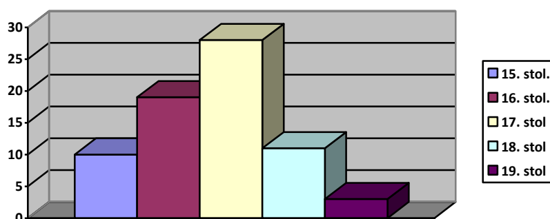
graf 1 – časové zařazení jednotlivých mincí – Prachatice (6)
