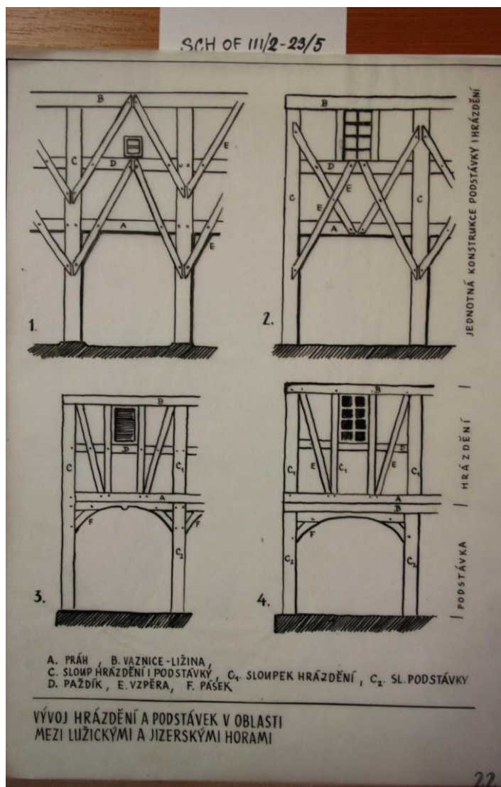
40. Josef Václav Scheybal: kresebná dokumentace vývoje hrázdění a podstávek v oblasti mezi Lužickými a Jizerskými horami, 1977, kresba tužkou, papír, 21 x 29 cm. Archiv Muzea Českého ráje v Turnově
