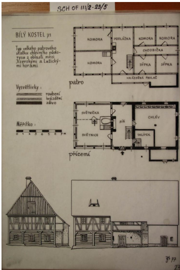
41. Josef Václav Scheybal: Bílý kostel 71, dokumentátorská kresba s půdorysnými plánky a 2 pohledy, 1977, kresba tuší, papír, 21 x 29 cm. Archiv Muzea Českého ráje v Turnově
