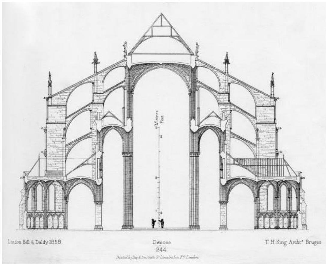
47. Le Mans , katedrála svatého Juliána (Saint-Julien), řez
