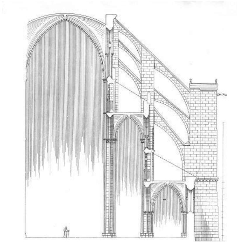
53. Bourges , katedrála svatého Štěpána (Saint-Étienne), řez
