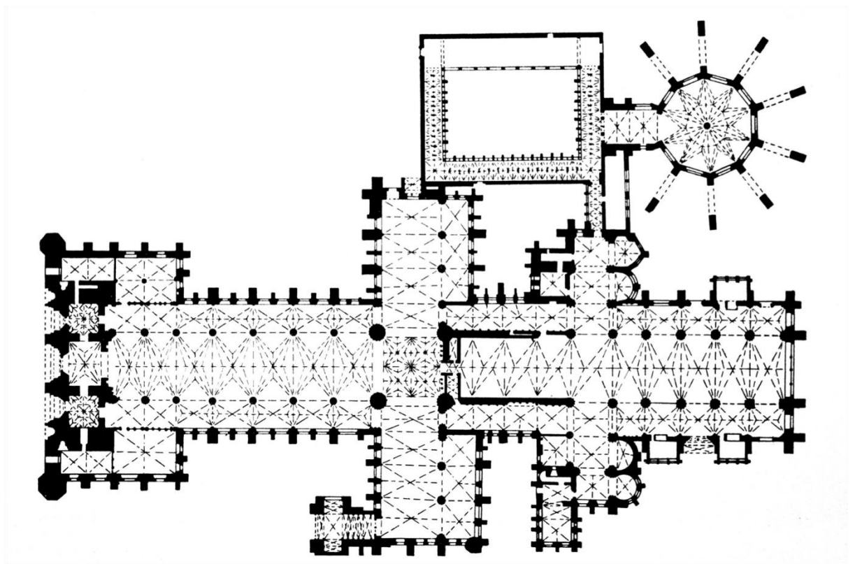
69. Lincoln, Lincolnská katedrála Panny Marie, půdorys
