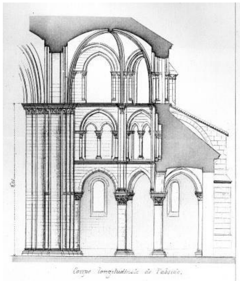
6. Domont , kostel svaté Máří Magdaleny (Sainte-Marie-Madelene), řez
