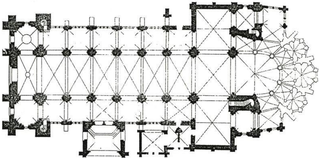
33. Châlons-sur-Marne (en-Champagne), kolegiální kostel Notre-Dame-en-Vaux, půdorys
