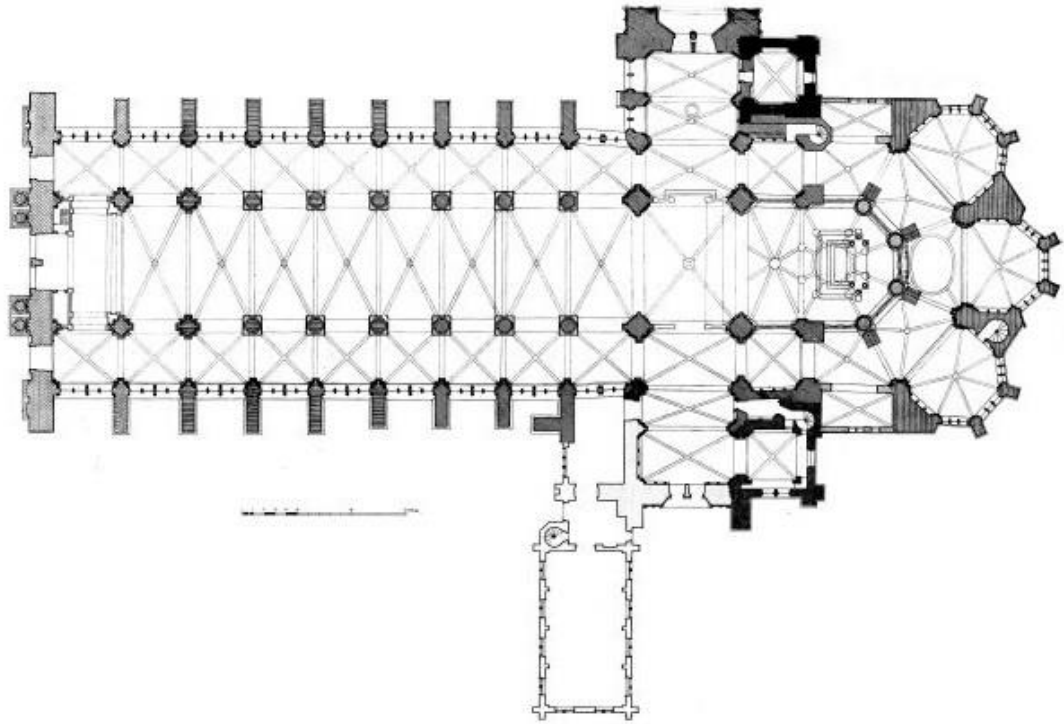
61. Châlons-sur-Marne (en-Champagne), katedrála svatého Štěpána (Saint-Étienne), půdorys
