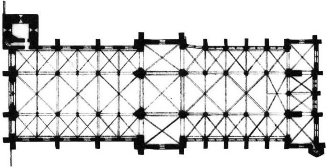
27. Champeaux, kolegiální kostel svatého Martina (Saint-Martin), půdorys
