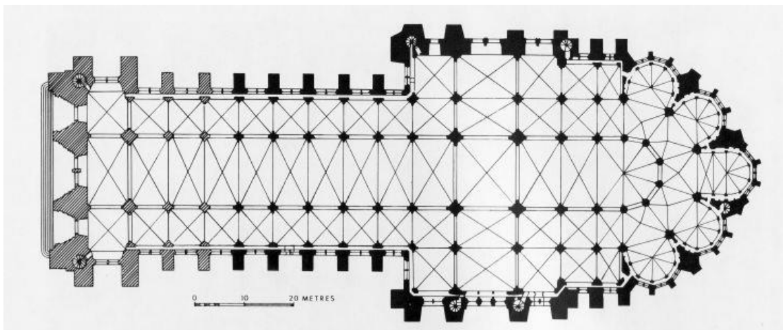
50. Reims (Remeš), katedrála Panny Marie (Notre-Dame), půdorys
