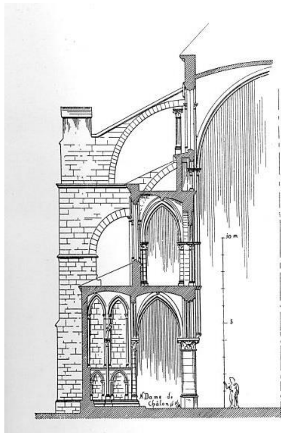
34. Châlons-sur-Marne (en-Champagne), kolegiální kostel Notre-Dame-en-Vaux, řez
