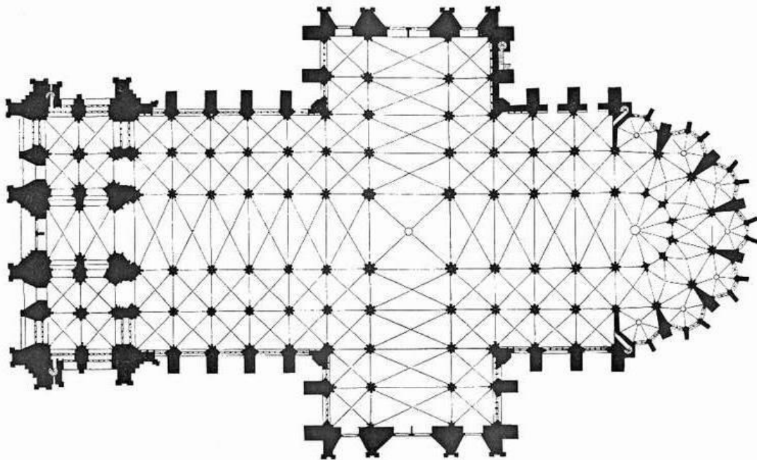
90. Kolín nad Rýnem, katedrála sv. Petra, půdorys
