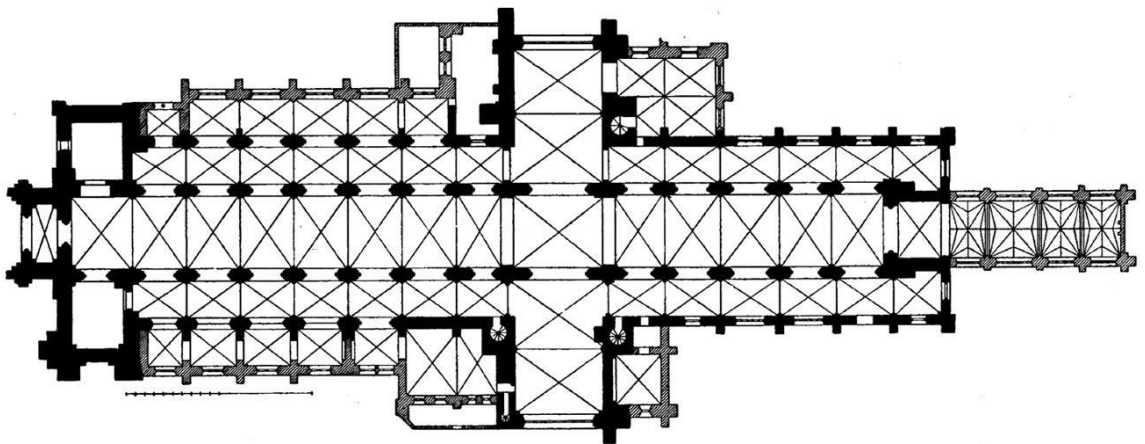
67. Chichester , Chichesterská katedrála Nejsvětější Trojice, půdorys
