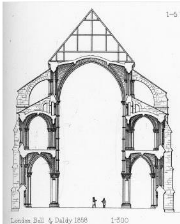
43. Laon , katedrála Panny Marie (Notre-Dame), řez
