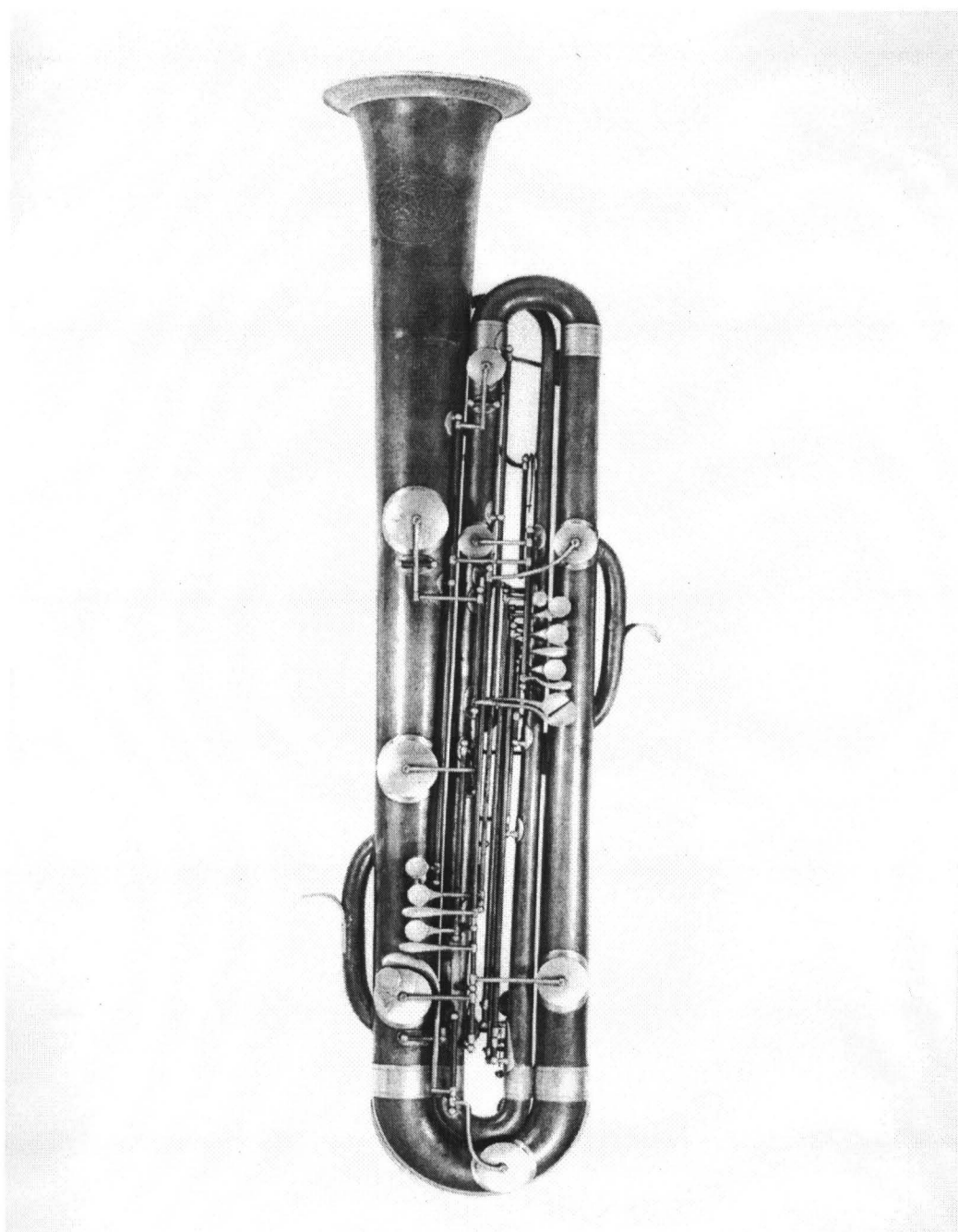
Tritonikon – poslední model po roce 1893 (Muzeum české hudby v Praze, hudební nástroje, sig. 1789 E.)
