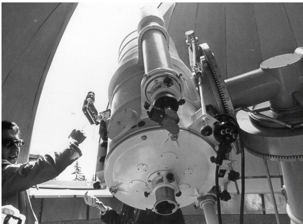
Meniscus Cassegrain, dalekohled v západní kopuli Štefánikovy hvězdárny, okolo roku 1976 (archív O. Hlada)
