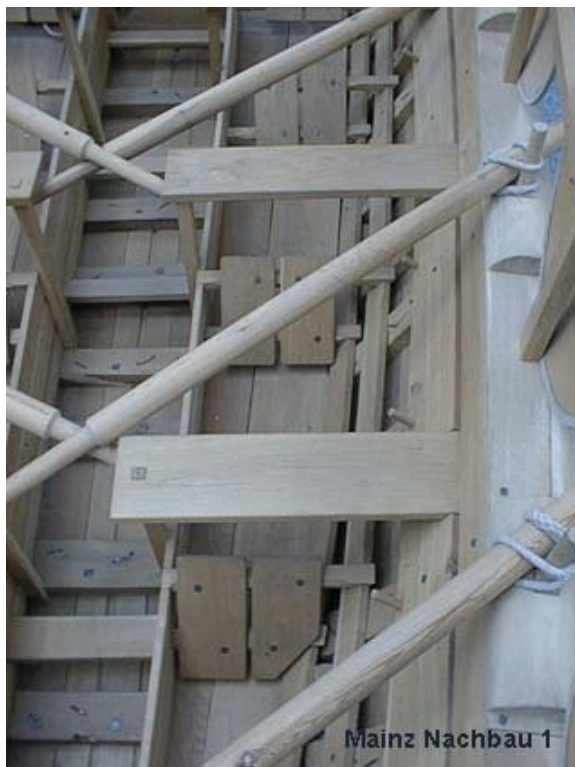
Obr.35 – rekonštrukcia veslárskoho systému lode typu Mainz A
