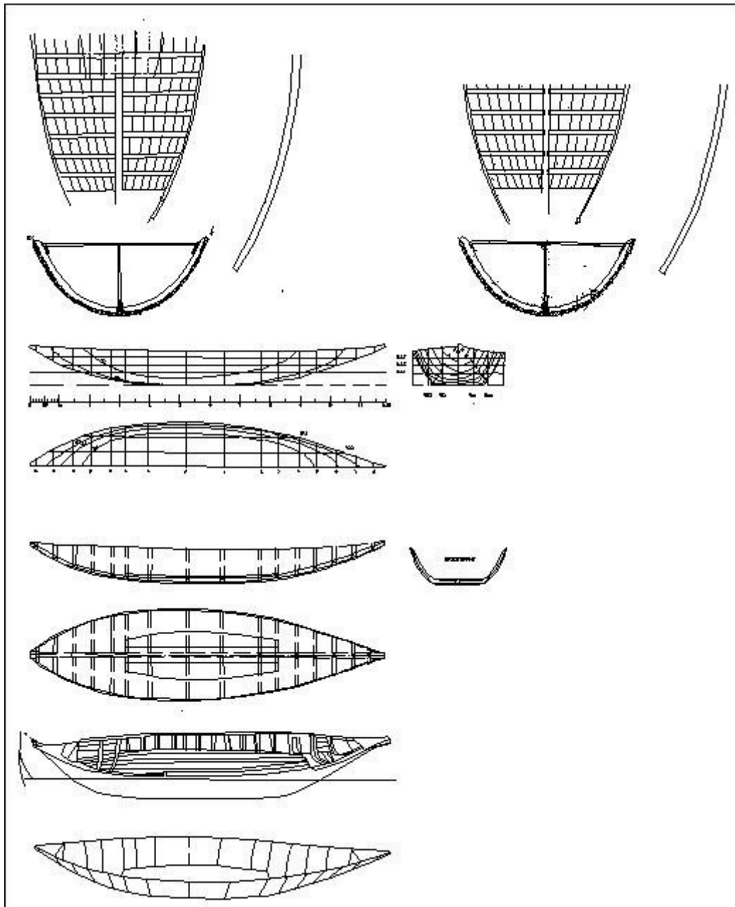
Obr.6 – rôzne rekonštrukcie lode z Vechtenu
