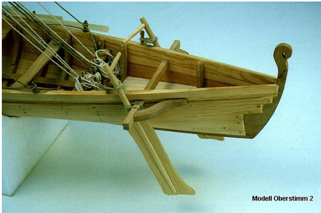
Obr.11 – kormovec modelu lode číslo 2 z Oberstimmu
