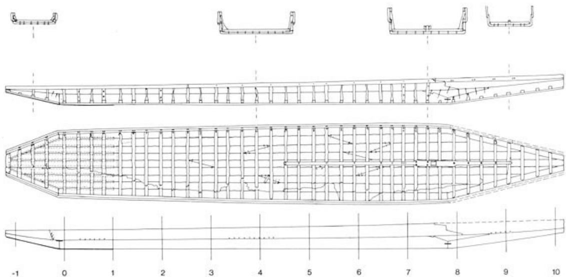
Obr.22 – plán lode číslo 2 z Zwammerdamu
