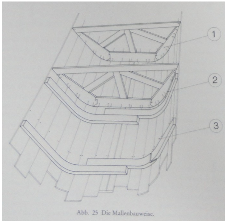
Obr.34 – použitie šablón pri stavbe lode typu Mainz A
