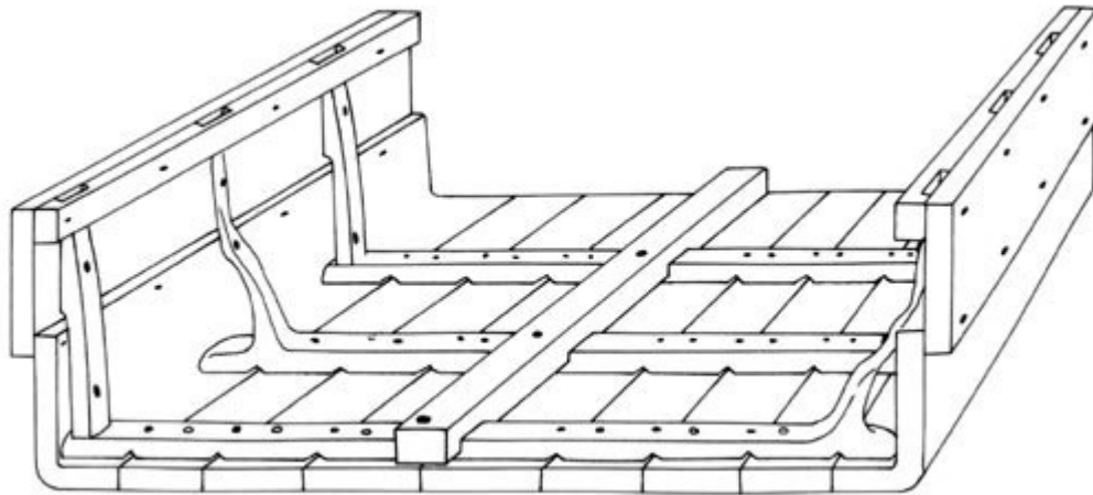
Obr.21 – priečny rez trupom lode číslo 2 z Zwammerdamu
