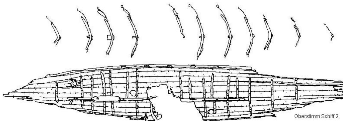
Obr.8 – lod' číslo 2 z Oberstimmu
