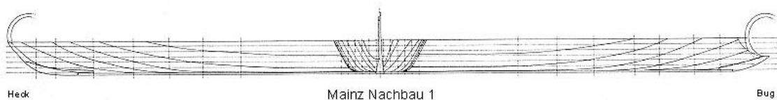
Obr.44 – plán a priečný rez trupu lode číslo Mainz A
