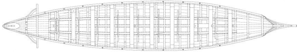
Obr.42 – plán trupu lode číslo 2 z Oberstimmu
