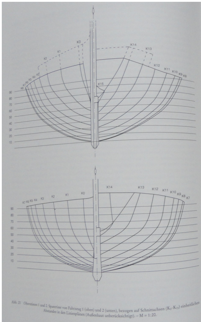
Obr.43 – priečný rez trupmi lodí číslo 1 a 2 z Oberstimmu
