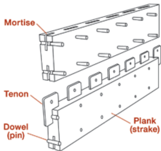
Obr.13 – tvorba obšívky trupu lode postavenej grécko-rímskym spôsobom
