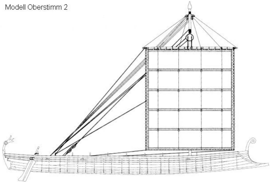
Obr.17 – rekonštrukcia oplachtenia lode číslo 2 z Oberstimmu
