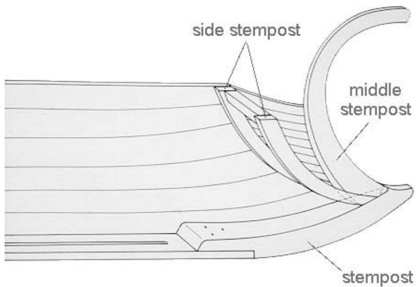
Obr.32 – stavba predného väzu lode typu Mainz A
