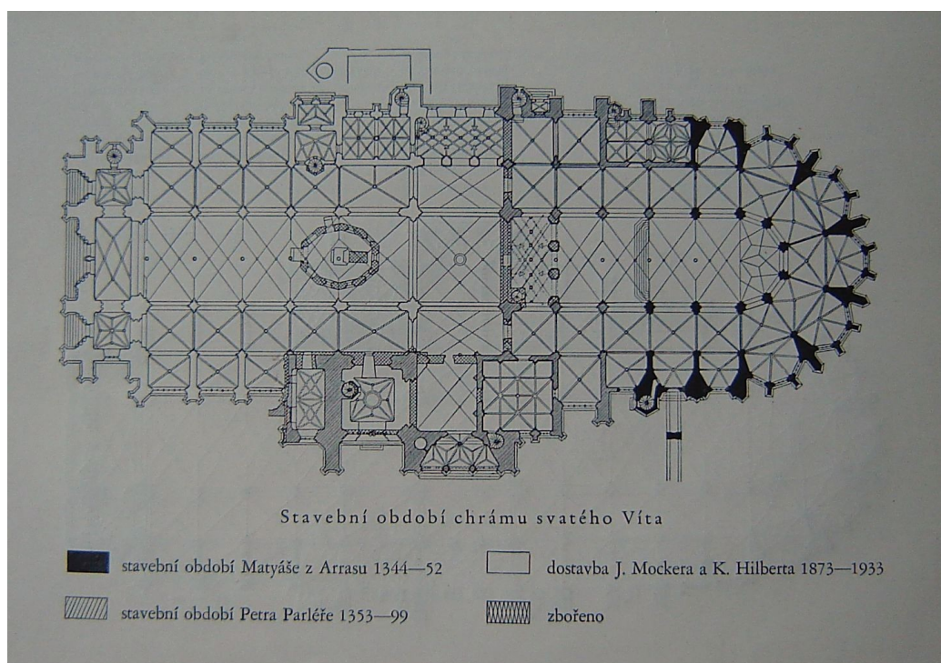
Obr. č. 6: Chrám sv. Víta zobrazující jeho stavební vývoj podle jednotlivých stavebních období. (Převzato z knihy Chrám sv. Víta v obrazech Jiřího Jeníčka ).
