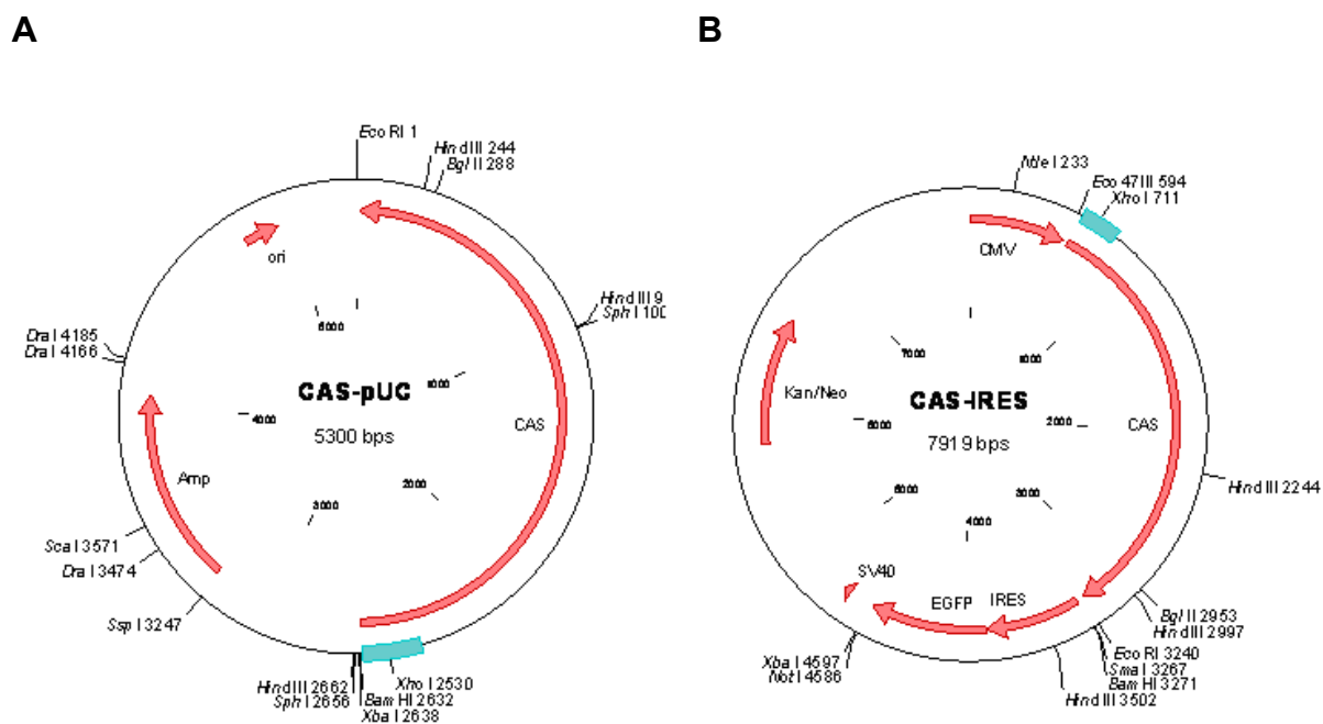
Obr. 5.3. A. Vektor pUC s vloženým CAS fragmentom. B. Vektor IRES-GFP s vloženým CAS fragmentom.
