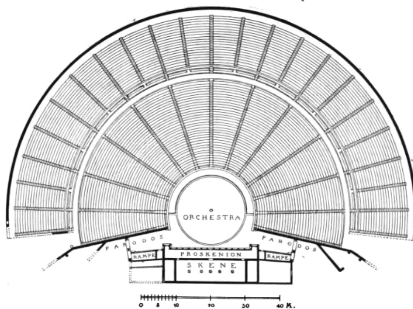
Figur 50. Grundriss des Theaters von Epidauros. Ergänzt.
