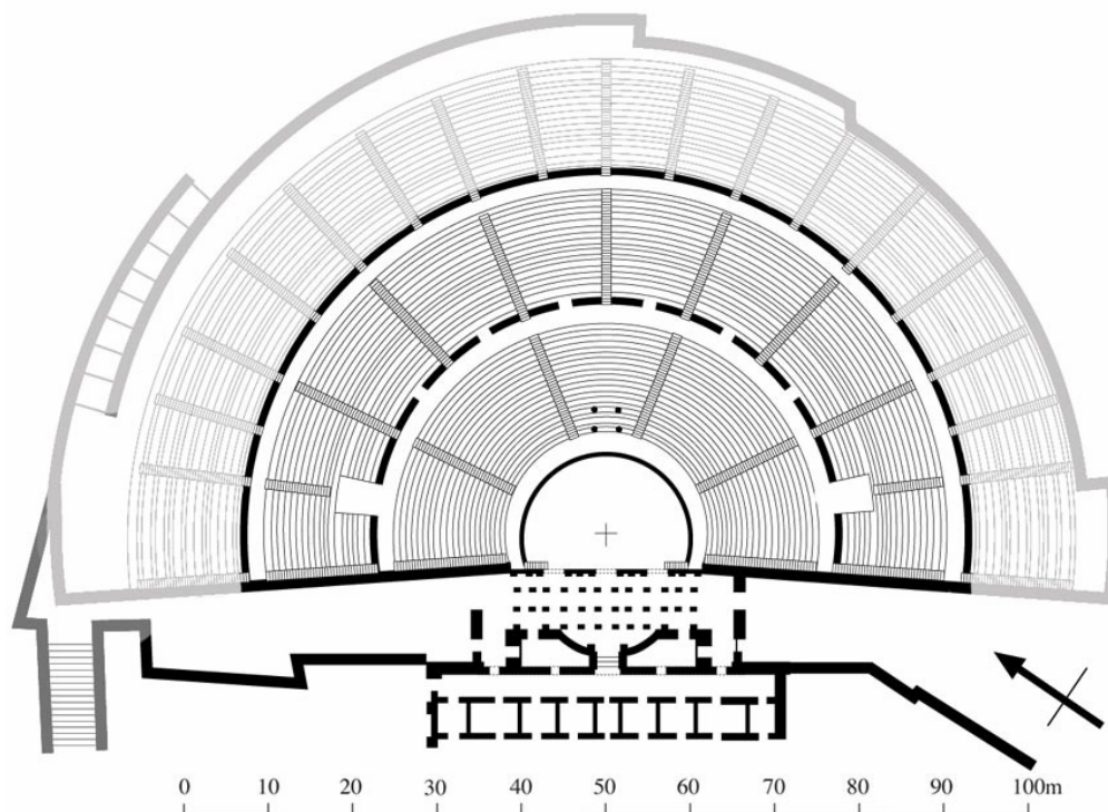
Obr. 9. Divadlo v Milétu. (Hines 2009).
