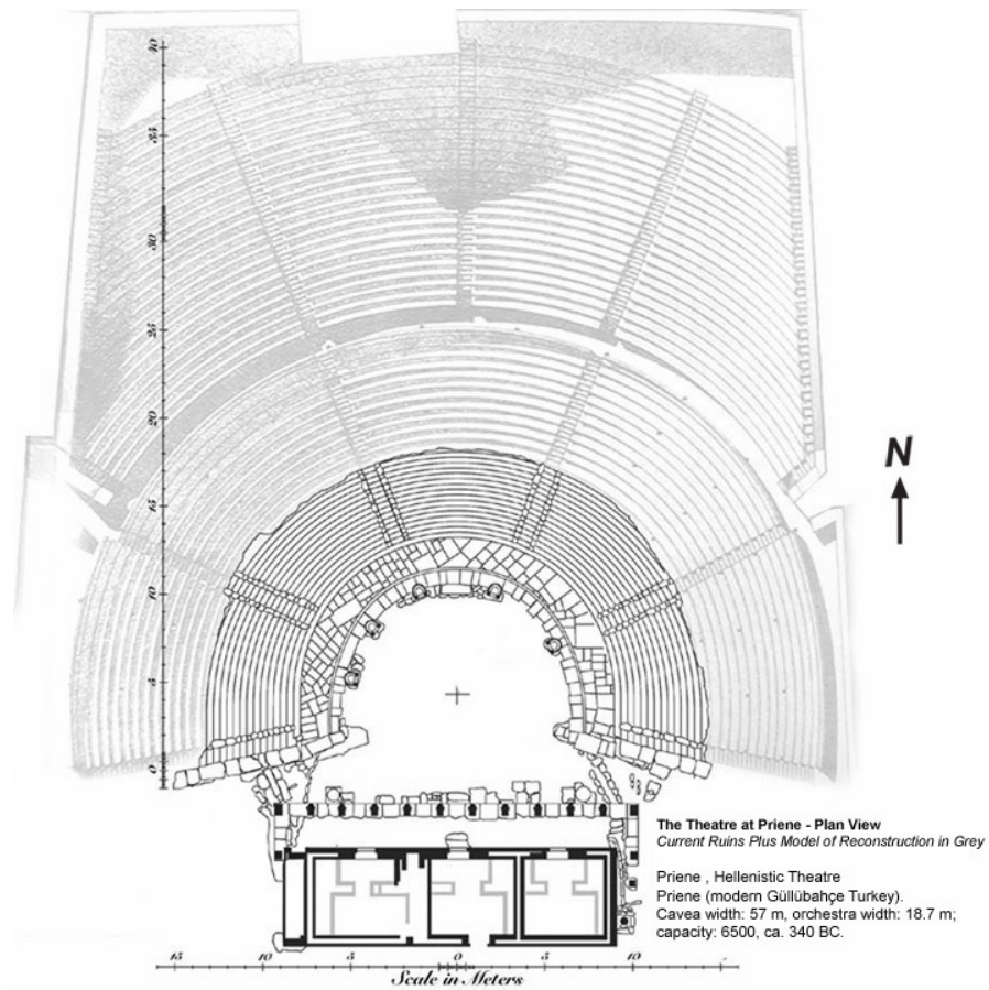
Obr. 11. Divadlo v Priené. (Heffernan 2003).
