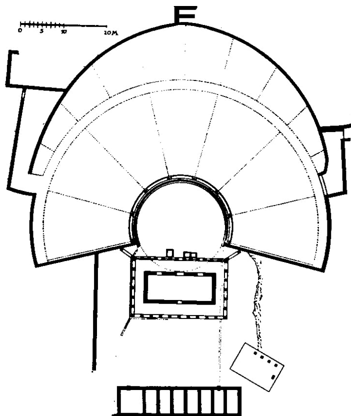
Figur 58. Grundriss des Theaters von Delos.
