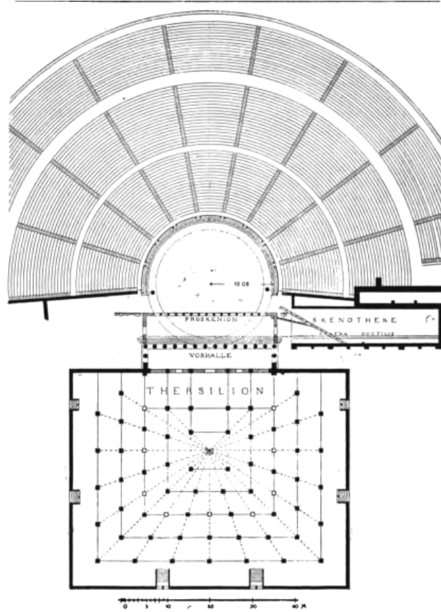
Figur 54. Grundriss des Theaters von Megalopolis.
