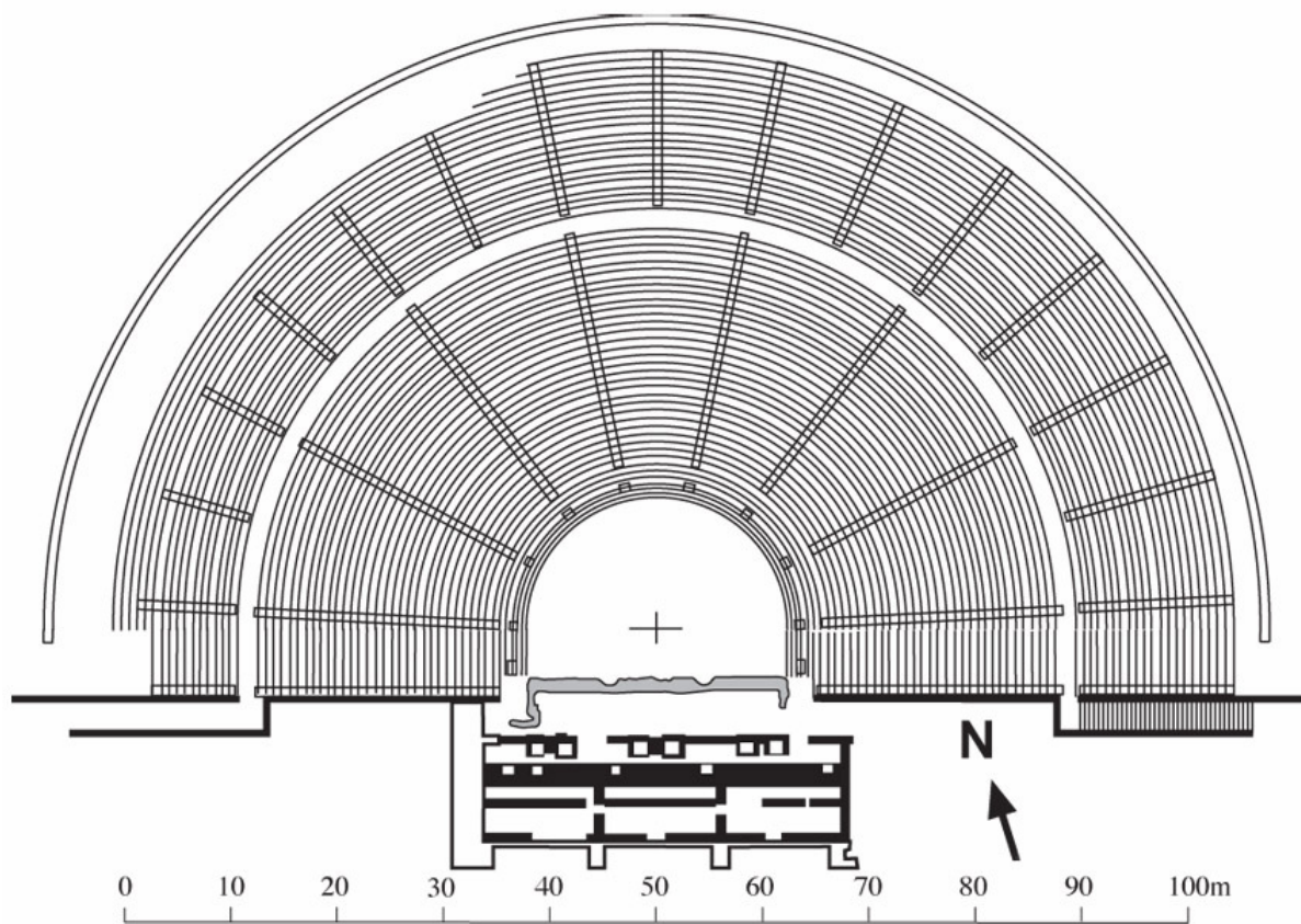
Obr. 20. Divadlo ve Spartě. (Hines 2009).
