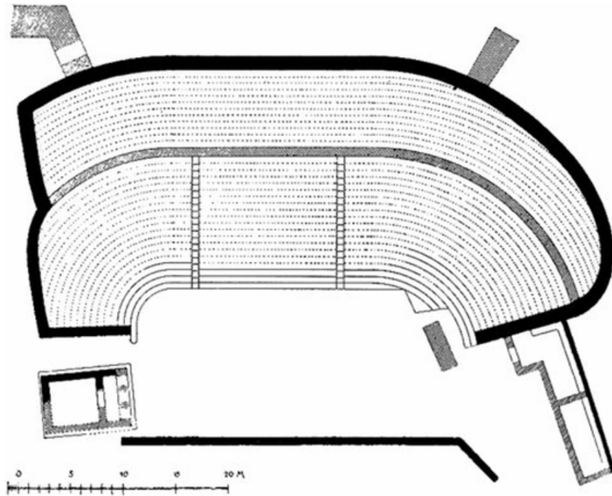
Obr. 7. Divadlo v Thoriku (Podle Dörpfelda 1896, 110).
