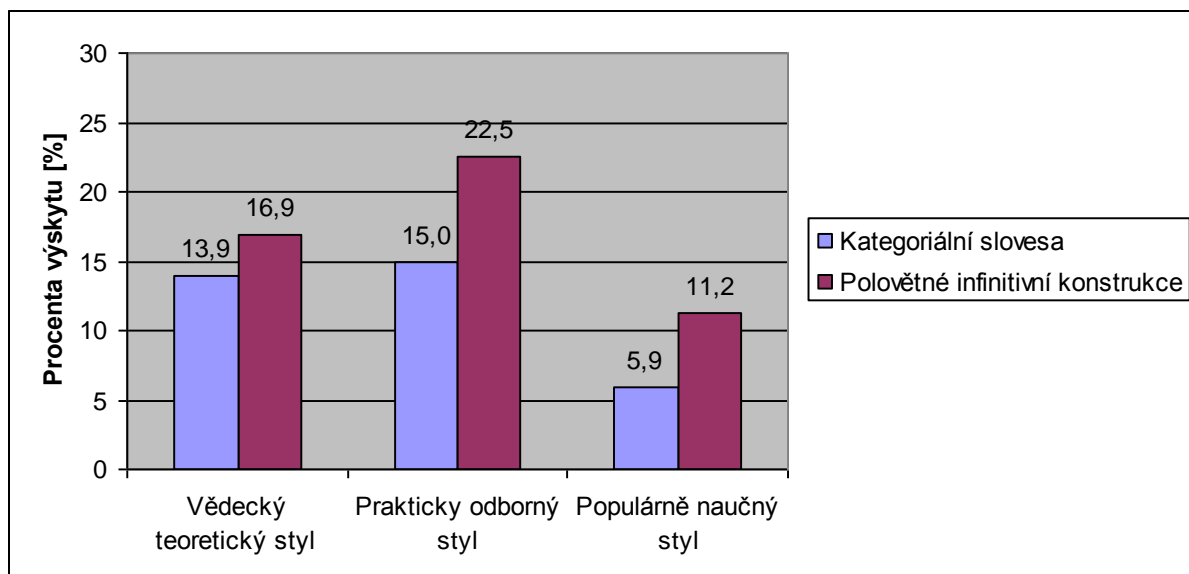
Graf 6.: Porovnání procent výskytu sledovaných slovesných jevů prostředků nominalizace vztažených na celkový počet sloves ve 3 000 slovech jednotlivých stylů (pro názornost maximum osy y zvoleno 30 %)
