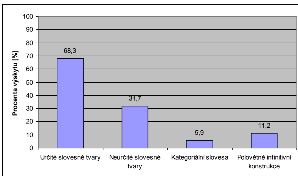
Graf 3.: Procentuální vyjádření sledovaných slovesných jevů vztahených na celkový počet sloves ve 3 000 slovech stylu populárně naučného
