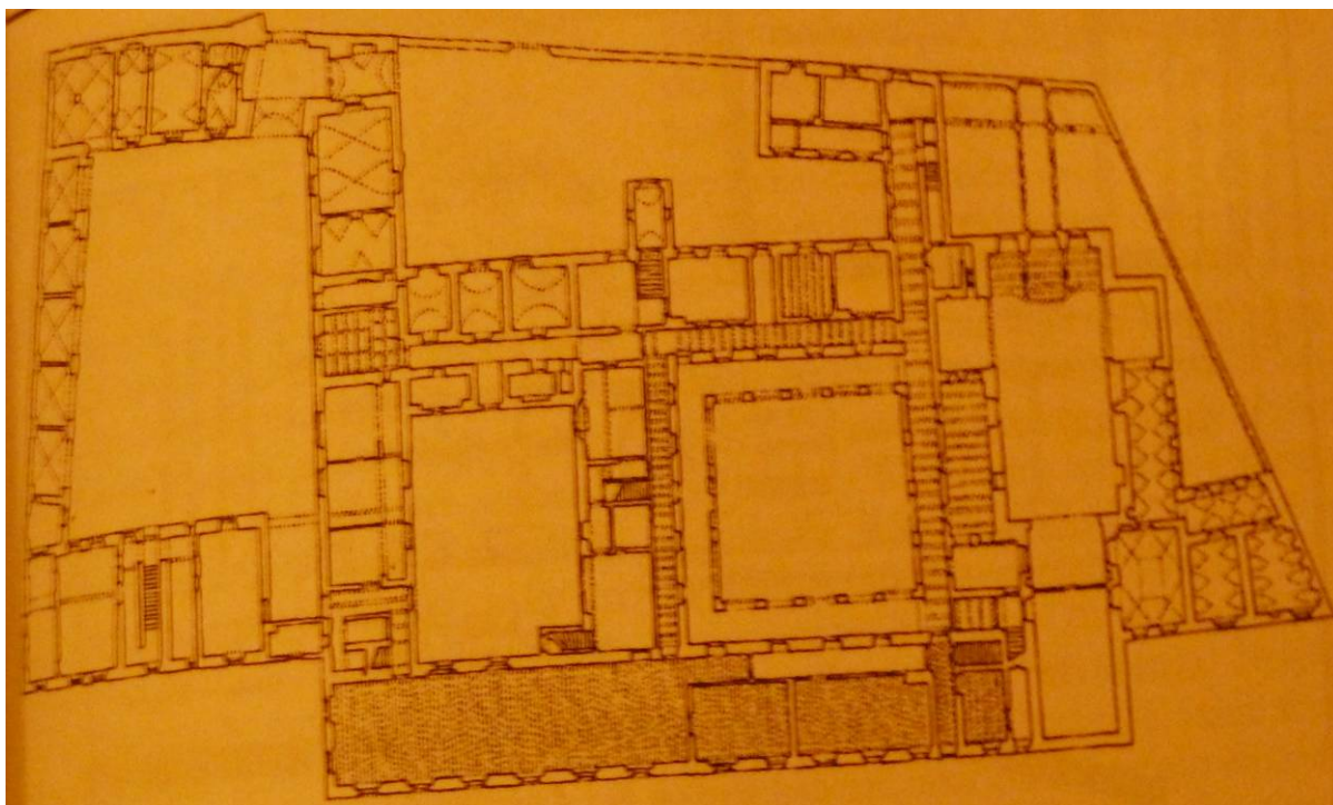
Obr. č. 14 – Půdorys přízemí hradčanského konventu, současný stav (FOLTÝN – SOMMER – VLČEK, s. 453)
