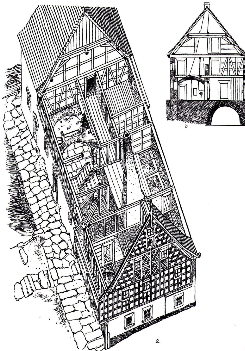
27 Chebský dům: a) Horní Lomany čp. 2, okres Cheb; b) Horní Lomany čp. 2, okres Cheb (konec 18. století), příčný řez
