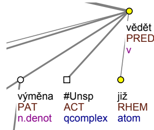
Figure 3.4: Example tectogrammatical subtree for the substring ”[...] o výměně již věděli.” (engl. ”[...] ([they] already knew about the exchange.”) to illustrate the empty functional role
