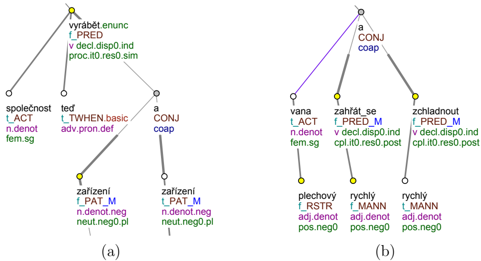
Figure 2.3: Two tectogrammatical subtrees that illustrate the effective child relation. (a): ” Společnost nyní vyrábí zařízení [...] a zařízení [...] ” (engl. ” The company now manufactures [...] equipment and [...] equipment ”) (b): ” Vana plechová se zahřeje rychle a rychle zchladne, [...] ” (engl. ” The tin bath heats up fast and cools off fast, [...] ”)
