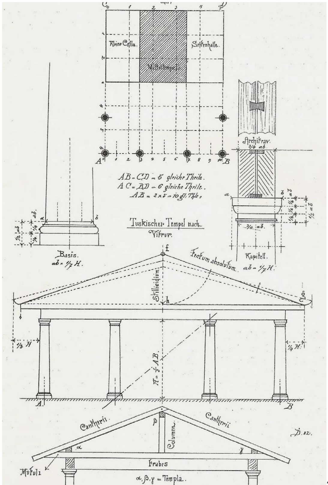
52. Tuskánský chrám dle Vitruvia, DURM 1905, s. 97, obr. 108.
