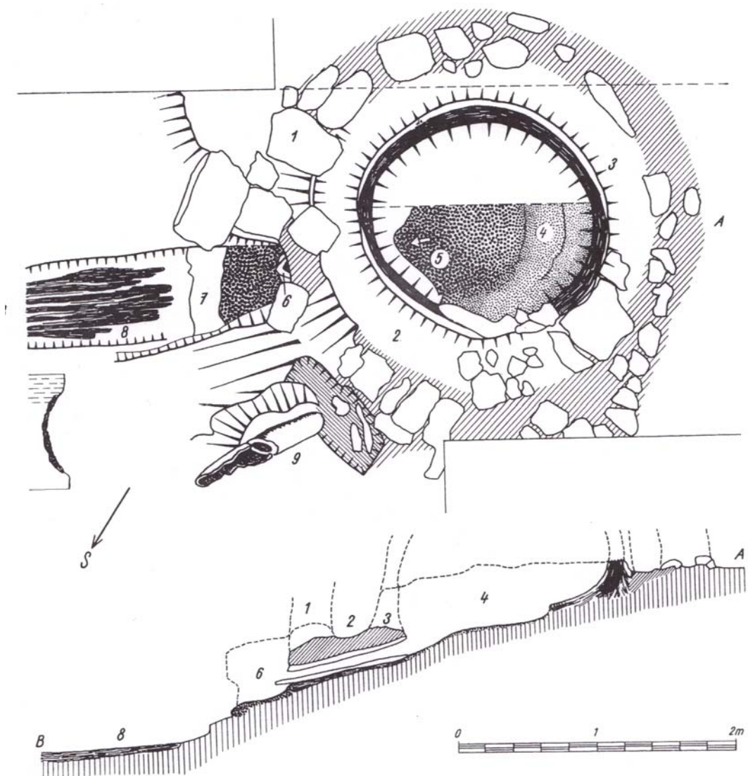
Obr. 22, Půdorys a profil destilační pece v Krásné dolině, 1-vnější kamenný plášť, 2-dno meziplášťového topeniště, 3-stěny kopule rozkladné komory, 4-dno rozkladné komory, 5-vtok do sopouchu, 6-hliněná výpustní trubka, 7-schodovitá část v hrudi pece pro záchytné misky, (podle R. Pleinera).
