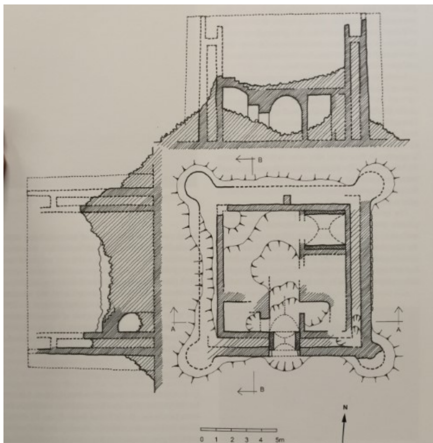
Obrázek 15: Plán a řezy pevností na lokalitě Qasr al-Sumaria, Chárga (Převzato z: Rossi, Ikram 2018).
