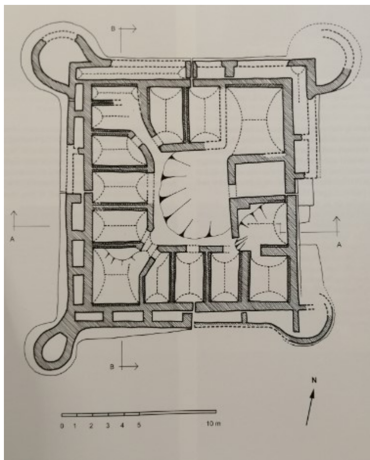
Obrázek 26: Plán pevnosti Qasr al-Labecha, Chárga (Převzato z: Rossi, Ikram 2018 ).
