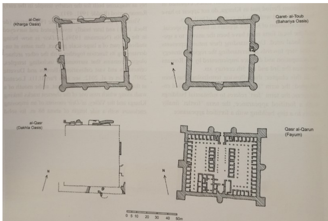
Obrázek 1: Porovnání půdorysů pevností al-Dér, Qaret al-Toub, al-Qasr a Qasr al-Qarun. (Převzato z: Rossi, Ikram 2018)
