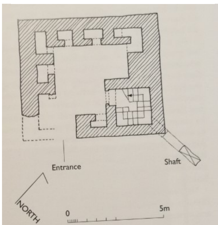
Obrázek 24: Plán strážní věže v lokalitě Umm al-Dabadíb, Chárga (Převzato z: Rossi, Ikram 2018 ).
