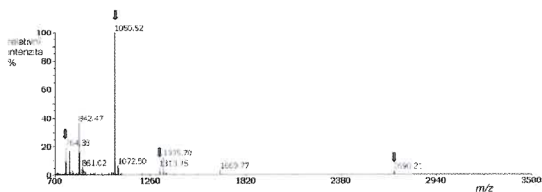
Obr. 4. Spektrum PMF neznámého proteinu po trypsinovém štěpení; spektrum bylo změněno v pozitivním reflektrotonovém módu s maticí CHCA; šipky označují peptidy, kterými byl proteom předběžně identifikován
