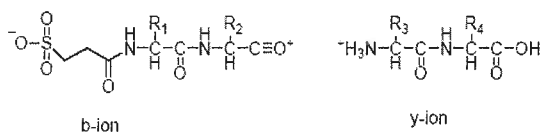
Obr. 3. Příklad fragmentace derivatizovaného tetrapeptidu; při fragmentaci vznikají výhradně b- a y-iony; díky celkovému neutrálnímu náboji není b-ion detegovatelný
