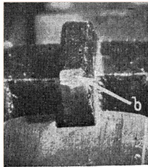
Obrázek 15: Vyhazovač nábojnic pistole: Beretta 233
