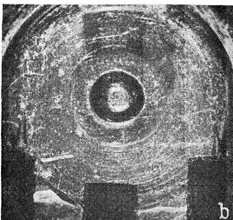
Obrázek 10: Lůžka pro dno nábojnice pistolí Beretta 228
