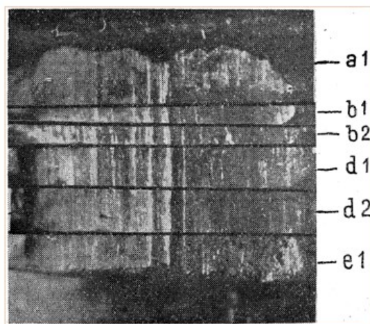
Obrázek 30: Vzájemné spojení makrofotografií sešinitých stop na obrubě dna nábojnic z předešlého snímku 249
