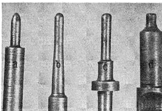
Obrázek 13: Zápalek pistolí: a) ČZ, b) Sauer, c) Walther, d) Beretta 231
