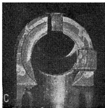
Obrázek 20: Nábojová komora pistole Sauer 238
