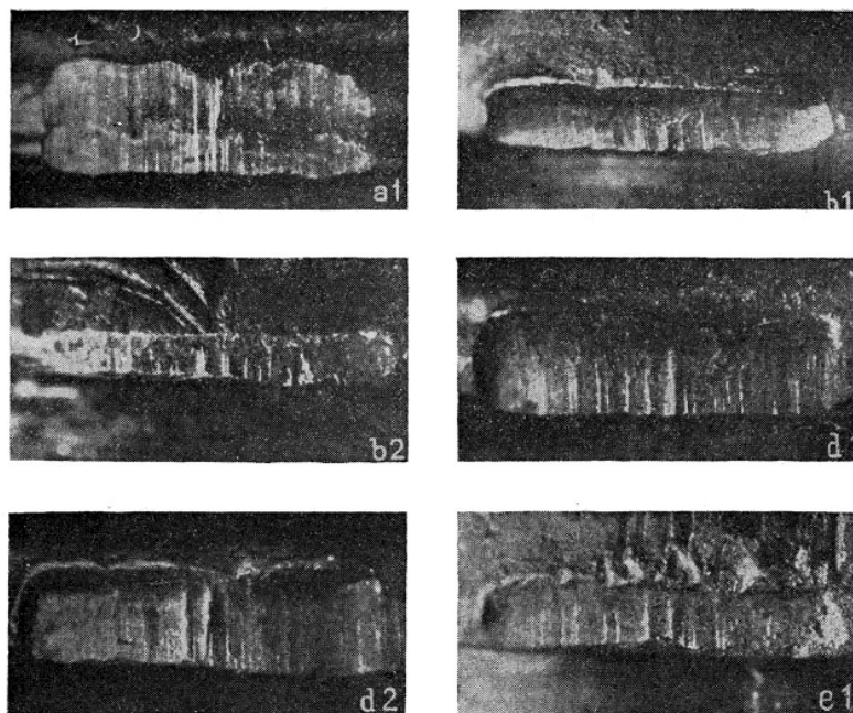
Obrázek 29: Makrofotografie sešinuté stopy na obrubě dna nábojnice 248
