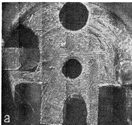
Obrázek 9: Lůžka pro dno nábojnice pistolí ČZ 227
