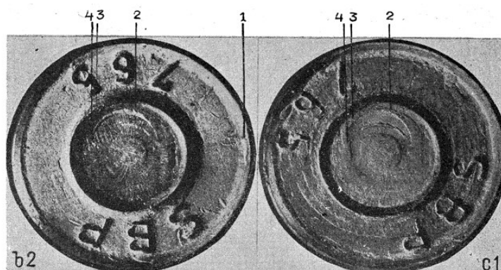
Obrázek 28: Makrofotografie dna nábojnic 247
