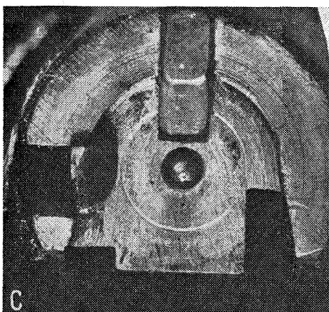
Obrázek 11: Lůžka pro dno nábojnice pistolí Sauer 229
