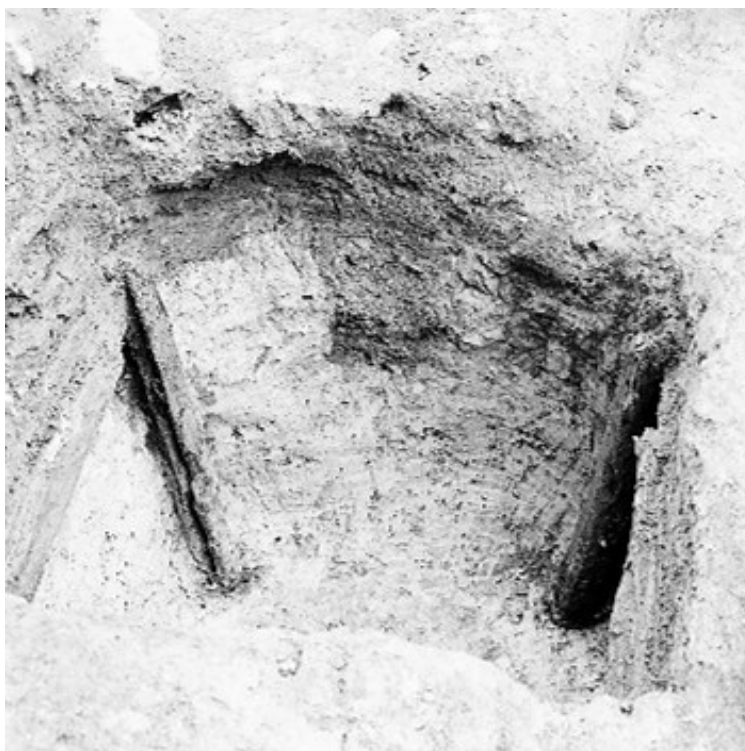
Obr. 27. Detail části výdřevy obj. 74 po rozebrání (foto 13.055). Zdroj: Velínský [1978b] .
