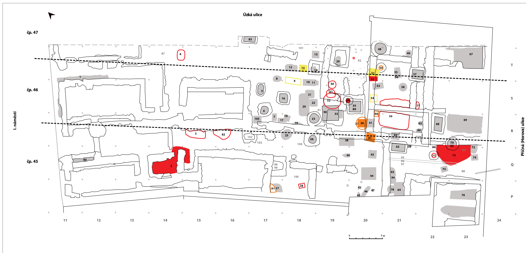
Obr. 6. Celkový plán zkoumané plochy s objekty II. fáze (plně objekty z keramické sekvence, obrysem další objekty nezařazené do sekvence), I-IIa: červená, IIb: oranžová, (IIb)IIIa: žlutá. Podle Velímský [1978b] vytvořila A. Ryšková.
