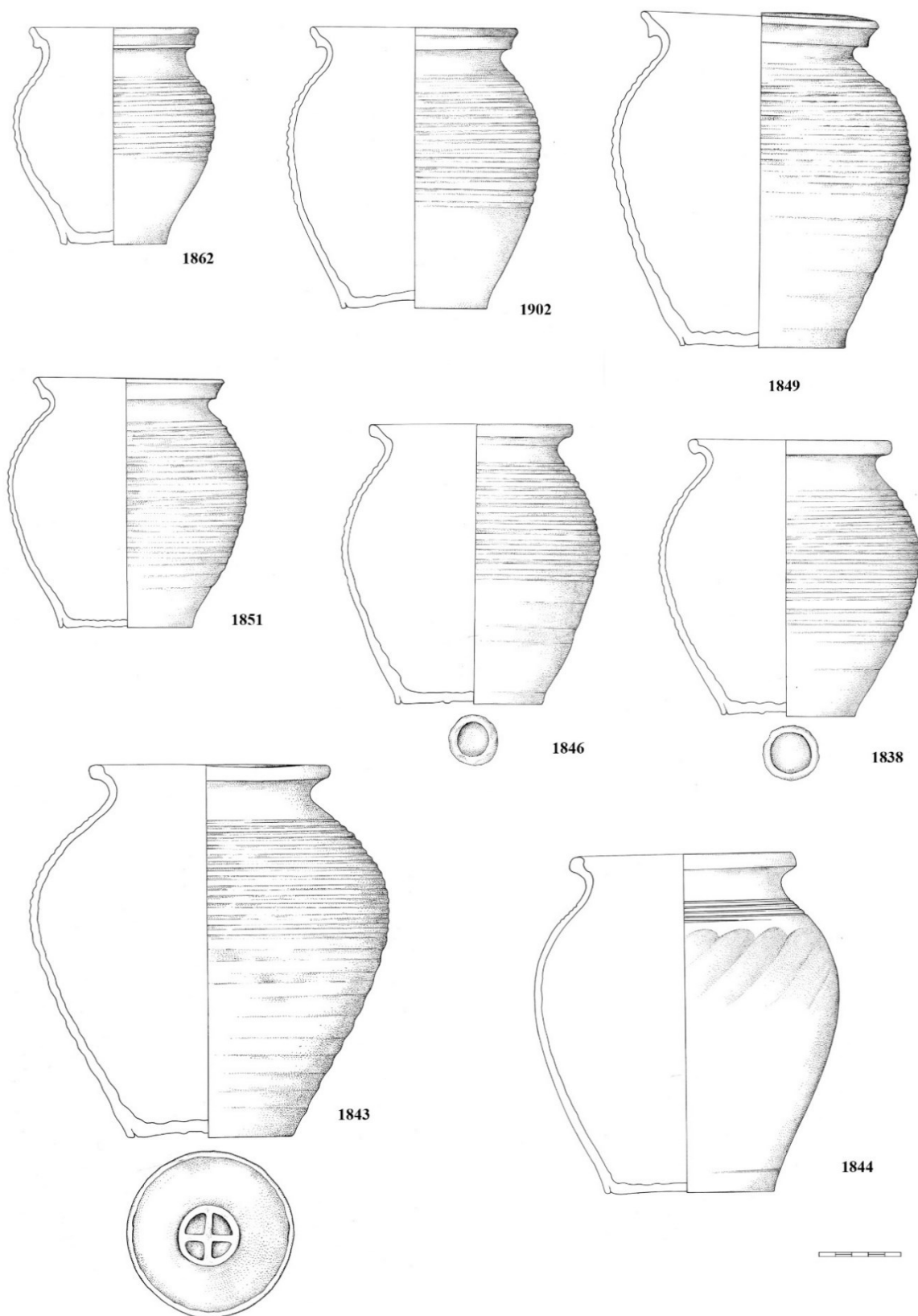
Obr. 53. Nádoby z obj. 36. Hrnc H10 : 1849, 1851, 1862, 1902. Hrnc H20 : 1838, 1843, 1844, 1846. Kresba: H. Jonášová.
