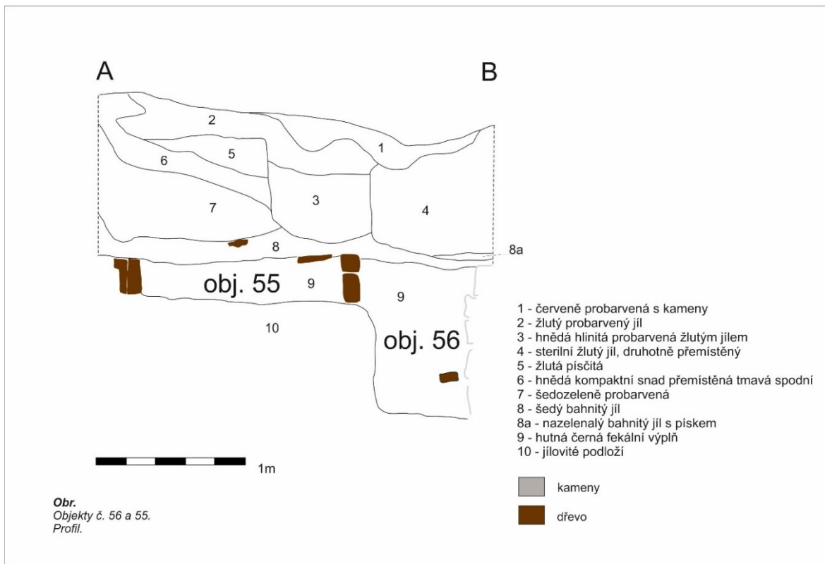
Obr. 44. Řez obj. 55 a 56. Podle Velímský [1978b] vytvořila P. Kabeláčová.
