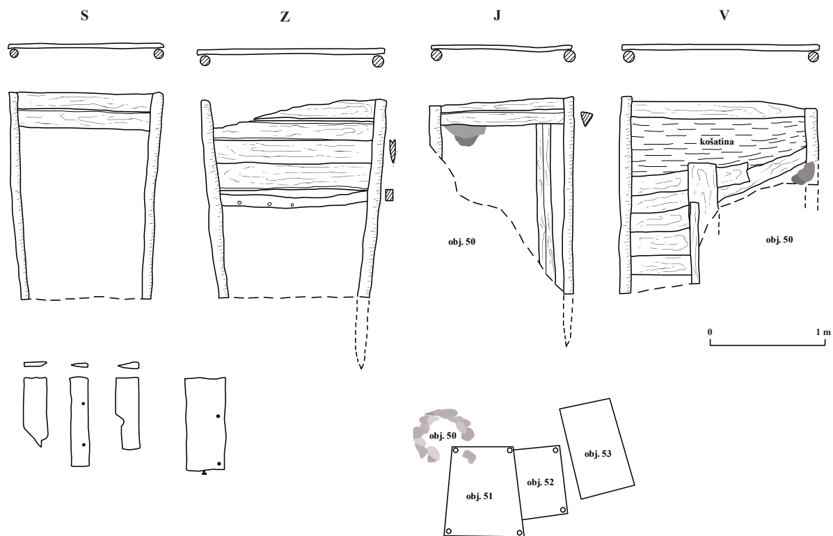
Obr. 39. Vydřeva obj. 51. Druhotně využitě dřevo (vlevo dole). Schematické zobrazení vztahu objektů 50 až 53 (vpravo dole). Podle Velímský [1978b] vytvořila A. Ryšková.
