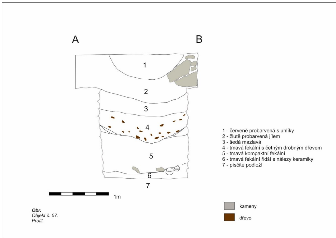
Obr. 45. Řez obj. 57. Podle Velímský [1978b] vytvořila P. Kabeláčová.
