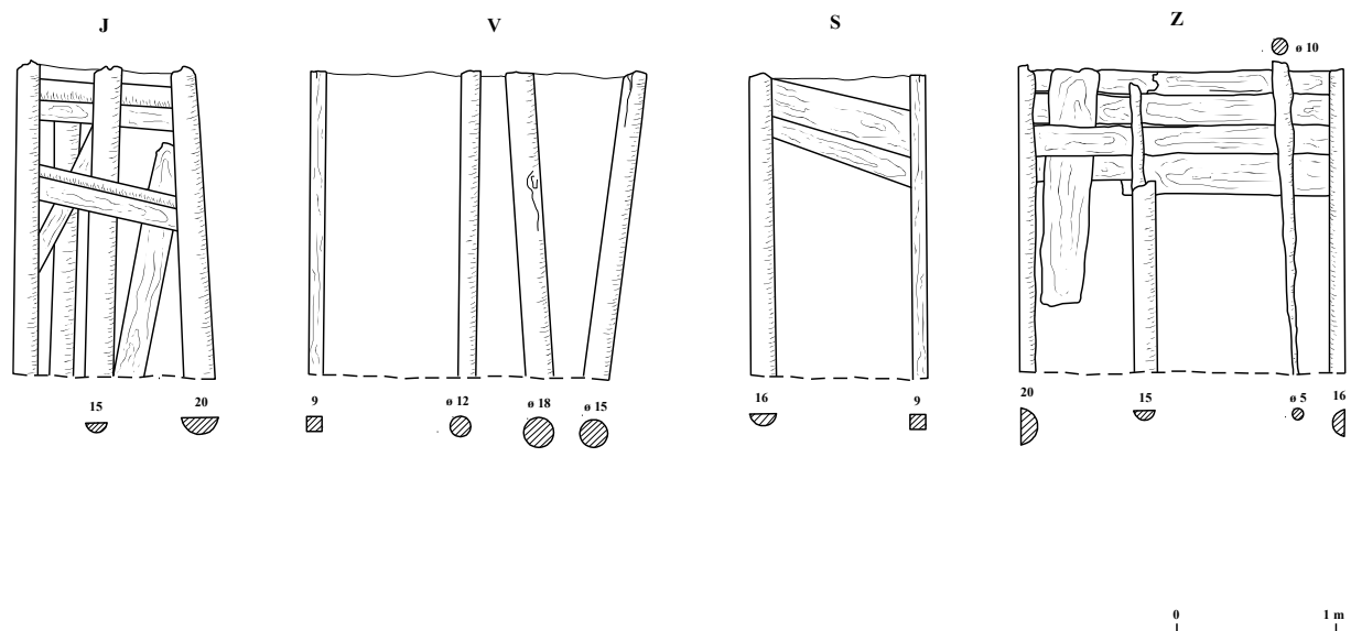
Obr. 36. Vřdřeva obj. 12. Podle Velímský [1978b] vytvořila A. Ryšková.
