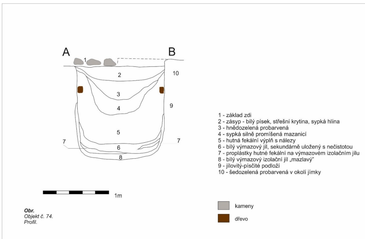
Obr. 47. Řez obj. 74. Podle Velímský [1978b] vytvořila P. Kabeláčová.
