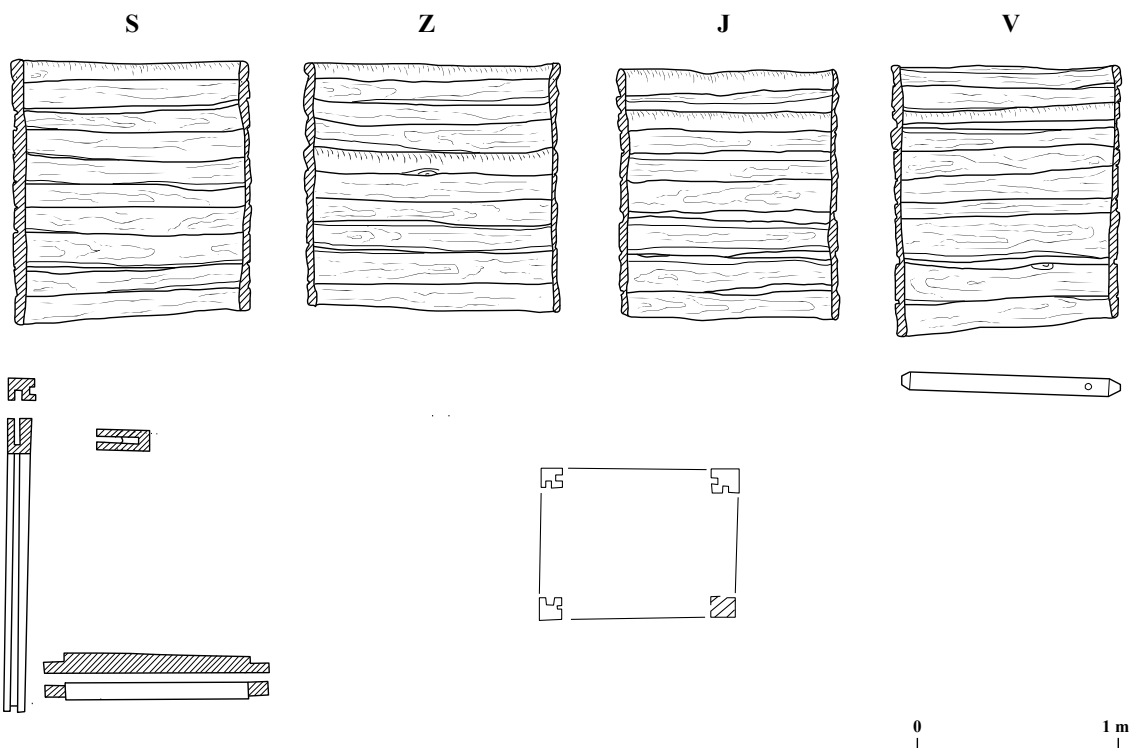
Obr. 40. Výchřeva obj. 54. Podle Velímský [1978b] vytvořila A. Ryšková.
