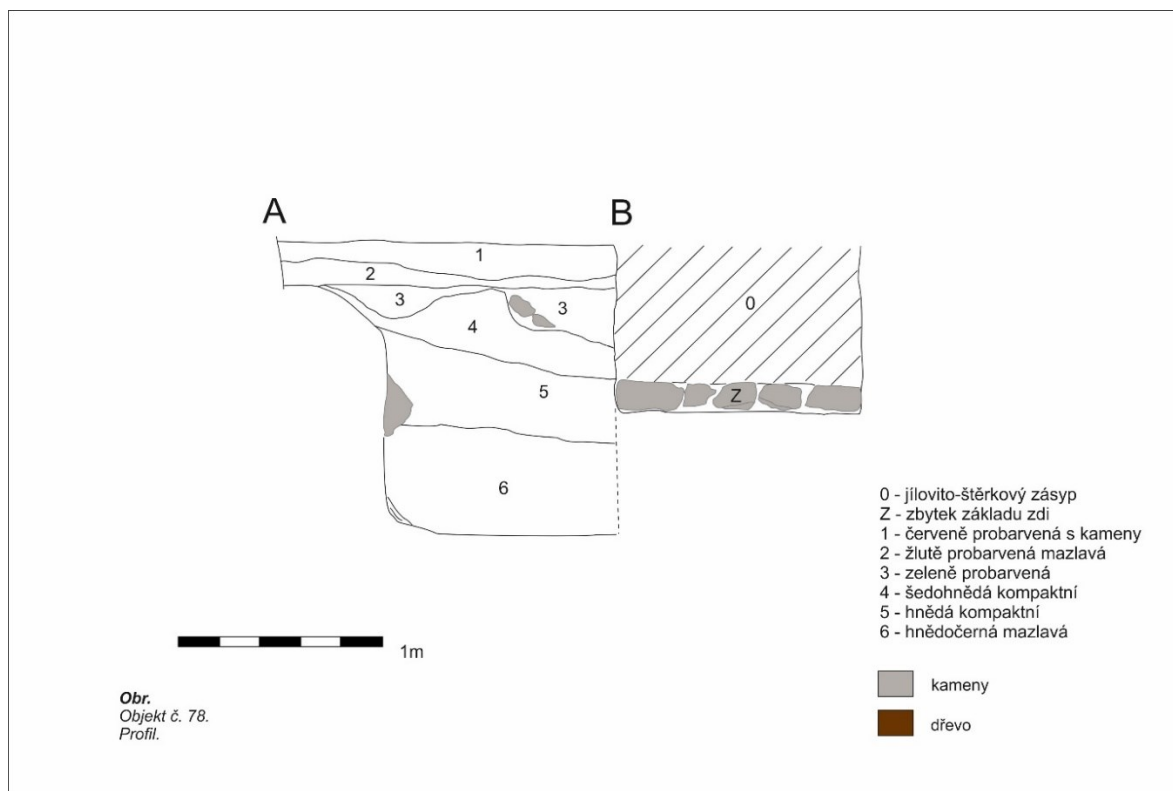
Obr. 48. Řez obj. 78. Podle Velímský [1978b] vytvořila P. Kabeláčová.
