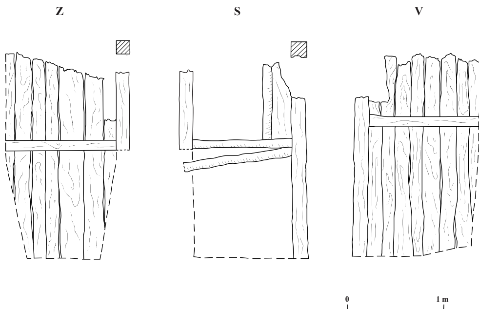
Obr. 38. Vydřeva obj. 43. Podle Velímský [1978b] vytvořila A. Ryšková.
