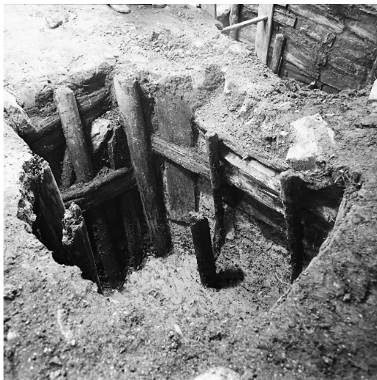
Obr. 15. Obj. 12, severní a západní stěna (foto 13.490). Zdroj: Velímský [1978b] .
