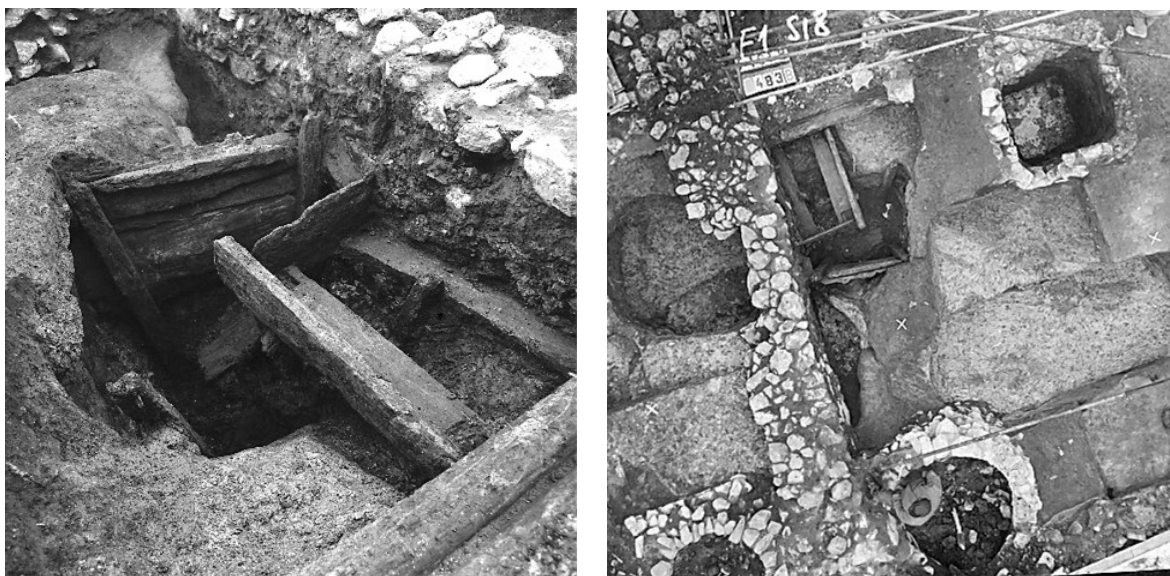
Obr. 17. Obj. 17 a 18 (foto 13.500). Superpozice obj. 17 a 18, vpravo studna č. 16, vlevo jáma č. 25, v dolní části studny č. 23 a 26 (fotogrammetrie snímek č. 483) Zdroj: Velímský [1978b] .
