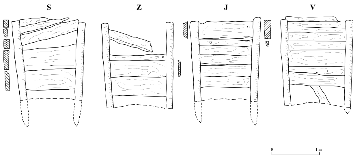
Obr. 37. Vřdřeva obj. 36. Podle Velímský [1978b] vytvořila A. Ryšková.
