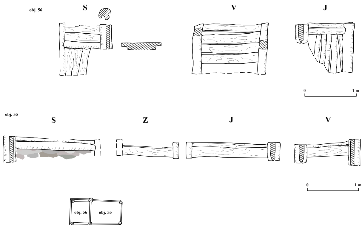
Obr. 41. Výchřeva obj. 55 a 56 a schematické zobrazení vztahu objektů 55 a 56. Podle Velímský [1978b] vytvořila A. Ryšková.
