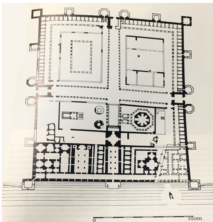
Obr. 50: Plán Diocletianova paláce ve Splitu (podle Ward-Perkins 1970, fig. 308).
