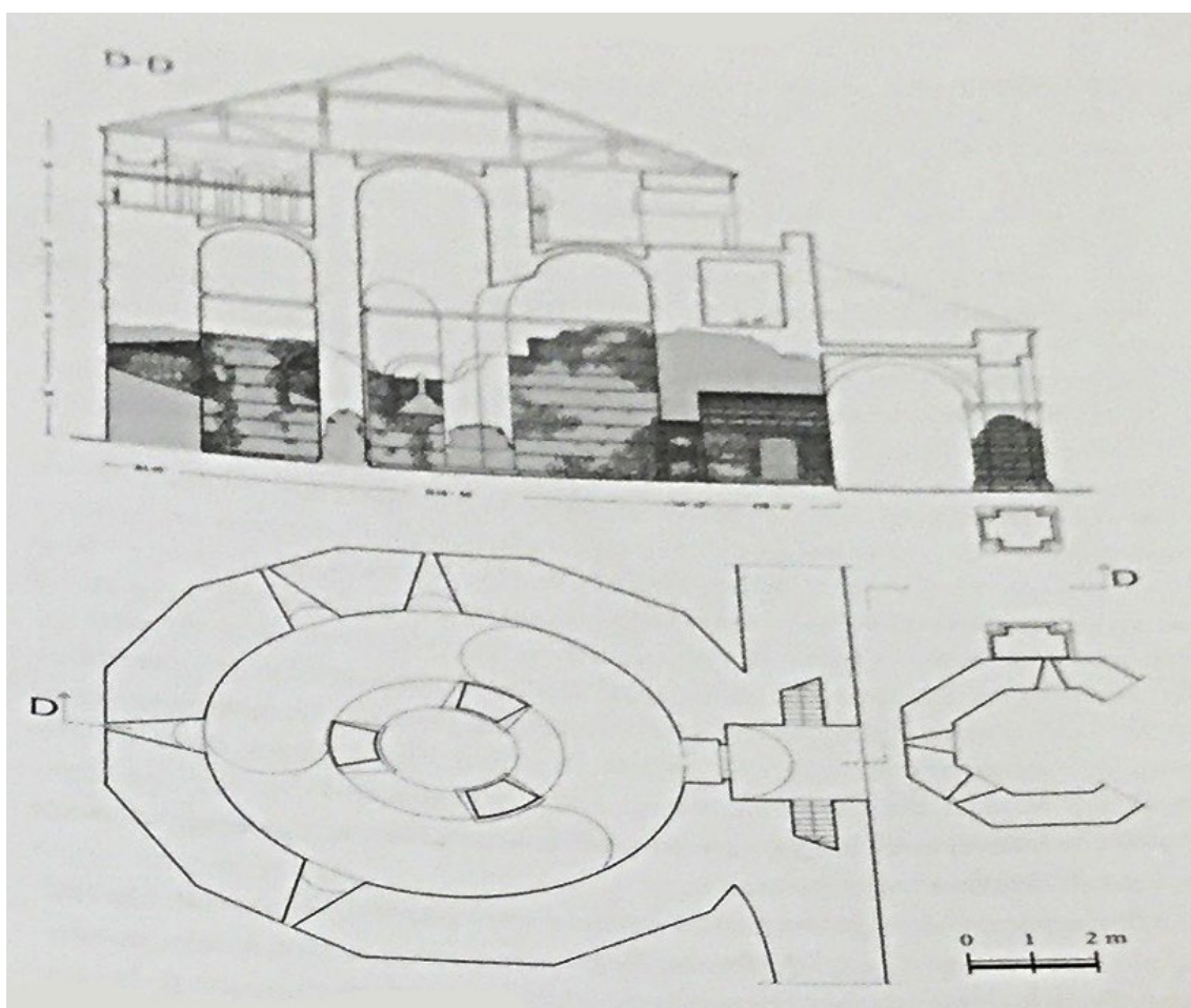
Obr. 12: Strážní věž pozdního opevnění (horní část: návrh možné rekonstrukce; dolní část: půdorys věže) (podle Popović 2011, pl. XIV).
