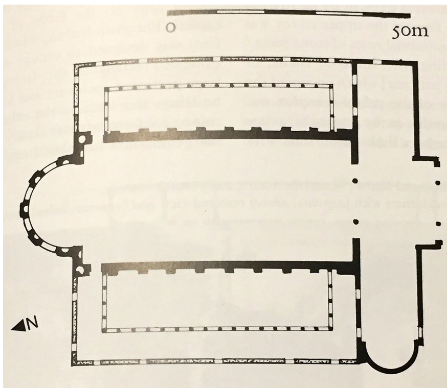
Obr. 49: Půdorys baziliky v Trieru (podle Ward-Perkins 1970, fig. 299).
