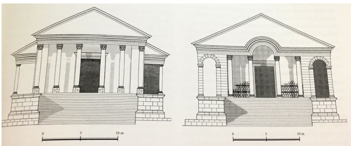
Obr. 28: Druhá varianta rekonstrukce Velkého chrámu (podle Popović 2011, pl. XXX).
