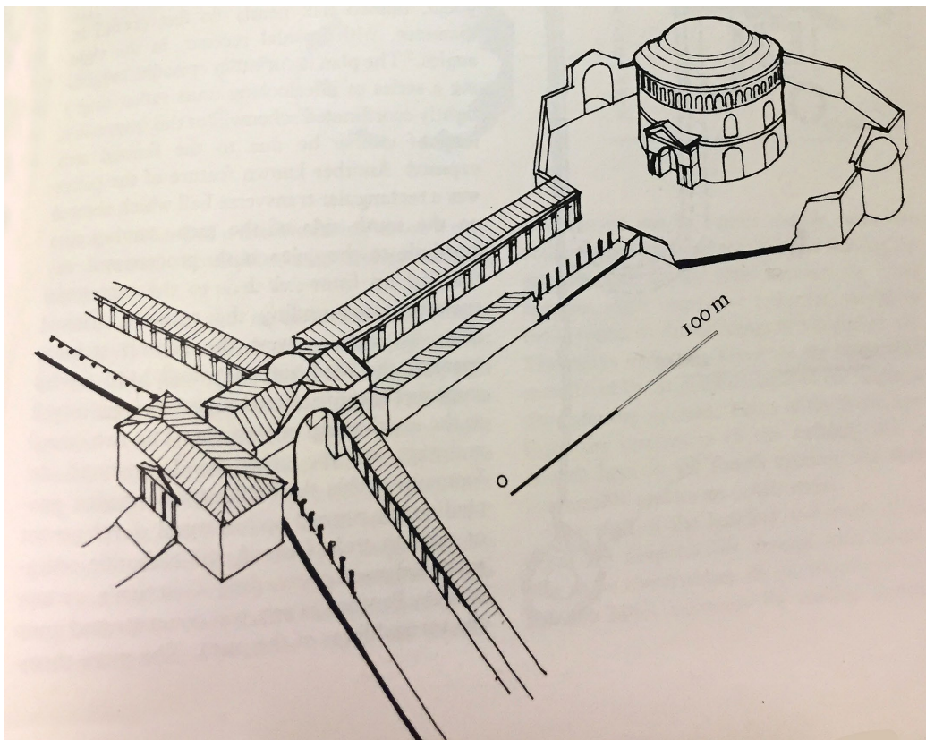
Obr. 47: Nákres kolonády, Galeriova triumfálního oblouku a Galeriova mauzolea v Thessaloníce (podle Ward-Perkins 1970, fig. 304).
