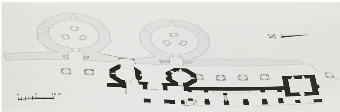
Obr. 7: Plán porovnávající rané a pozdní opevnění západní brány Felix Romuliany (podle Popović 2011, pl. VII).
