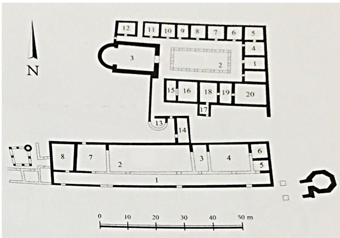
Obr. 22: Plán Paláce 2 (podle Popović 2011, pl. XXXIX).
