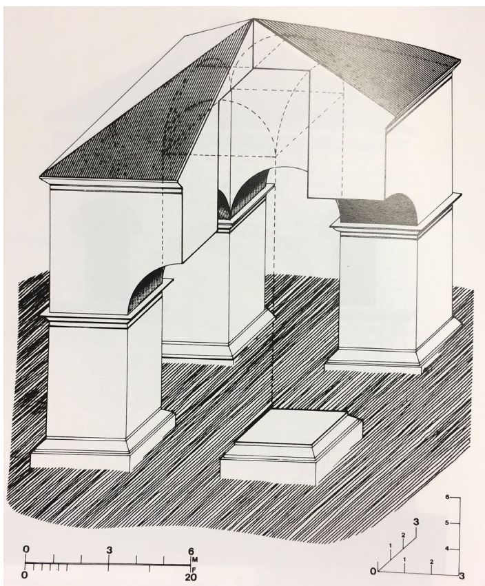
Obr. 45: Krypta pod Mauzoleem 2 (podle Srejšović – Vasić 1993, fig. 58).
