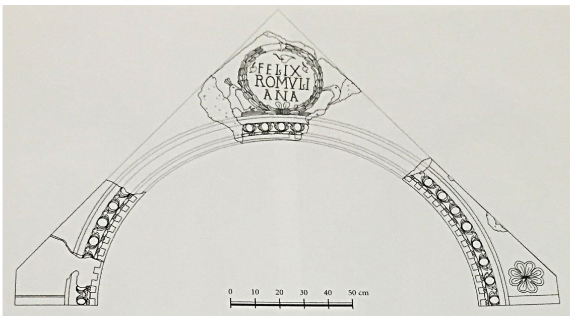
Obr. 14: Návrh rekonstrukce archivolty z galerie západní brány pozdního opevnění (podle Popović 2011, pl. XVI).
