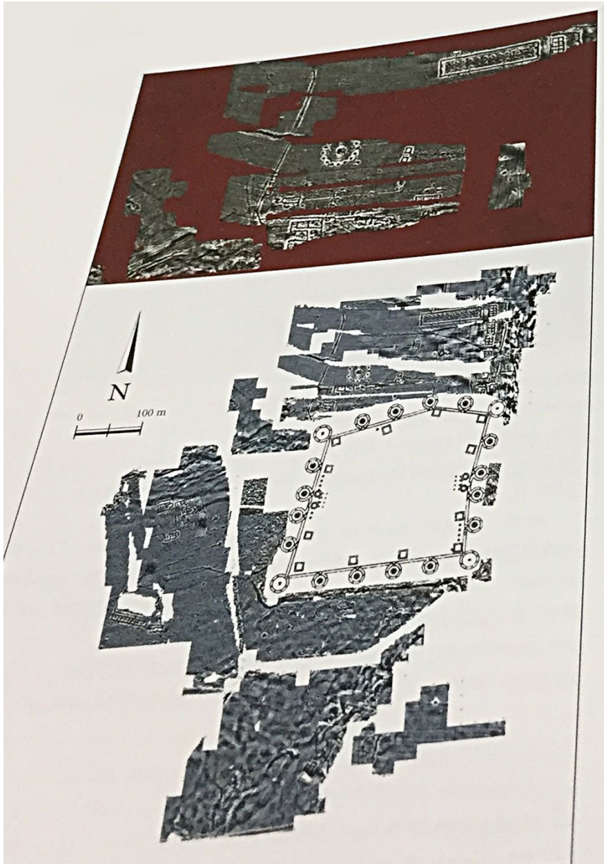
Obr. 4: Geofyzikální prospekce v okolí Felix Romuliany (podle Popović 2011, pl. IV).
