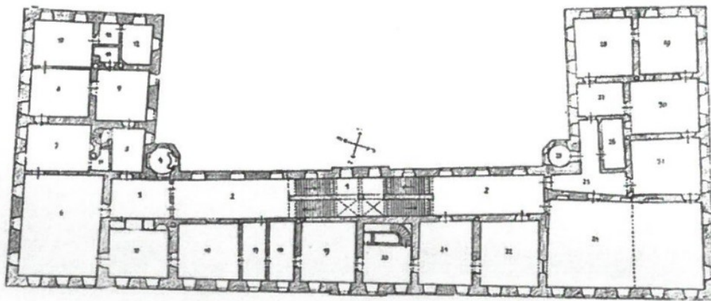
Obr. 196. Hradiště M.n. Zámek. Půdorys přízemku (nahore) a 1. patra (dole). Vue en plan du rez-de-chaussée et du 1er étage.
