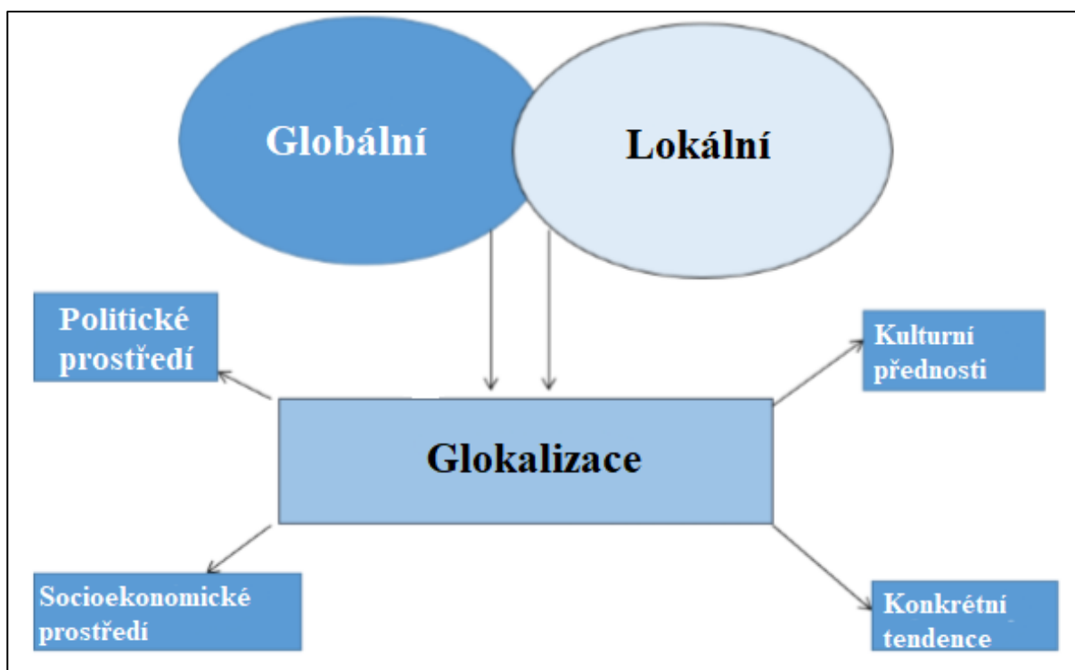
Obrázek 1 - Glocalizační rozhraní
