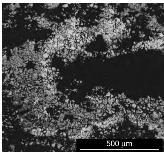
Obr. 7 Struktura kovu fragmentu B – výrazné korozní napadení po hranicích zrn kovu s absencí materiálu ve střední části vzorku (foto z metalografického mikroskopu Olympus PME 3 J. Kmošek)
