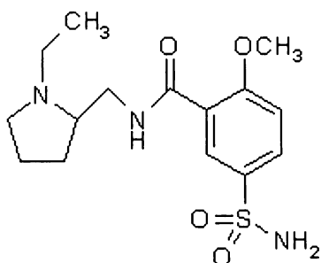
Obr. 4. Strukturální vzorec sulpiridu
