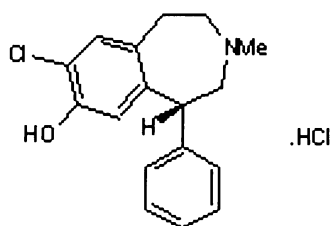
Obr. 3. Strukturní vzorec SCH23390
