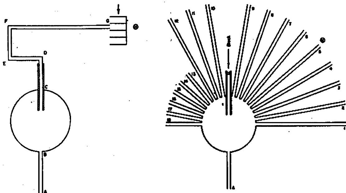
Obr. 1. Tolmanovo bludiště. Převzato z Tolman E. C. (1948), Cognitive maps in rats and men , Psychol. Rev. , 55: 189-208. Obrázek nalevo ukazuje jednoduché bludiště. Potkan měl za úkol běžet z místa A do místa G, kde našel potravu. H značí světlo. Po čtyřech nocích, každou noc se prováděly tři pokusy, ve kterých se potkan naučil bez váhání projít cestu z A do G, bylo toto bludiště vyměněno za paprskovité (obrázek napravo). Potkani byli opět položeni na centrální základnu, odkud měli jít na konec každého z ramen, kde na ně čekala odměna. Optimálním řešením pro potkany bylo navštívit všechna ramena a vyhnout se návratu do již navštíveného ramene.
