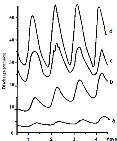
Obrázek 6. Vývoj denní amplitudy průtoku na toku napájeného tavnou vodou z ledovce. Sledované období: a) 17.-20. 5. b) 14.-17.6. c) 23.-26.6. d) 19.-22.7. Zdroj: Hubbard a Glasser, 2005
