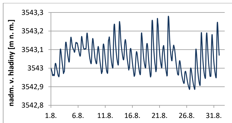
Obrázek 57. Denní kolísání hladiny jezera Adygine v srpnu roku 2010.
