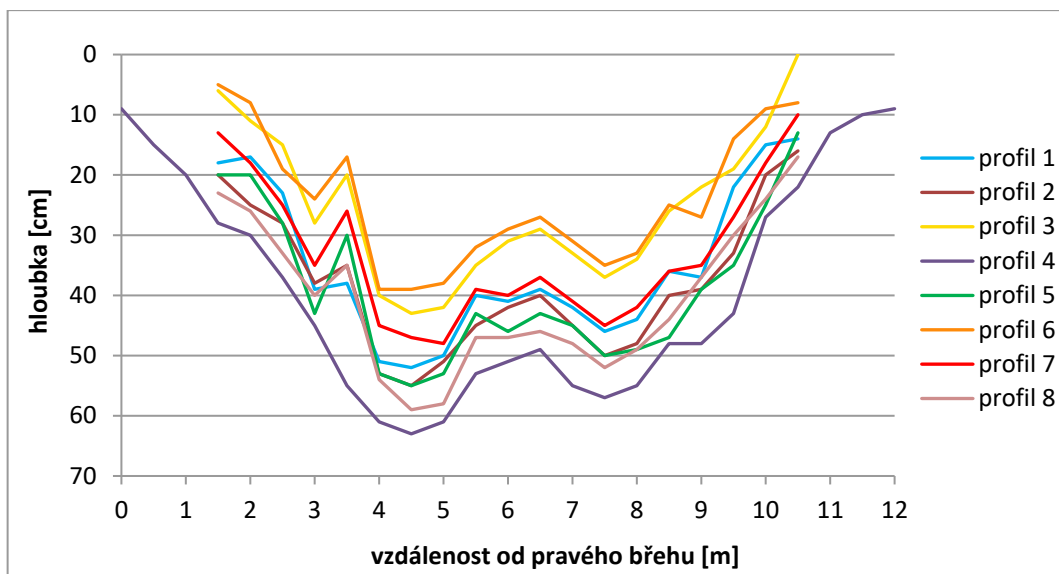
Obrázek 49. Příčné profily výtoku z jezera při různých vodních stavech. Profil 1 – 3.8. 15:30-16:00; profil 2 – 3.8. 17:45-18:05; profil 3 – 4.8. 8:00-8:15; profil 4 – 4.8. 17:20-17:40; profil 5 – 4.8. 20:10-20:35; profil 6 – 5.8. 10:10-10:30; profil 7 – 5.8. 13:50-14:10; profil 8 – 5.8. 15:00-15:15.
