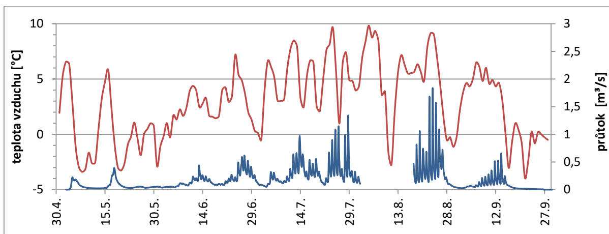
Obrázek 62. Průběh průtoku (modře) na odtoku z jezera Adygine a teploty vzduchu (červeně) v ablační sezóně roku 2011.
