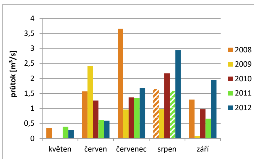
Obrázek 64. Maximální měsíční průtoky na odtoku z jezera Adyginé.
