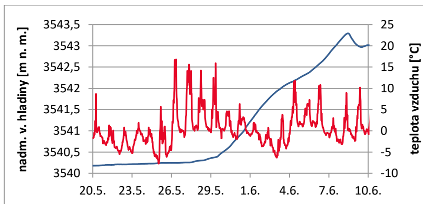
Obrázek 54. Průběh teplot vzduchu z horní meteostanice a úrovně hladiny v období plnění jezera Adygine v roce 2009. Teplota červeně, úroveň hladiny modře.
