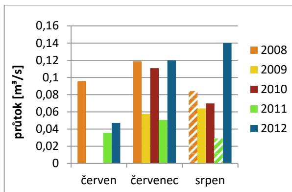
Obrázek 65. Minimální měsíční průtoky na odtoku z jezera Adygiene.
