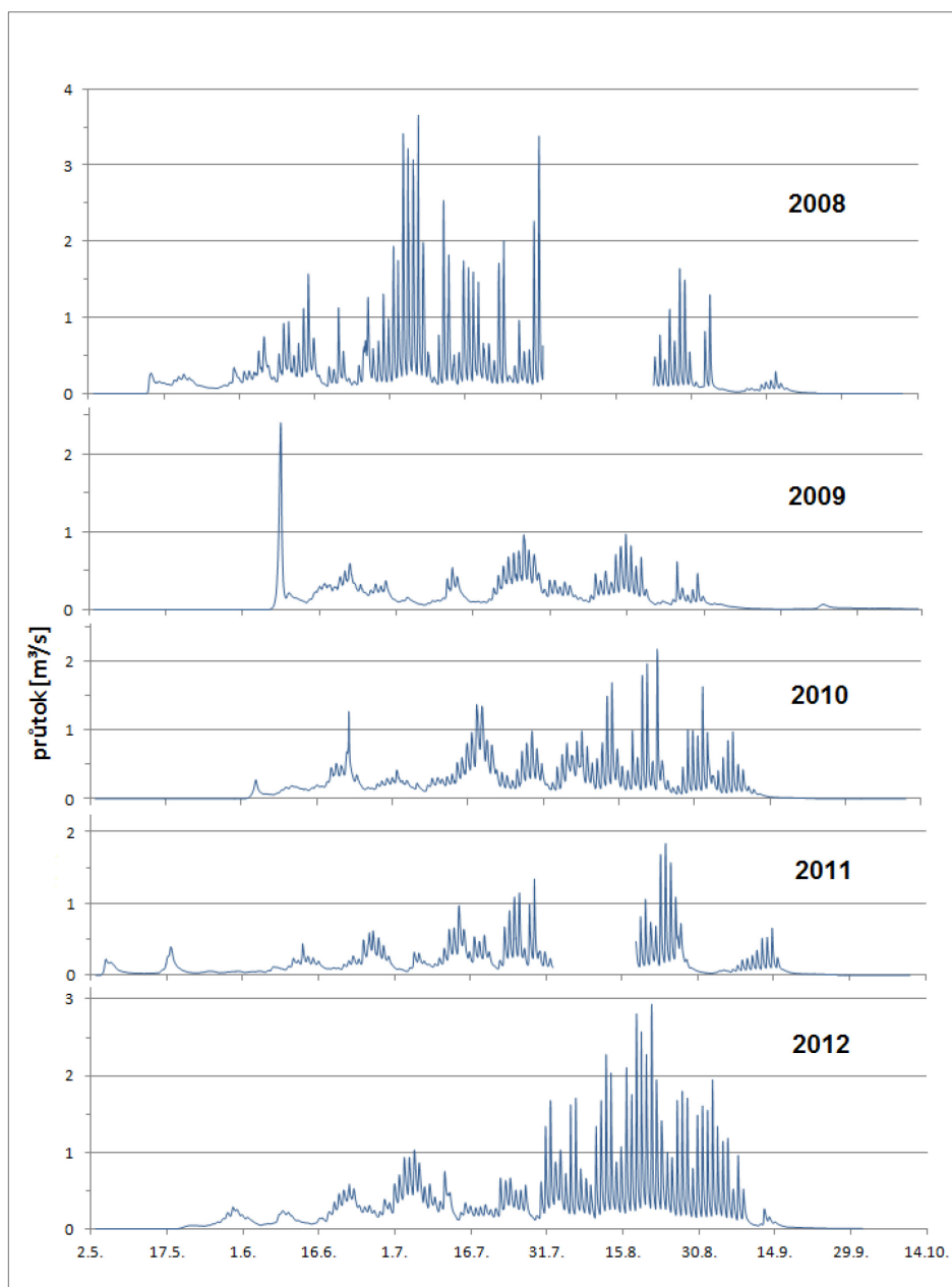
Obrázek 61. Průtoky na odtoku z jezera Adygině v ablační sezóně, roky 2008-2012.
