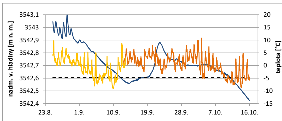
Obrázek 53. Vývoj úrovně hladiny jezera a teploty vzduchu na podzim roku 2009. Žlutá – horní meteostanice, oranžová – dolní meteostanice, čárkovaně – úroveň povrchového odtoku.
