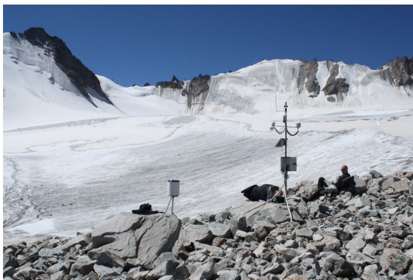
Obrázek 45. Horní meteorologická stanice na lokalitě Adygine ve výšce 3800 m n. m.
