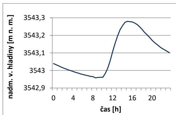
Obrázek 56. Denní kolísání hladiny jezera Adygine dne 22. srpna 2010.
