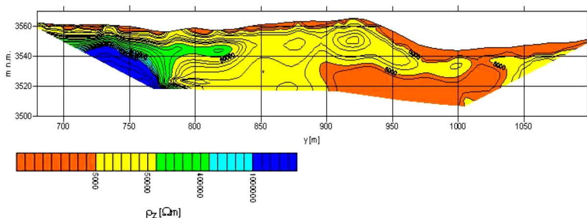
Obrázek 37. Podélný profil hrází jezera Adygine Horní – odporová měření. Zdroj: Černý et al., 2010. Oranžová – sutě, pevné horniny, místy zvlhčené; žlutá – sutě, pevné horniny, místy promrzlé; zelená – promrzlé horniny, místy zbytky ledovce; sv. modrá – ledovec, místy s morénovým materiálem; tm. modrá – ledovec.
