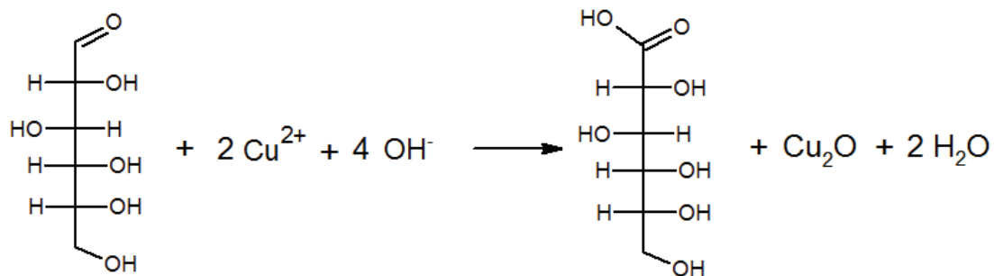
Obr. 34 - Chemická rovnice Fehlingovy zkoušky
