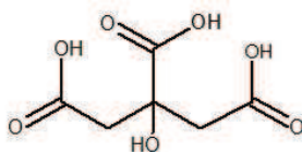
Obr. 56 - struktura citronové kyseliny
