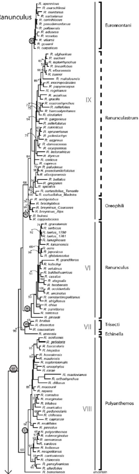
Příloha 1 – Fylogram vymezující lakušníky jako sekci Batrachium v rámci rodu Ranunculus . Převzato (Hörandl & Emadzade, 2012).
