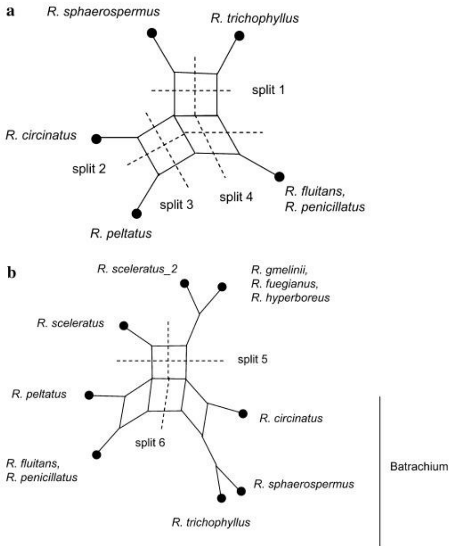
Příloha 2 – a) Diagram vytvořený metodou „split decomposition“ demonstrující retikulární vztahy v rámci sekce Batrachium , b) Diagram vytvořený metodou „split decomposition“ demonstrující retikulární vztahy sekce Batrachium s příbuznými sekcemi Hecatonia a Xenthobatrachium . Převzato (Hörandl et al., 2005).
