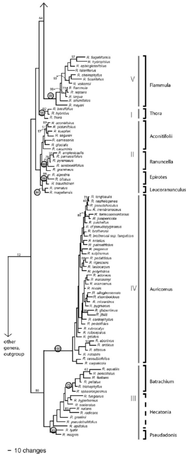
Příloha 1 – Fylogram vymezující lakušníky jako sekci Batrachium v rámci rodu Ranunculus . Převzato (Hörandl & Emadzade, 2012).
