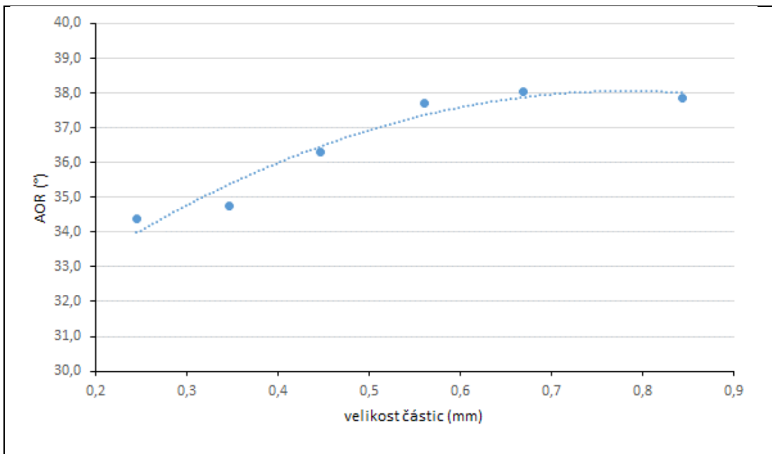
Obr. 3 Závislost úhlu sypání (AOR) na velikosti částic pro granulát sorbitolu s přísávkem 0,5 % steáranu hořečnatého (St).
