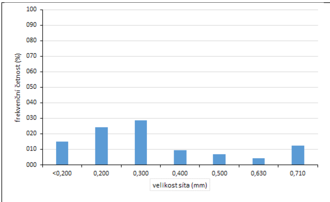
Obr. 1 Histogram čítnosti částic granulátu sorbitolu
