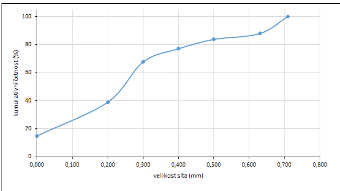
Obr. 2 Kumulativní čítnost částic granulátu sorbitolu
