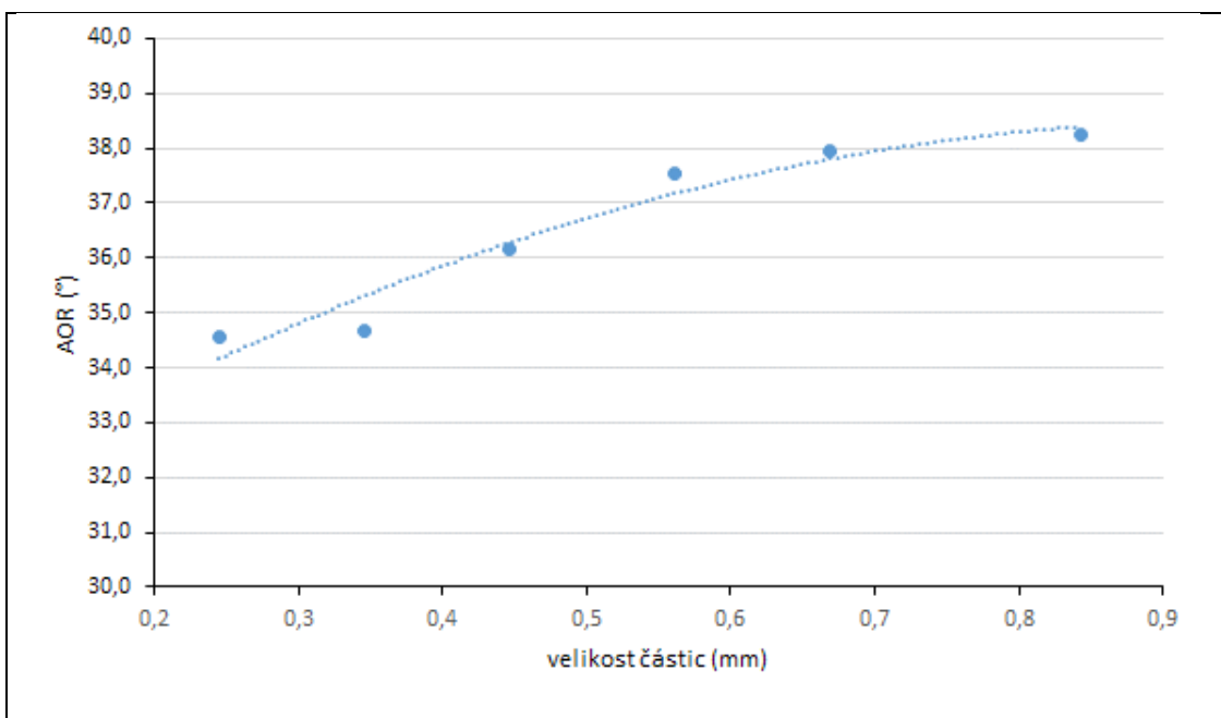
Obr. 4 Závislost úhlu sypání (AOR) na velikosti částic pro granulát sorbitolu s přísávkem 1,0 % steáranu hořečnatého (St).
