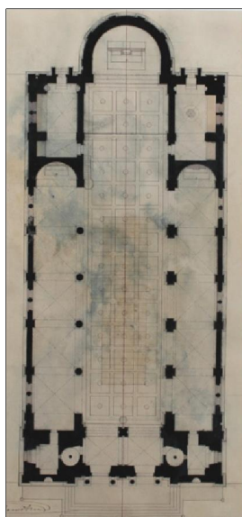
83. A. V. Barvítius: Návrh kostela sv. Václava na Smíchov , p dorys A´ XI, 1879, detail, kolorovaná kresba, 44x29, NTM, AAS, Fond . 3 ó Barvítius Antonín Viktor, desky . 20080603/07.
