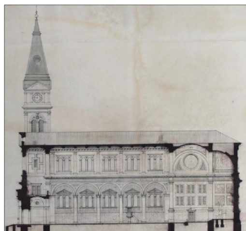
76. A. V. Barvitijs, I. Ullmann: Návrh kostela sv. Václava na Smíchov , bo ní pohled B 0 IV, 1879, detail, ernobílá kresba, 42,5x48,5, NTM, AAS, Fond. . 3 ó Barvitijs Antonín Viktor, desky . 20100809/01.
