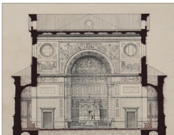
58. I. Ullmann: Návrh kostela sv. Václava na Smíchov , p í ný ez v úrovni transeptu, B V, 1878, detail, kolorovaná kresba, 29x42, NTM, AAS, Fond. . 3 ó Barvitius Antonín Viktor, desky . 20061027/01.
