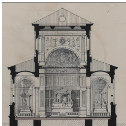
72. A. V. Barvitius: Návrh kostela sv. Václava na Smíchov , p í ný ez, 1878, detail, ernobílá kresba, 29x40, NTM, AAS, Fond. . 3 ó Barvitius Antonín Viktor, desky . 20080603/09.
