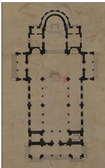
8. J. Schulz: Vít zný sout flní návrh kostela sv. Václava na Smíchov , p dorys, 1872, detail, ernobílá kresba, papír na kartonu, 40,5x56, NTM, AAS, Fond. . 46 ó Schulz Josef, desky . 20041104/04.
