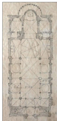
34. P. Sprenger, J. G. Müller: Kostel Altlerchenfeld, Víde , 184861862, t í tvrte ní pohled.
