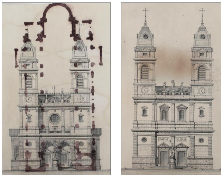
68. A. V. Barvitius: Návrh kostela sv. Václava na Smíchov , pohled na průčelí, 1878, detail, černobílá kresba, 42x29, NTM, AAS, Fond. . 3 ó Barvitius Antonín Viktor, desky . 20080603/09.
