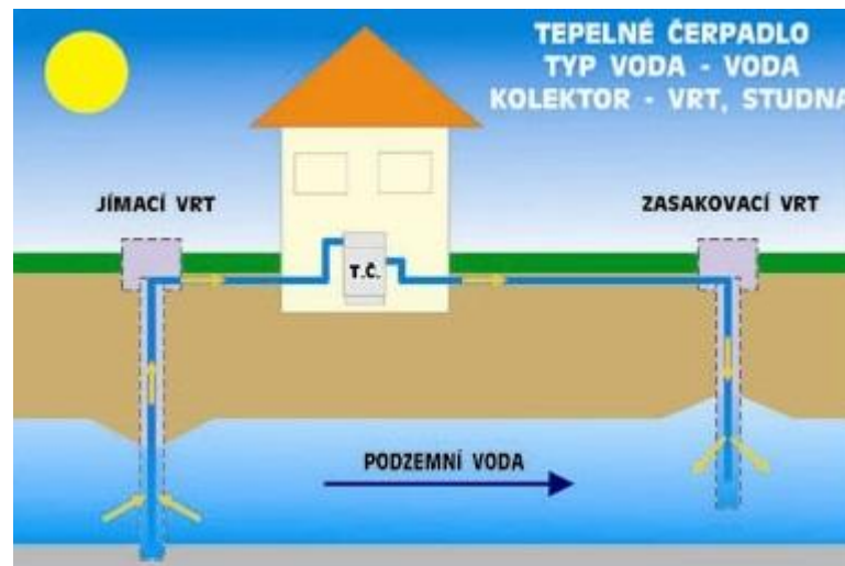
Obrázek 4.1: Řešení vytápění a ohřevu TUV pro observatoř Doksany
