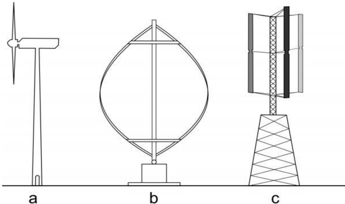
a) větrná elektrárna s horizontální osou, b) větrná elektrárna Darrieus, c) větrná elektrárna Giromill
