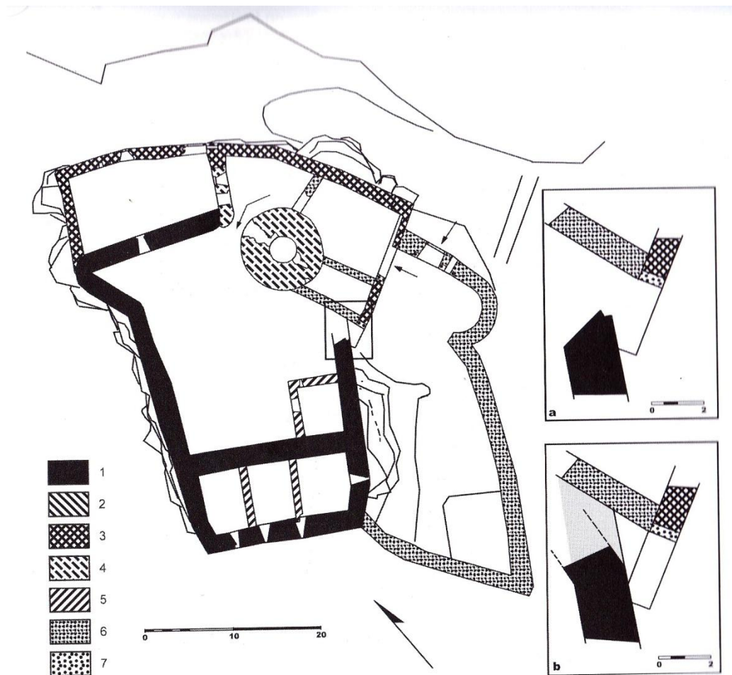
Obr. 7: Hrad Valdek. Půdorys hradu s vyhodnocením stáří zdiva – současný stav: 1 – první stavební etapa – 13. století; 2 – hypotetické nejstarší zdivo 13. století; 3 – druhá stavební etapa – 13. století; 4 – třetí stavební etapa – počátek 14. století; 5 – zdivo z druhé poloviny 14. století nebo počátku 15. století; 6 – pozdně gotické zdivo z 15. století; 7 – zdivo 19. a 20. století; detail a – současná nálezová situace nejstarší brány; b – zakreslení téže situace podle J. Muka v roce 1976, šedě je vybarveno stratigraficky nejmladší zdivo
