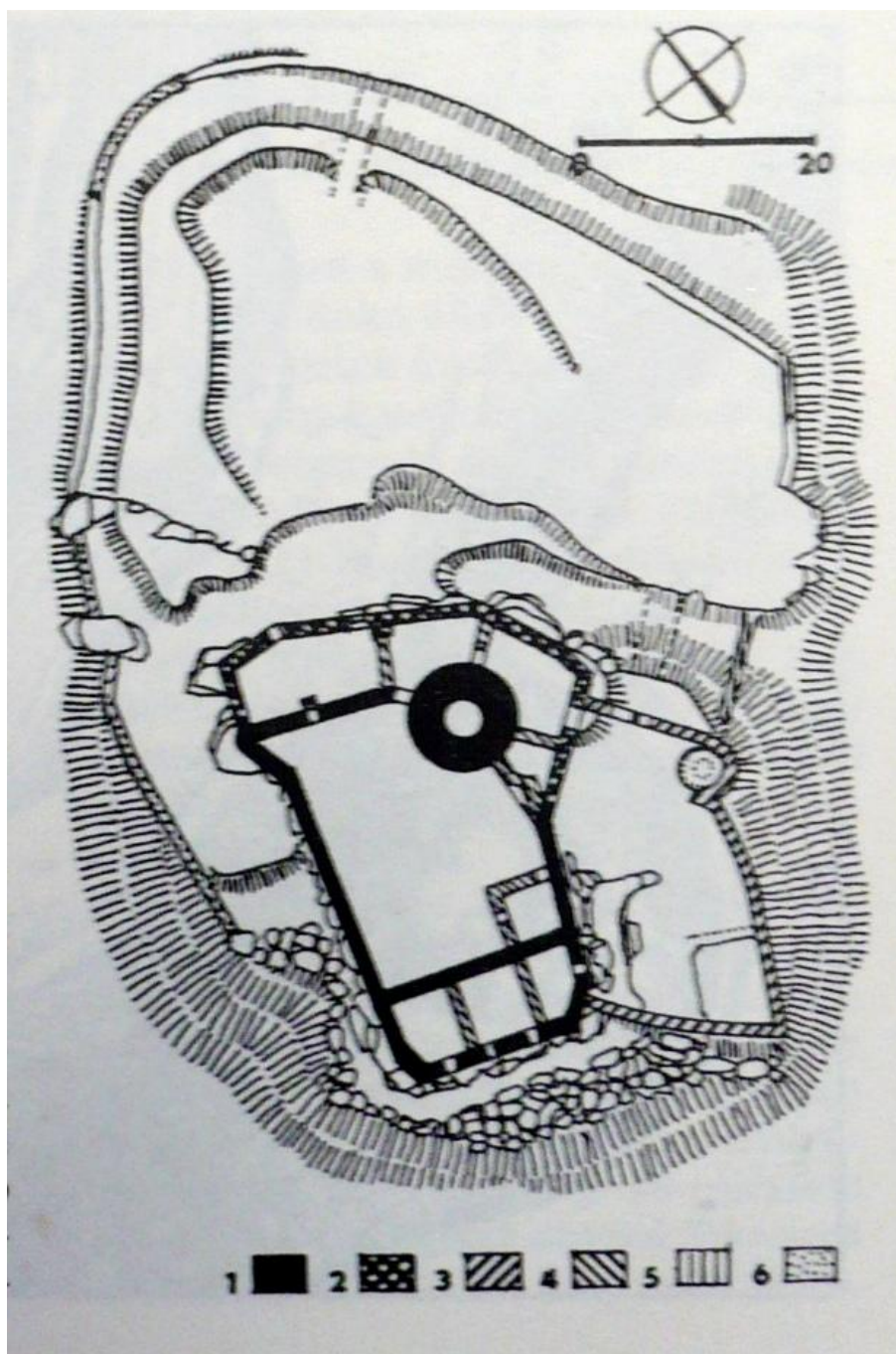
Obr. 4: Půdorys hradu Valdek podle J. Muka, upraven T. Durdíkem
