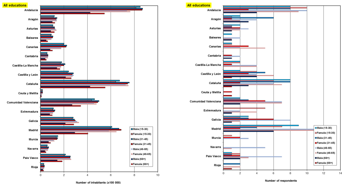
Obrázek 9. Dotazník 4: srovnání skutečné a dotazníkové populace
