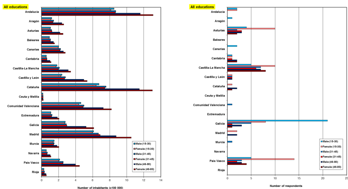
Obrázek 7. Dotazník 3: srovnání skutečné a dotazníkové populace
