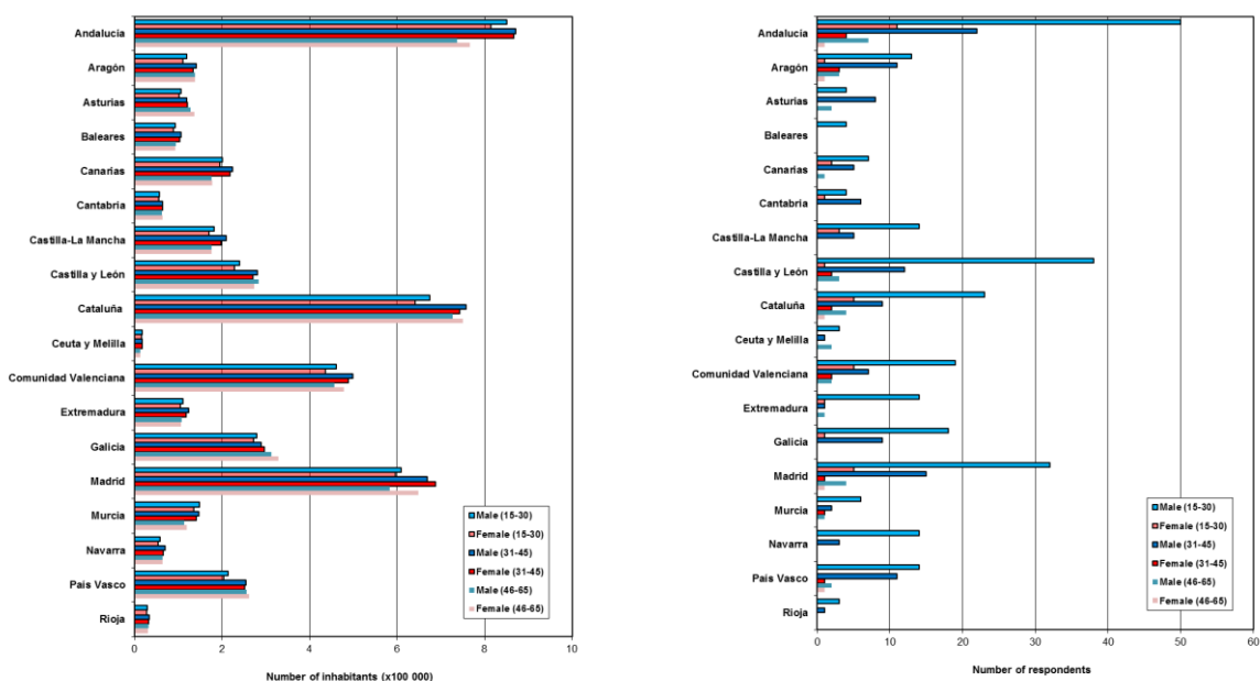
Obrázek 6. Dotazník 2: srovnání skutečné a dotazníkové populace
