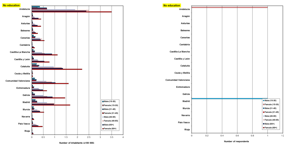
Obrázek 10. Dotazník 4: srovnání skutečné a dotazníkové populace podle vzdělání
