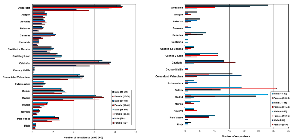
Obrázek 5. Dotazník 1: srovnání skutečné a dotazníkové populace
