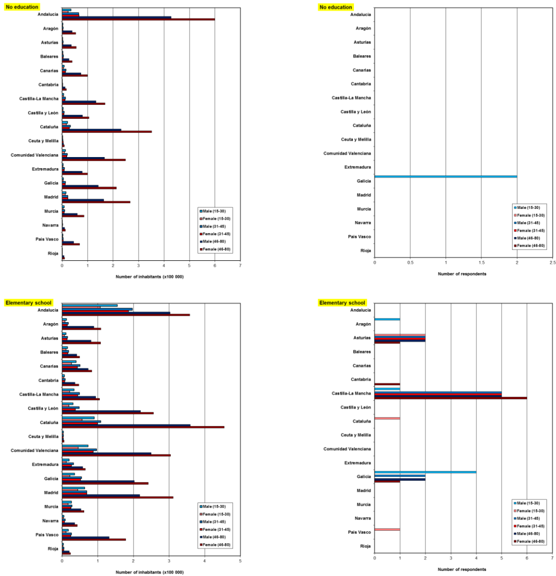
Obrázek 8. Dotazník 3: srovnání skutečné a dotazníkové populace podle vzdělání
