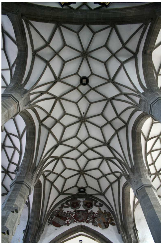
Prachatice, sv. Jakuba Větší – pohled na klenbu hlavní lodi a jižní lodi (vlevo), Průhled hlavní lodí na vítězný oblouk s malovanou datací 1500 (1490–1500)
