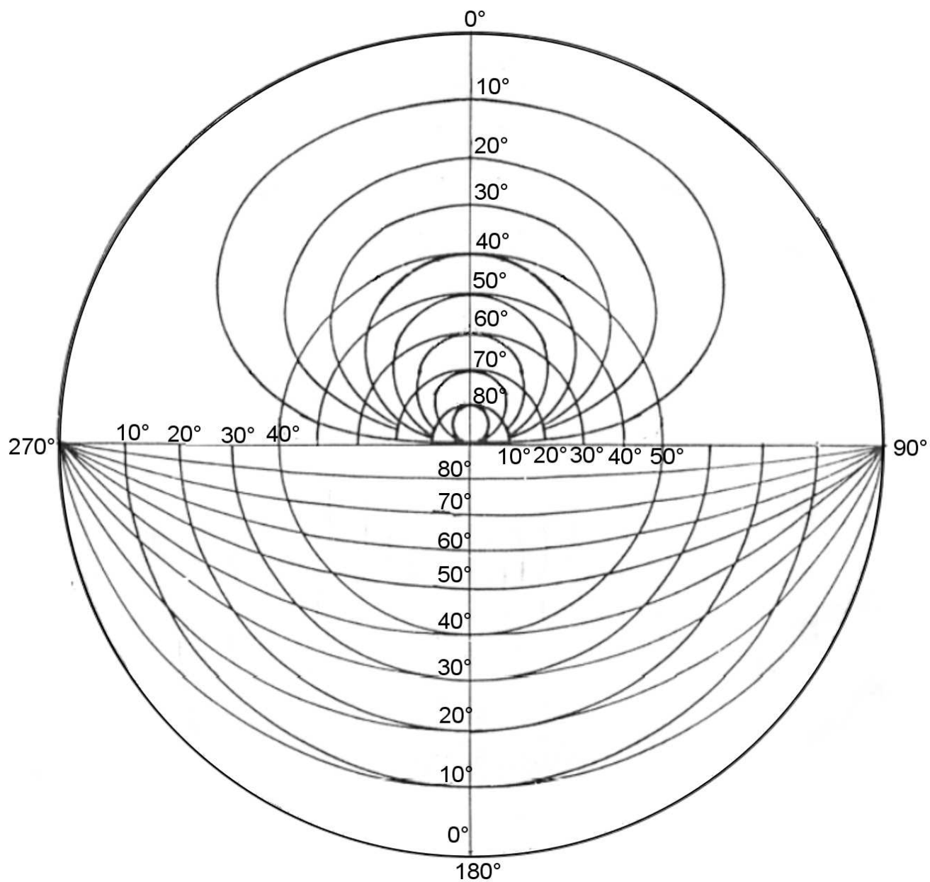
Příloha č. 3. Paletka pro rýsování křivek \lambda (upraveno podle Drozd, 1981)
