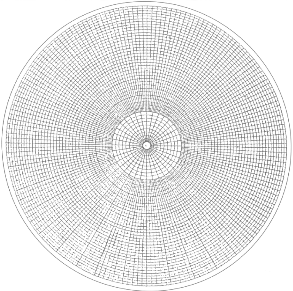
Příloha č. 4. Stereografická plochojevná Lambertova síť v pólové projekci (úprava Lisle, Leyshon, 2004)
