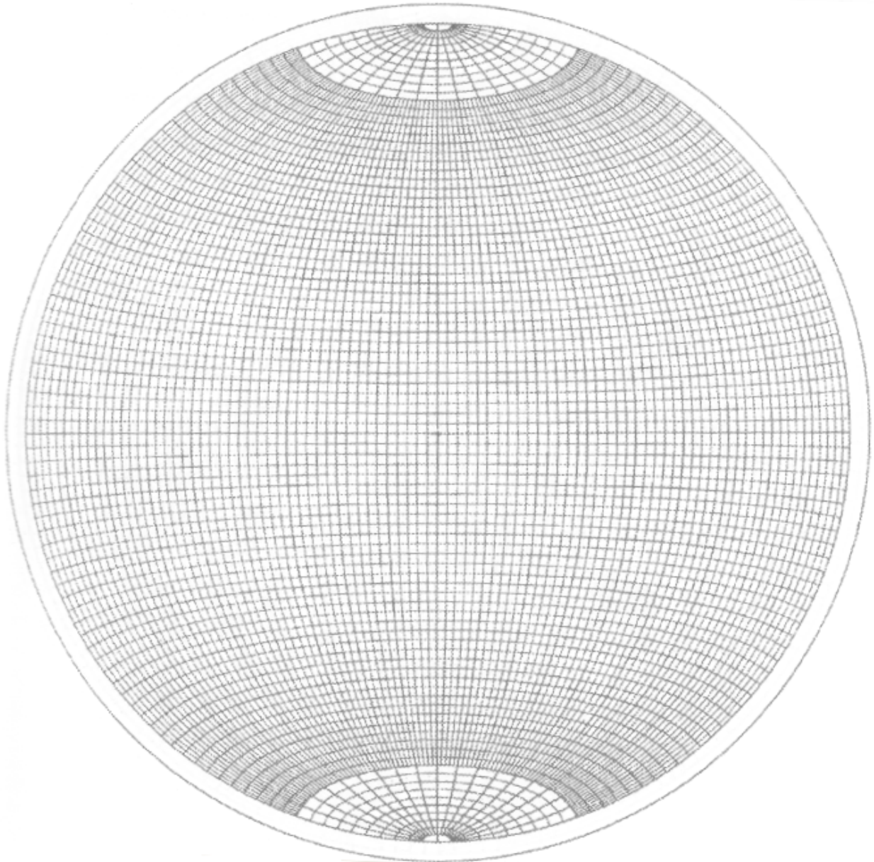
Příloha č. 5. Stereografická plochojevná Lambertova síť v rovníkové projekci (úprava Lisle, Leyshon, 2004)
