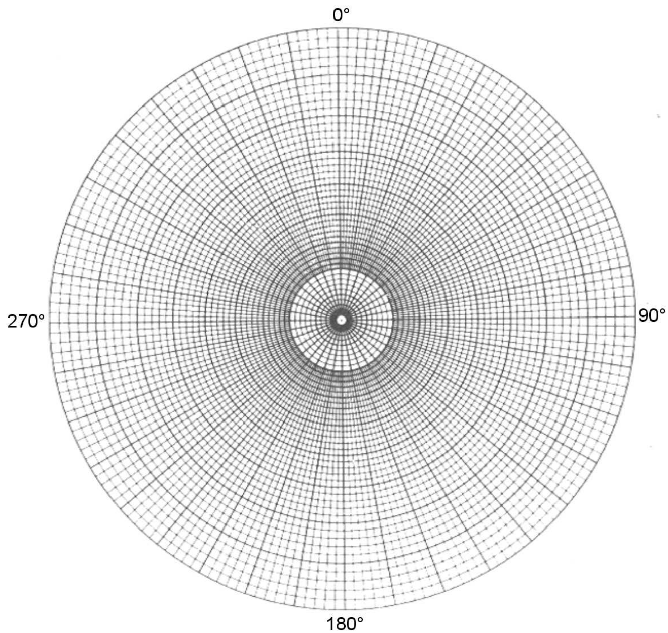
Příloha č. 1. Stereografická úhlojevná Wulfova síť v pólové projekci
