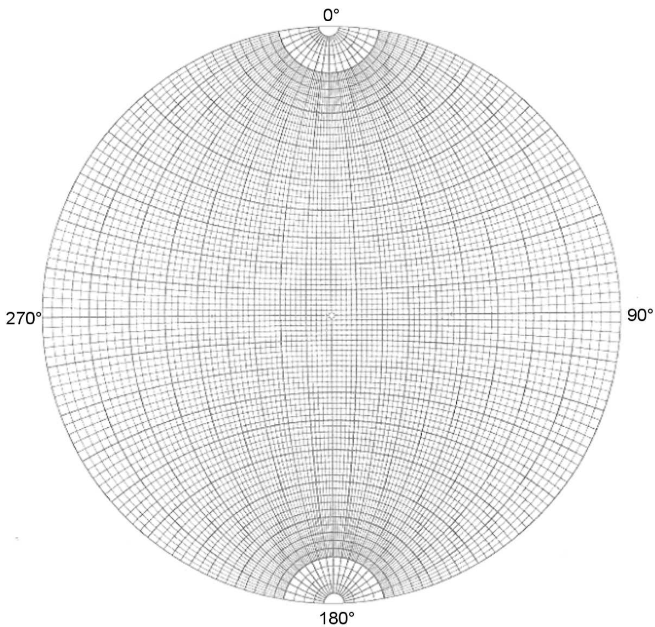
Příloha č. 2. Stereografická úhlojevná Wulfova síť v rovníkové projekci
