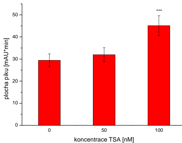
Obrázek 34 Vliv TSA na oxidaci ellipticinu hovězí laktoperoxidásou. Složení inkubační směsi: 10 \mu M ellipticin; 10 \mu g/ml laktoperoxidasa; 0,50 nebo 100 nM TSA; 100 \mu M H_2O_2 ; 0,1 M KH_2PO_4 pufr pH 7,4. Hodnoty jsou průměrem tří nezávislých měření, *** p < 0,01 . Studentův t-test.
