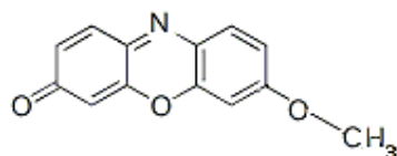
Obrázek 18 Struktura 7-methoxyresorufinu.
