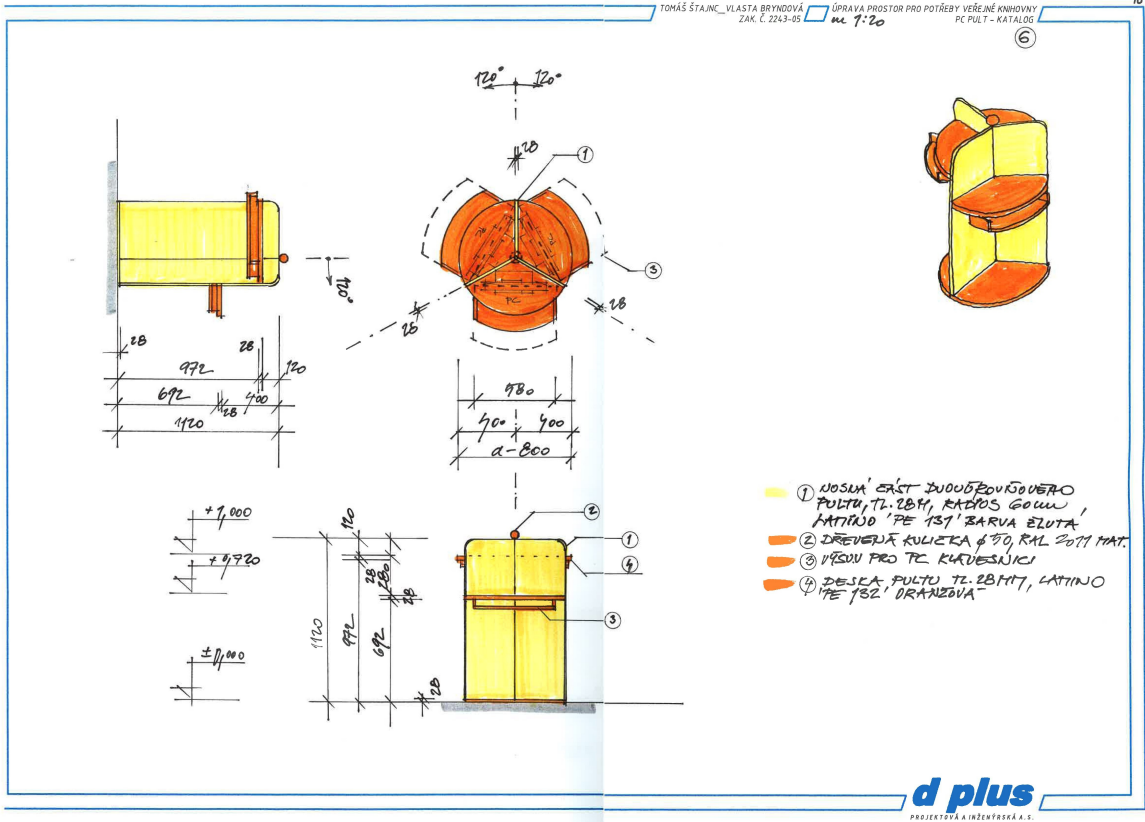
Obrázek číslo 18 – Návrh pultu pro OPAC (archiv Knihovny na Vinohradech)
