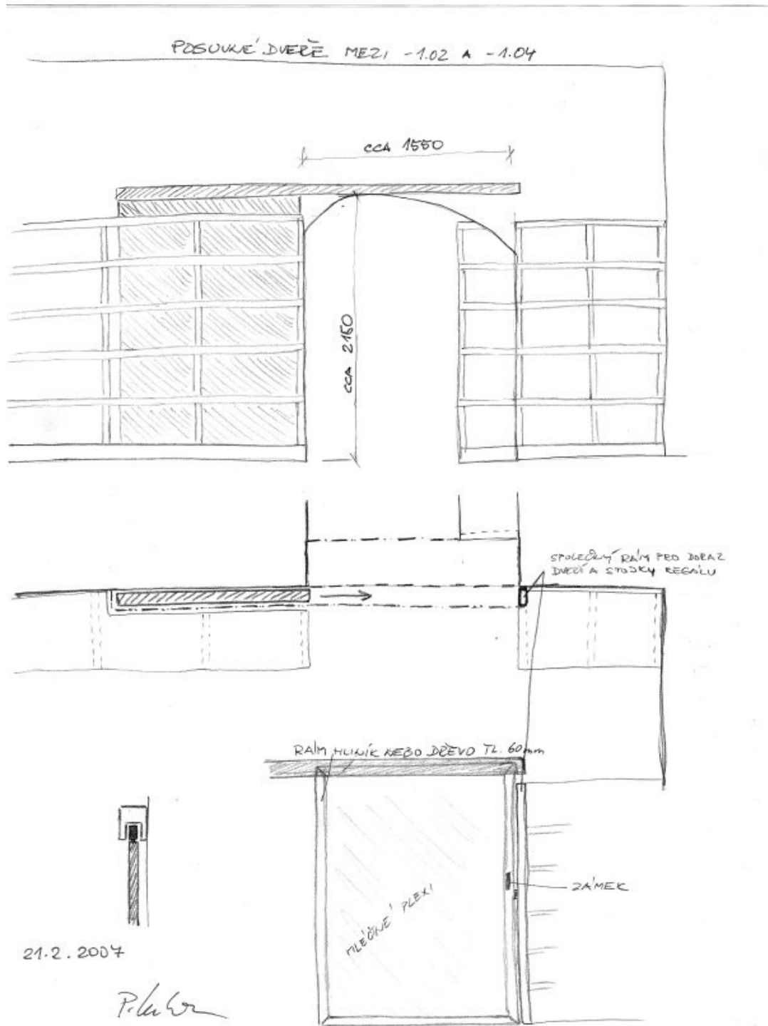
Obrázek číslo 15 – Návrh posuvné dveře (archiv Knihovny na Vinohradech)
