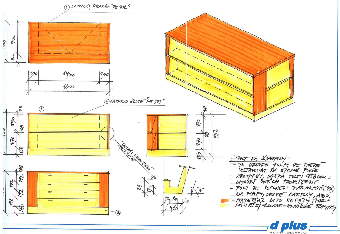
Obrázek číslo 16 – Návrh pultu na časopisy (archiv Knihovny na Vinohradech)
