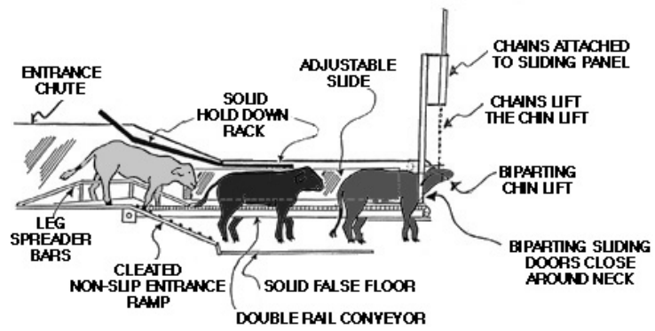
Obrázek 4: Princip klece na malý dobytek
