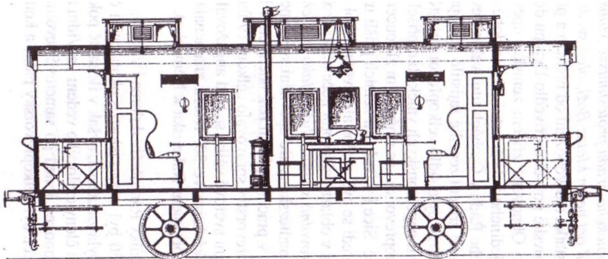
A – vůz velitele vlaku
