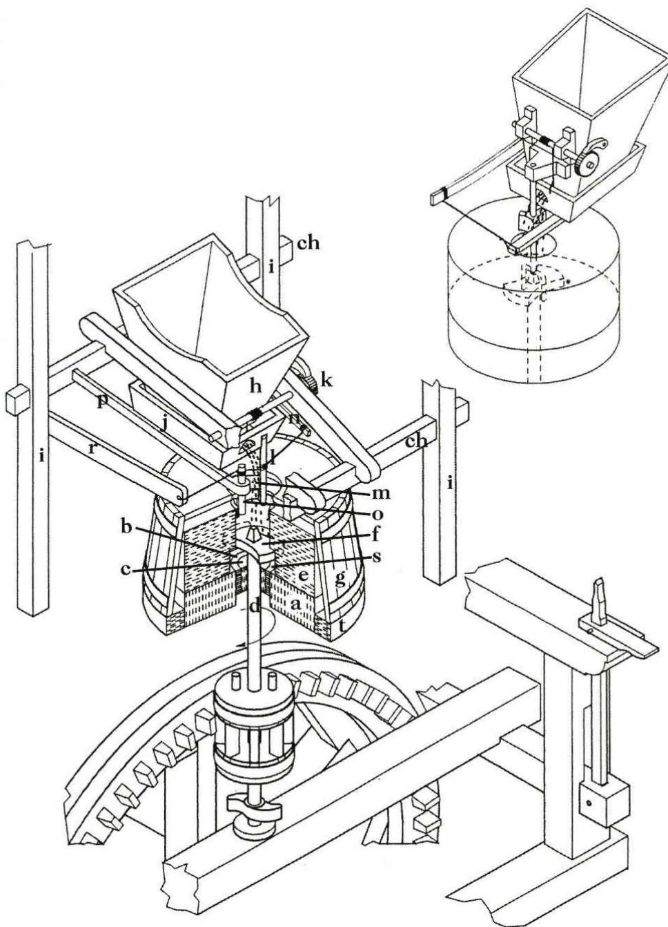
Obrázek 16: Mlecí ústrojí
