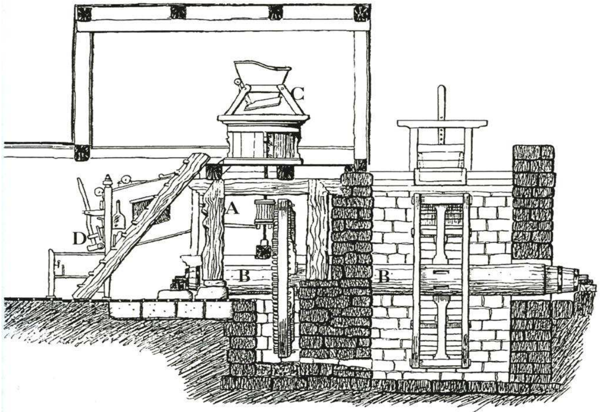
Obrázek 14: Části staročeského mlýna
