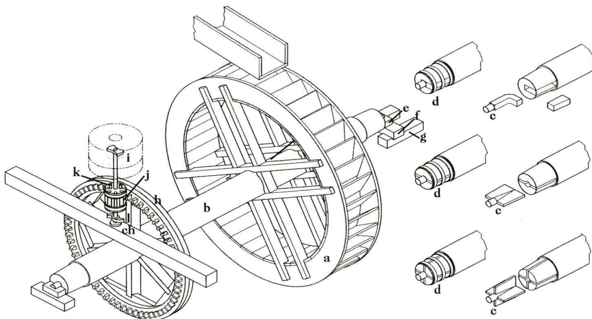
Obrázek 15: Pohony a převody mlýnského složení
