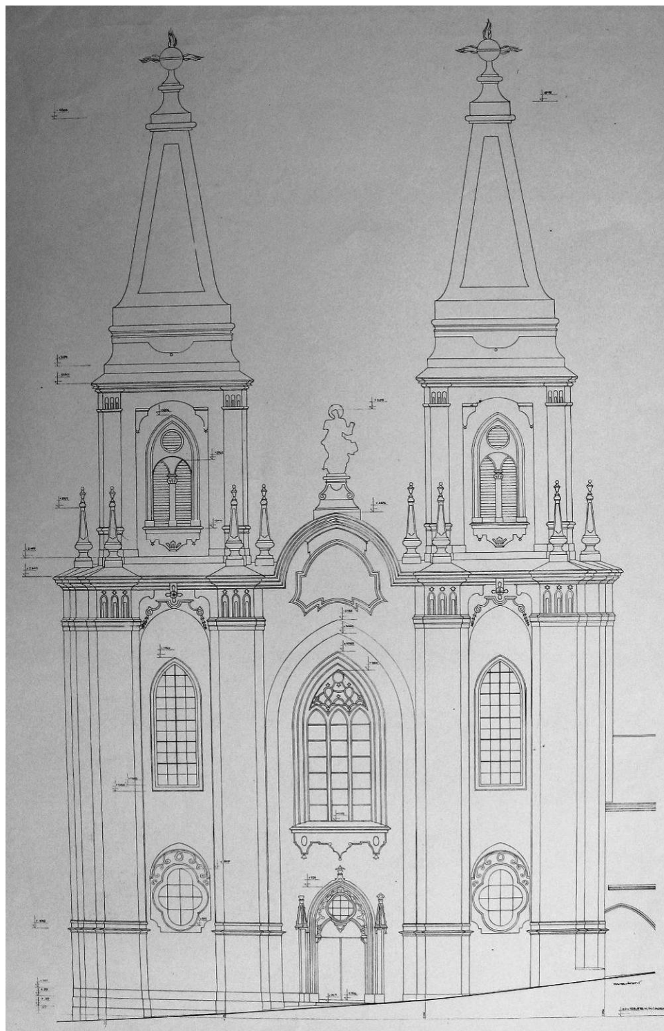
Výkres č. 1. Pohled na západní průčelí kostela
