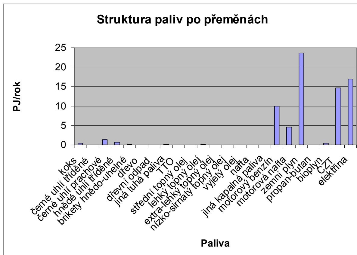
Graf 9 Struktura paliv po přeměnách, Praha, 2001
