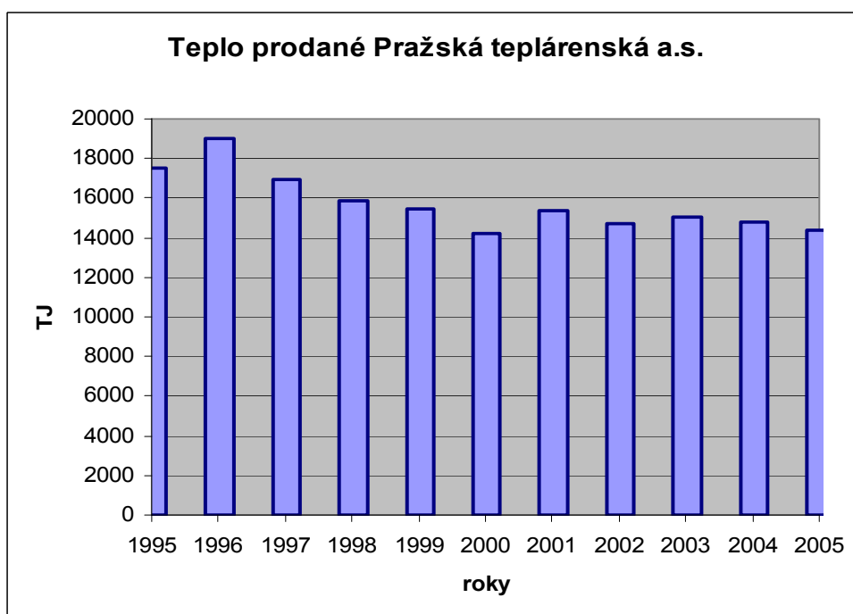
Graf 18 Teplu prodané Pražská plynárenská a.s., Praha Zdroj: Ročenka životního prostředí, 2007
