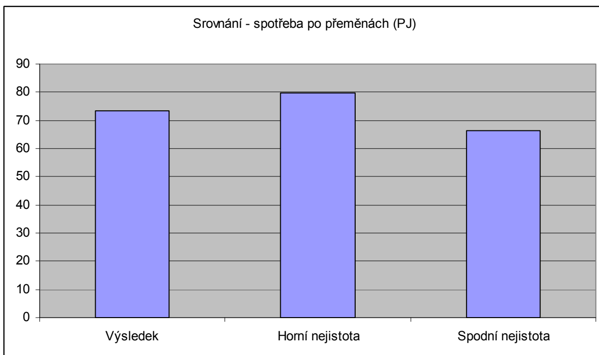
Graf 28 Nejistoty srovnání - spotřeba po přeměnách, Praha, 2001
