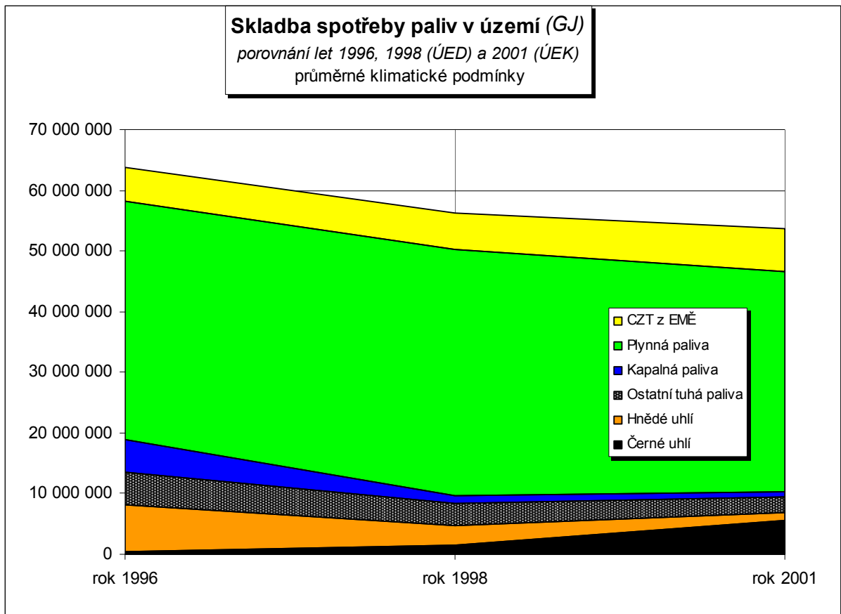
Graf 8 Skladba spotřeby paliv v území, Praha
